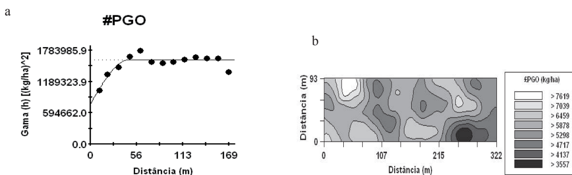
Figura 3. Semivariograma e Mapa de krigagem da produtividade de grãos de arroz ( \text{EPGO} ) em um Latossolo Vermelho distroférico sob plantio direto. Números entre parênteses são, respectivamente, valor do efeito pepita ( C_0 ), contribuição ( C_1 ) e alcance (a). Selvíria – MS, 2009/2010.
