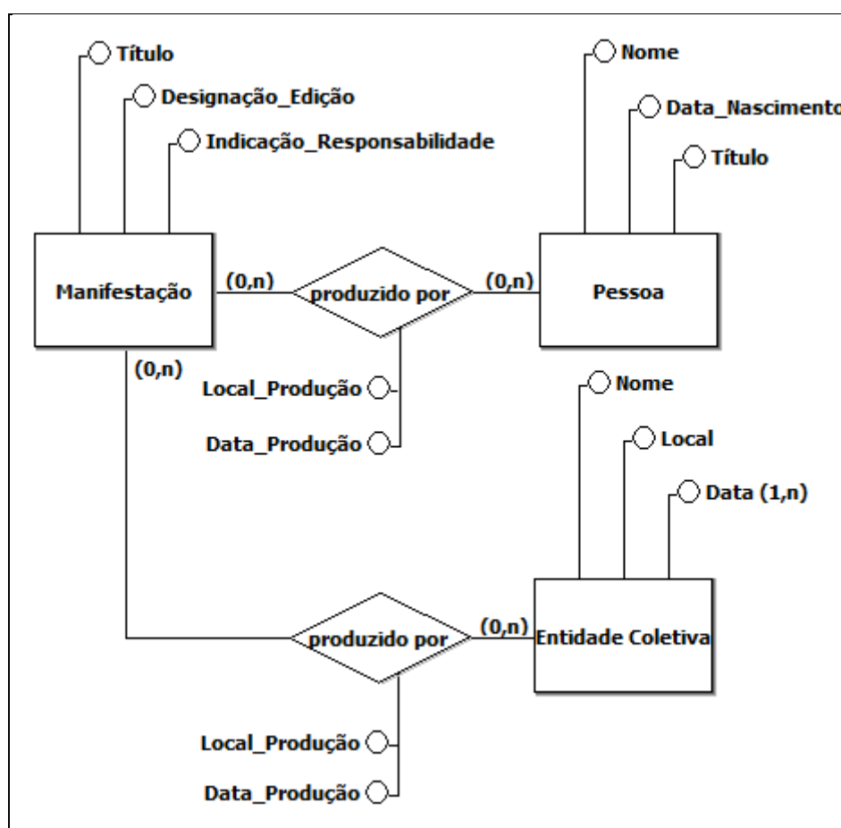
Figura 27 - Diagrama Entidade-Relacionamento
