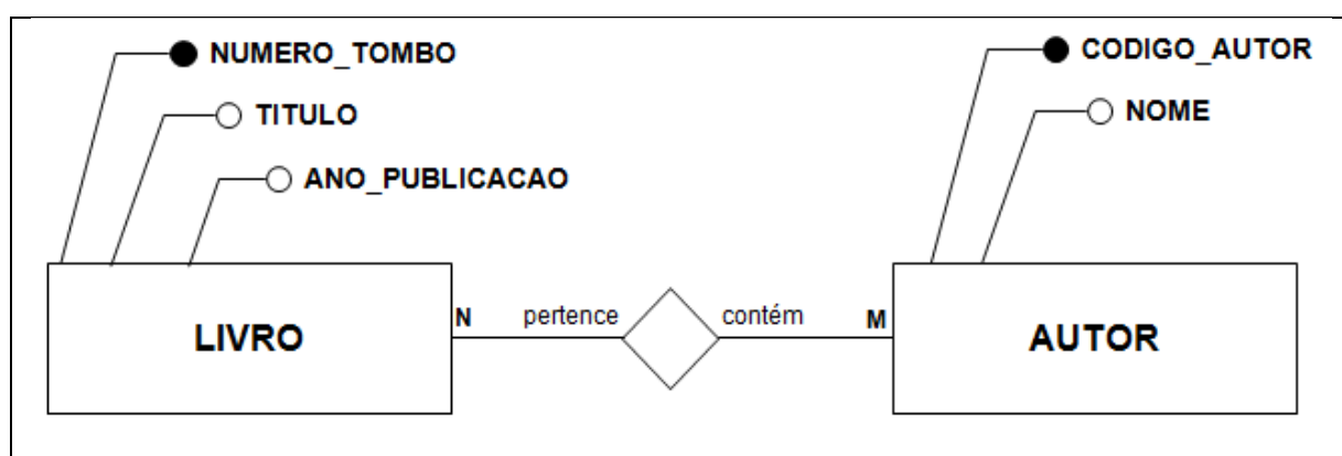
Figura 13 – Diagrama Entidade-Relacionamento
