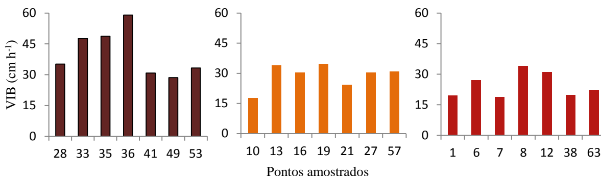
Figura 15. Velocidade de infiltração básica de água no solo (VIB), obtida por metodologia de anéis concêntricos, amostrados em 21 pontos no Perímetro de Irrigação Pontal Sul.
