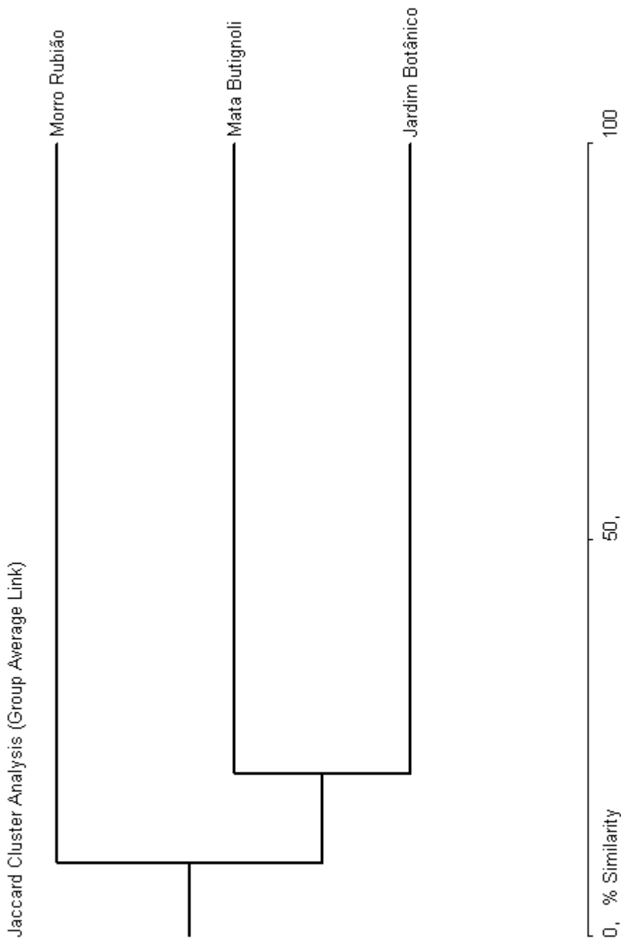
Figura 25: Dendrograma de similaridade florística entre os fragmentos de Floresta Estacional Semidecidual estudados, Botucatu, SP.
