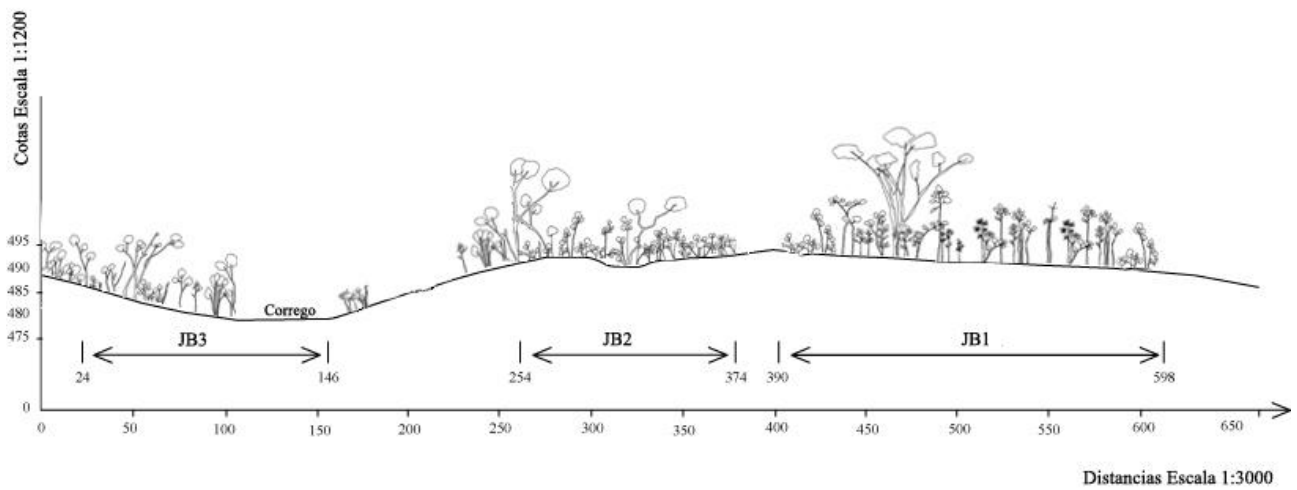
Figura 10: Diagrama de perfil representando a distribuição de três fragmentos de vegetação nativa no Jardim Botânico do Instituto de Biociências-UNESP, localizado no distrito de Rubião Júnior, Botucatu, SP. Exagero vertical do perfil: 2,5. vezes. Valores de distâncias e cotas em metros.
