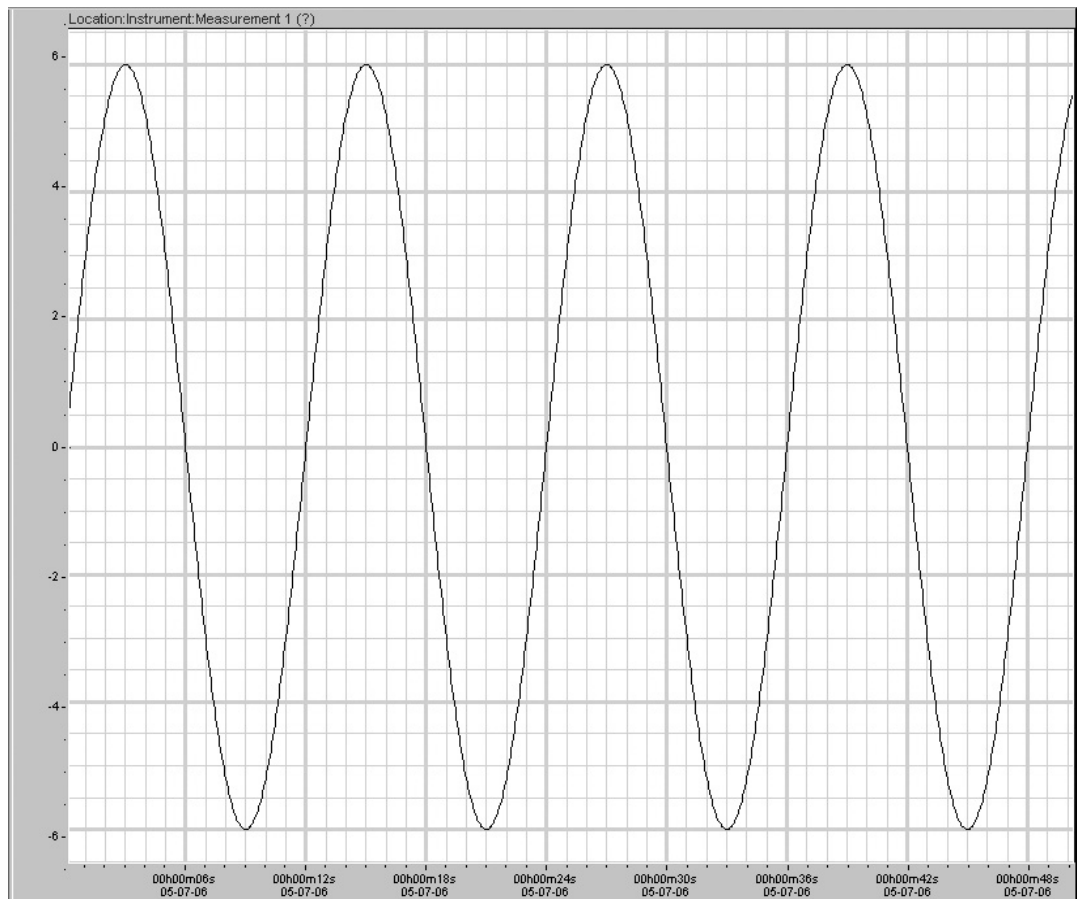
Figura 3.8 – Gráfico da função (3.12)
