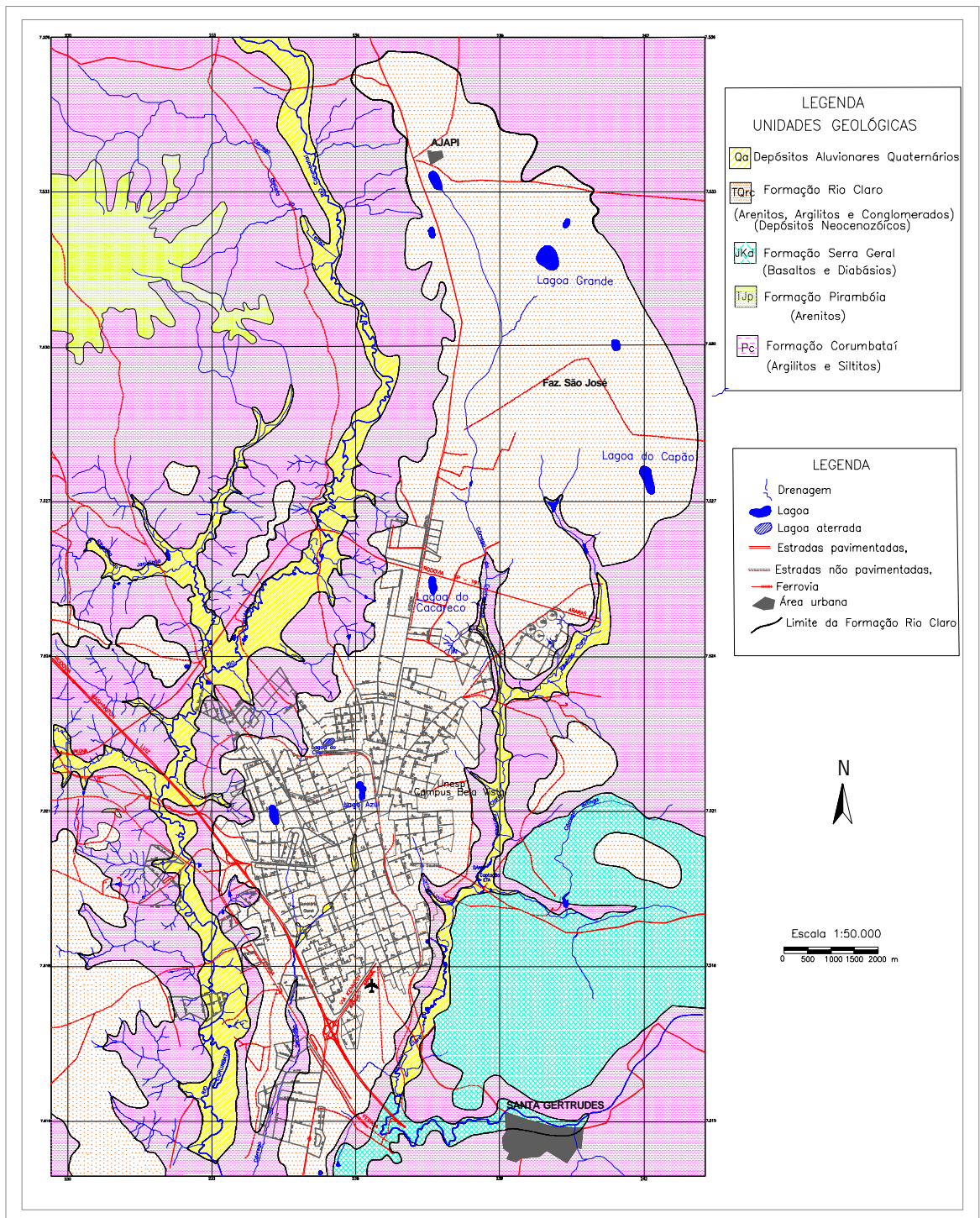
Figura 2.1 – Mapa geológico do Município de Rio Claro (OLIVA, 2002).
