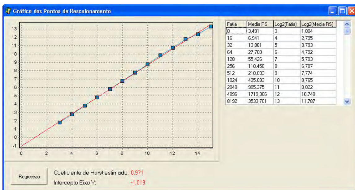
Figura 6.11 – Gráfico dos pontos da Tabela 5.1 (em azul), juntamente com a reta ajustada (em vermelho) da análise R/S para os dados de variação de coluna d’água.
