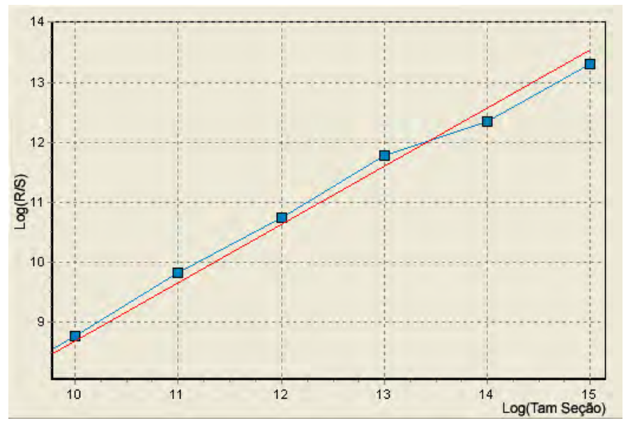
Figura 6.14 – O mesmo tipo de quebra da Figura 6.13, porém mais sutil, no gráfico da série temporal de coluna d'água, em t = \log_2 8192 horas = 341 dias
