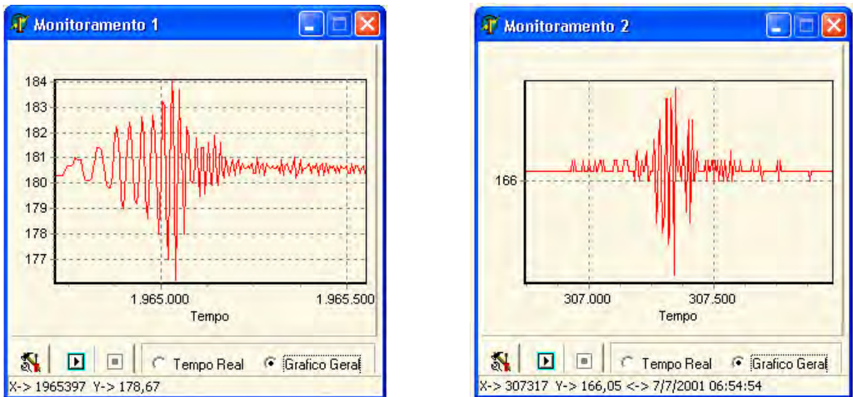
Figura 5.8 – Oscilação devido ao terremoto no dia 23 de Junho de 2001 – Peru (à esquerda), e seu aftershock (à direita), em 7 de Julho. (Tempo em segundos e Coluna em cm)
