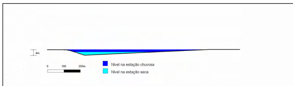
Figura 29: Perfil esquemático da Lagoa do Vânico, demonstrando a variação sazonal do lençol freático. Exagero vertical 10 vezes. Elaborado por Rubens Hardt.
