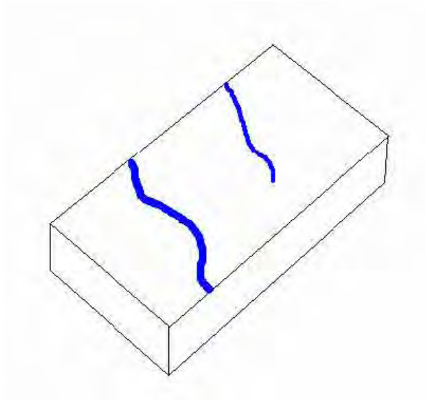
Figura 48: Inicialmente, a área era plana, com a drenagem seguindo antigos planos de falha.
