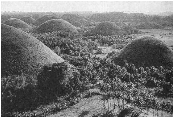
Figura 6: Carste em torre (Filipinas) segundo Ford & Williams (1989), foto de R. Wasson.
