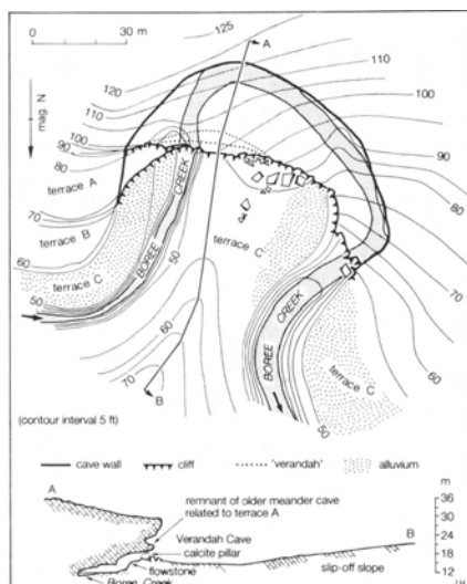
Figura 10: Caverna meândrica em Boree Creek, Borenore, NSW, segundo JENNINGS (1985 - pag. 93).
