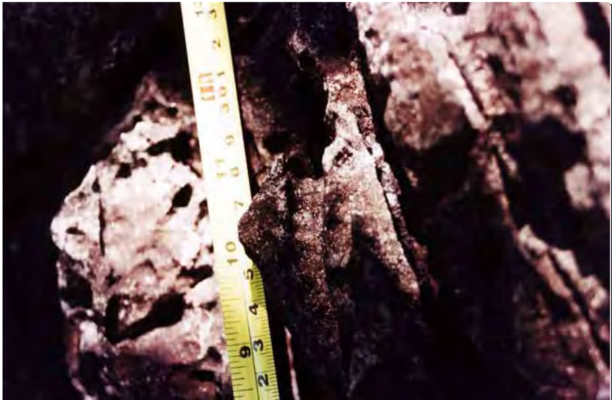
Figura 46: Karrens observados na porção média da Serra do Calcário. À direita, rillenkarren, canais de dissolução devido ao fluxo gravitacional da água sobre a superfície da rocha. (Foto: Rubens Hardt)
