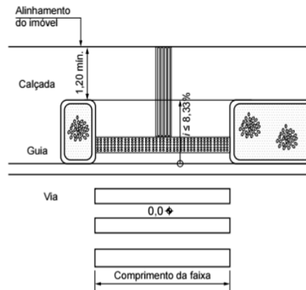
Figura 60 - Rebaixamentos de calçada entre canteiros (em metros)
