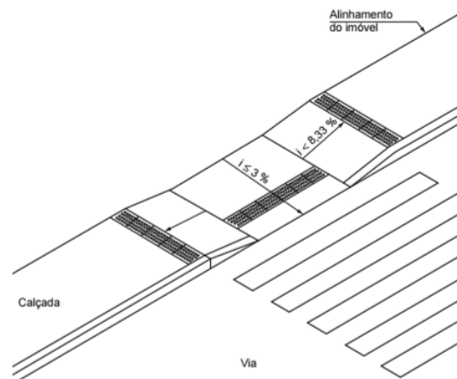
Figura 61 - Rebaixamentos de calçadas estreitas
