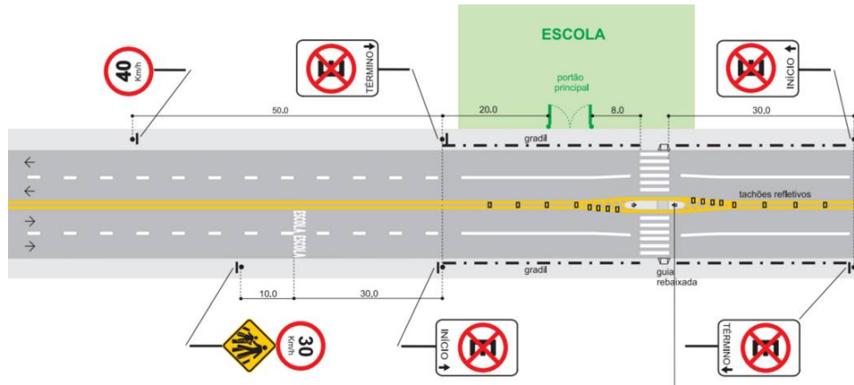
Figura 67 - Modelo de projeto para sinalização e segurança e áreas escolares para vias com pista simples e sentido duplo de circulação
