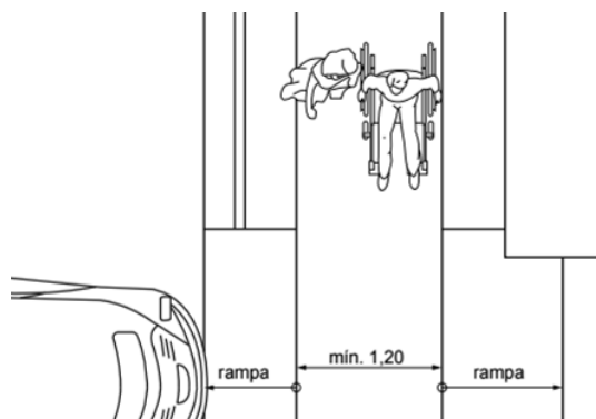
Figura 54 - Acesso de veículos aos lotes, desenhos na calçada (em metros)
