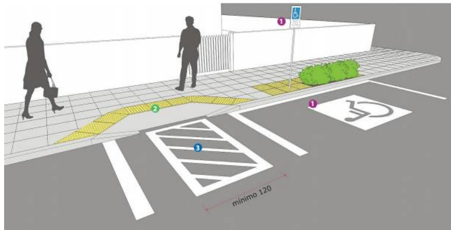
Figura 62 – Estacionamento para pessoa com deficiência física motora
