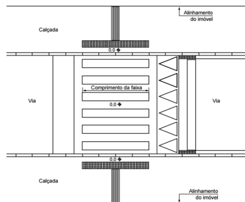
Figura 57 - Faixa elevada de travessia (em metros)
