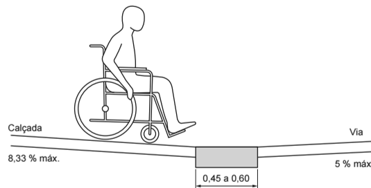
Figura 59 - Faixa de acomodação para travessia de pedestres (em metros)
