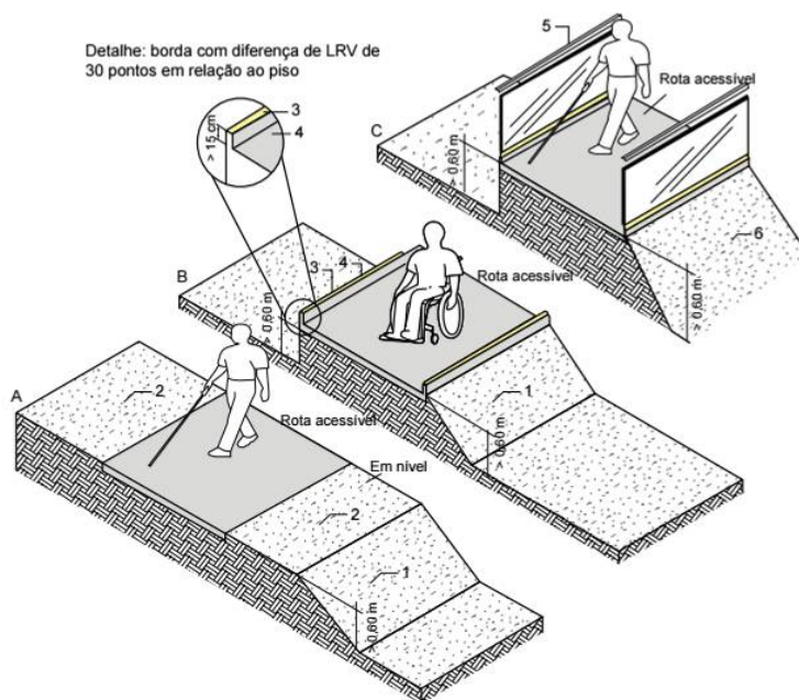
Figura 64 - Exemplos de proteção contra quedas em rotas acessíveis (em metros)
