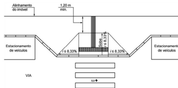
Figura 56 - Redução do percurso de travessia (em metros)
