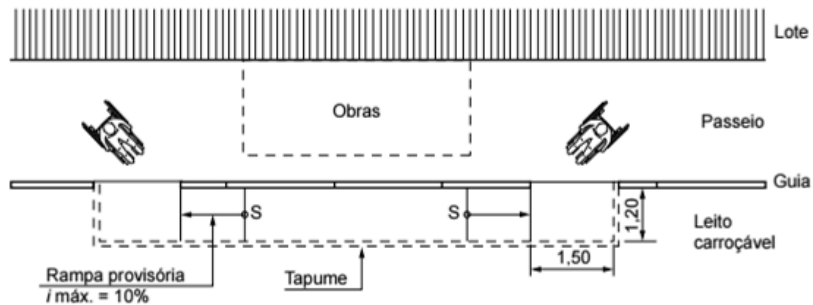
Figura 55 - Rampas de acesso provisórias (em metros)
