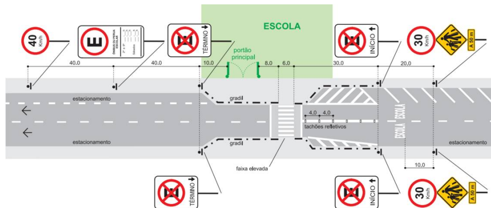
Figura 66 - Modelo de projeto para sinalização e segurança e áreas escolares para vias com pista simples e sentido único de circulação
