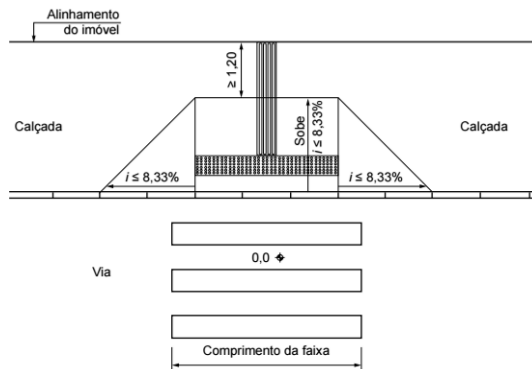
Figura 58 - Rebaixamento de calçadas (em metros)
