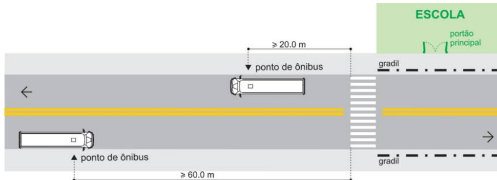
Figura 71 - Localização de pontos de parada de ônibus próximo à escola
