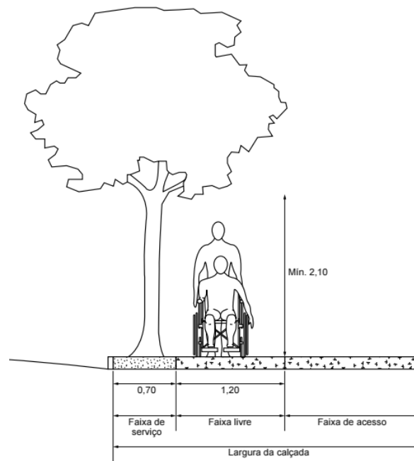
Figura 53 - Faixas de uso das calçadas (em metros)
