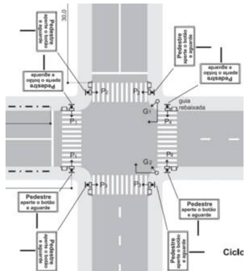
Figura 68 - Localização de semáforos de pedestres nas travessias
