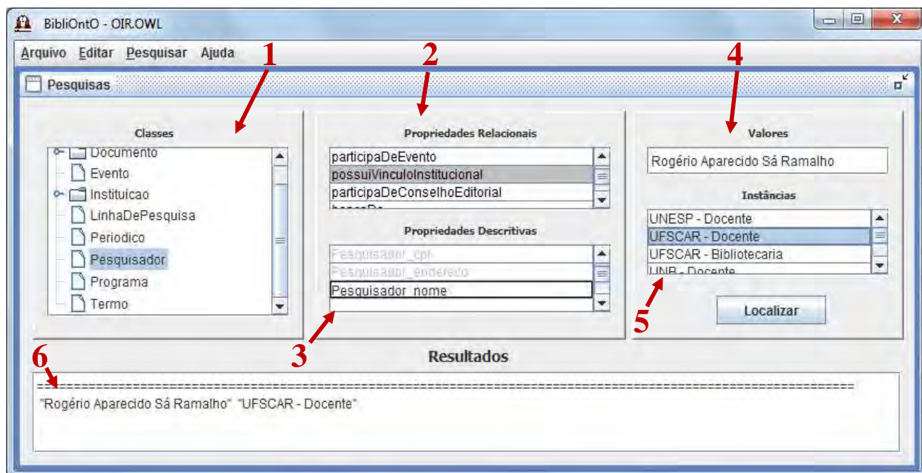
FIGURA 22 – Interface de Busca do BibliOntO
