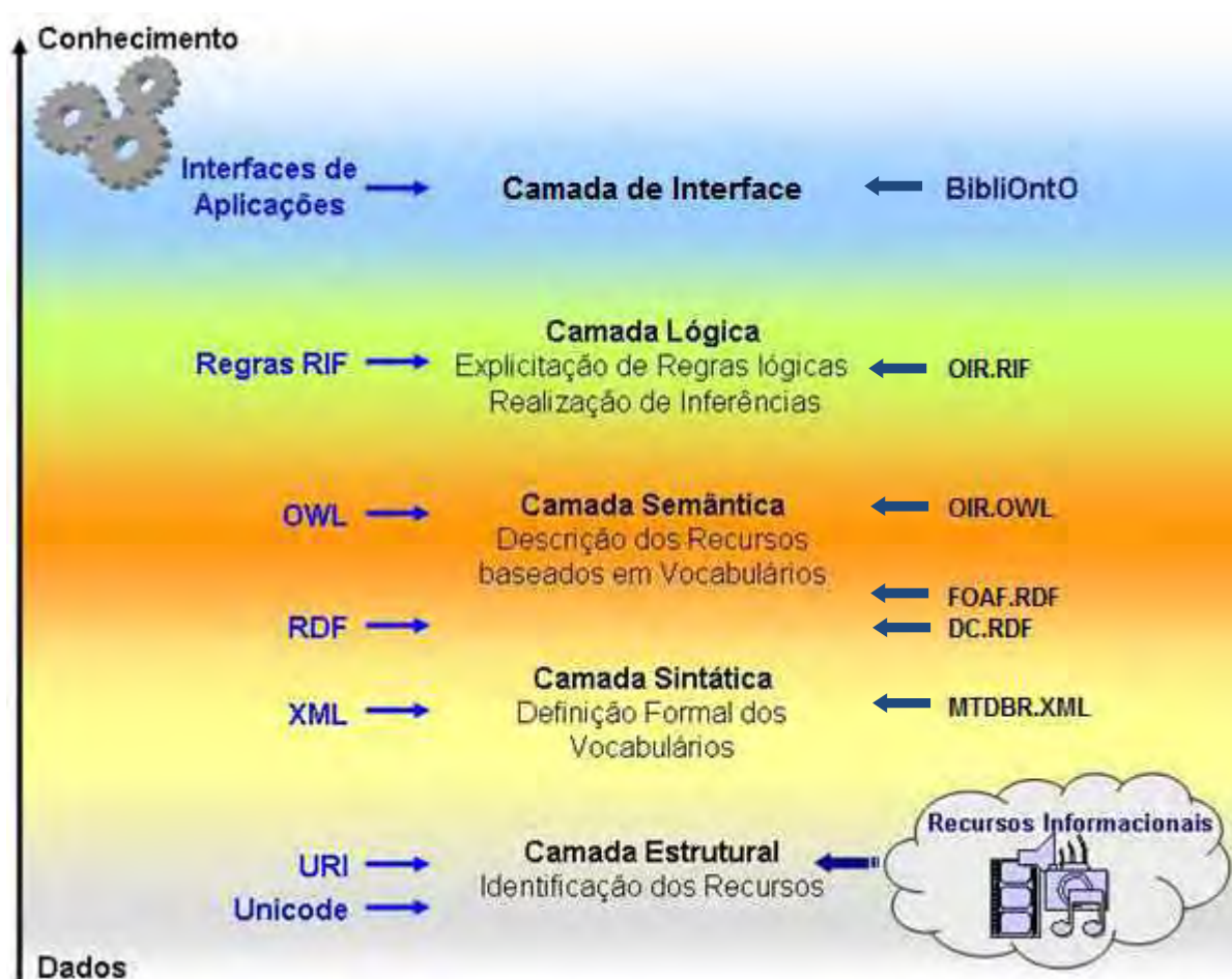
FIGURA 21 – Tecnologias e Camadas da Web Semântica
