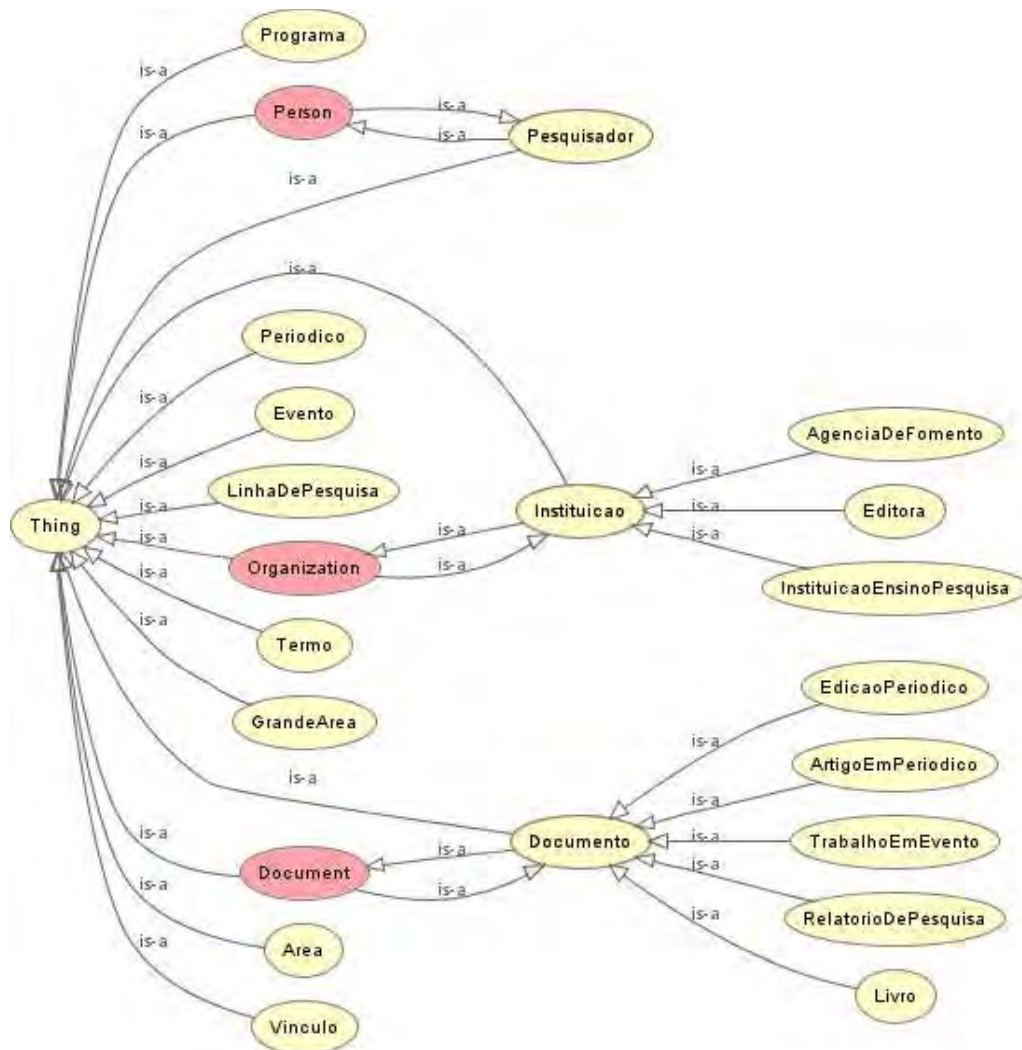
FIGURA 19 – Hierarquia de Classes da OIR
