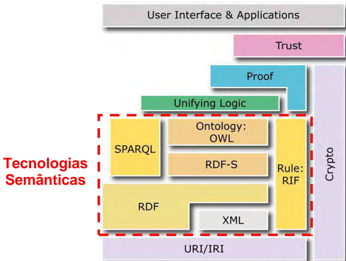
FIGURA 11 – Arquitetura da Web Semântica e Tecnologias Semânticas FONTE: Adaptado de Bratt (2008, p. 22)
