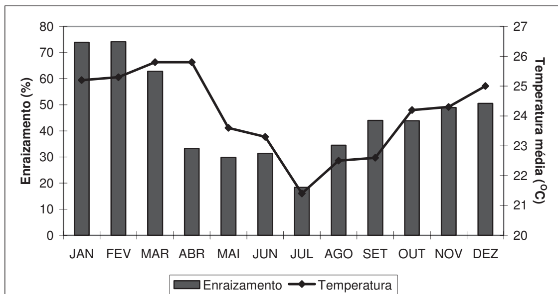
Figura 1 – Percentagem de enraizamento de estacas de cacaueteiro e temperatura média dos meses de coleta de estacas.
