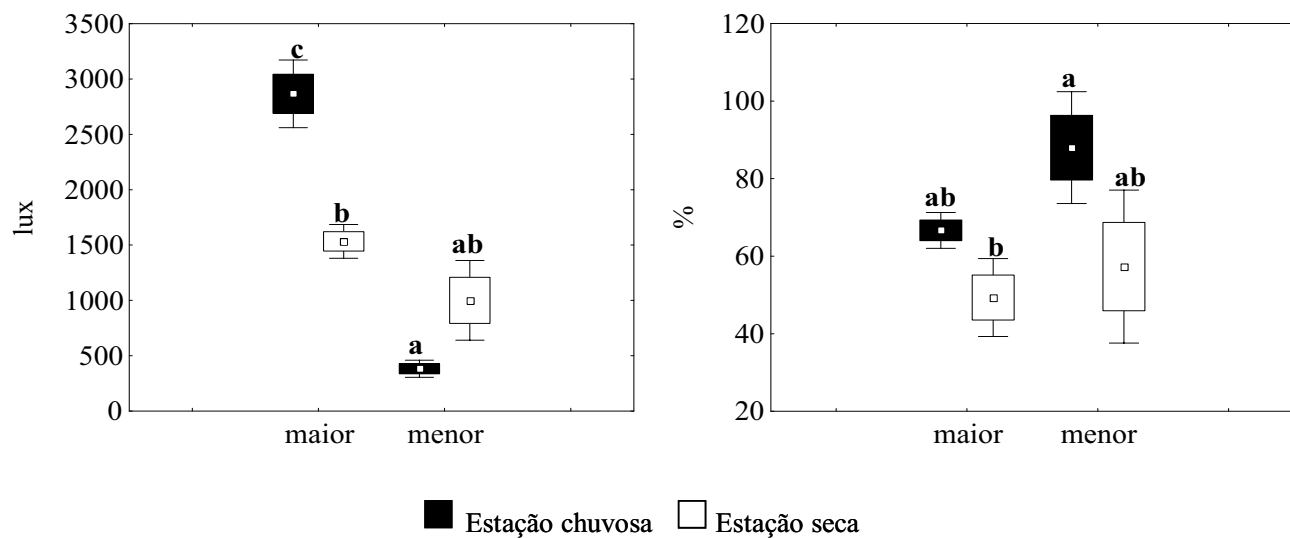
Figura 7. Luminosidade (Lux) e percentual de cobertura vegetal (%) mensuradas nos riachos de maior e menor porte da Bacia do Rio Paranapanema, durante as estações chuvosa (janeiro e fevereiro/2007) e seca (julho e agosto/2007). As letras minúsculas indicam os resultados do Teste de Tukey.
