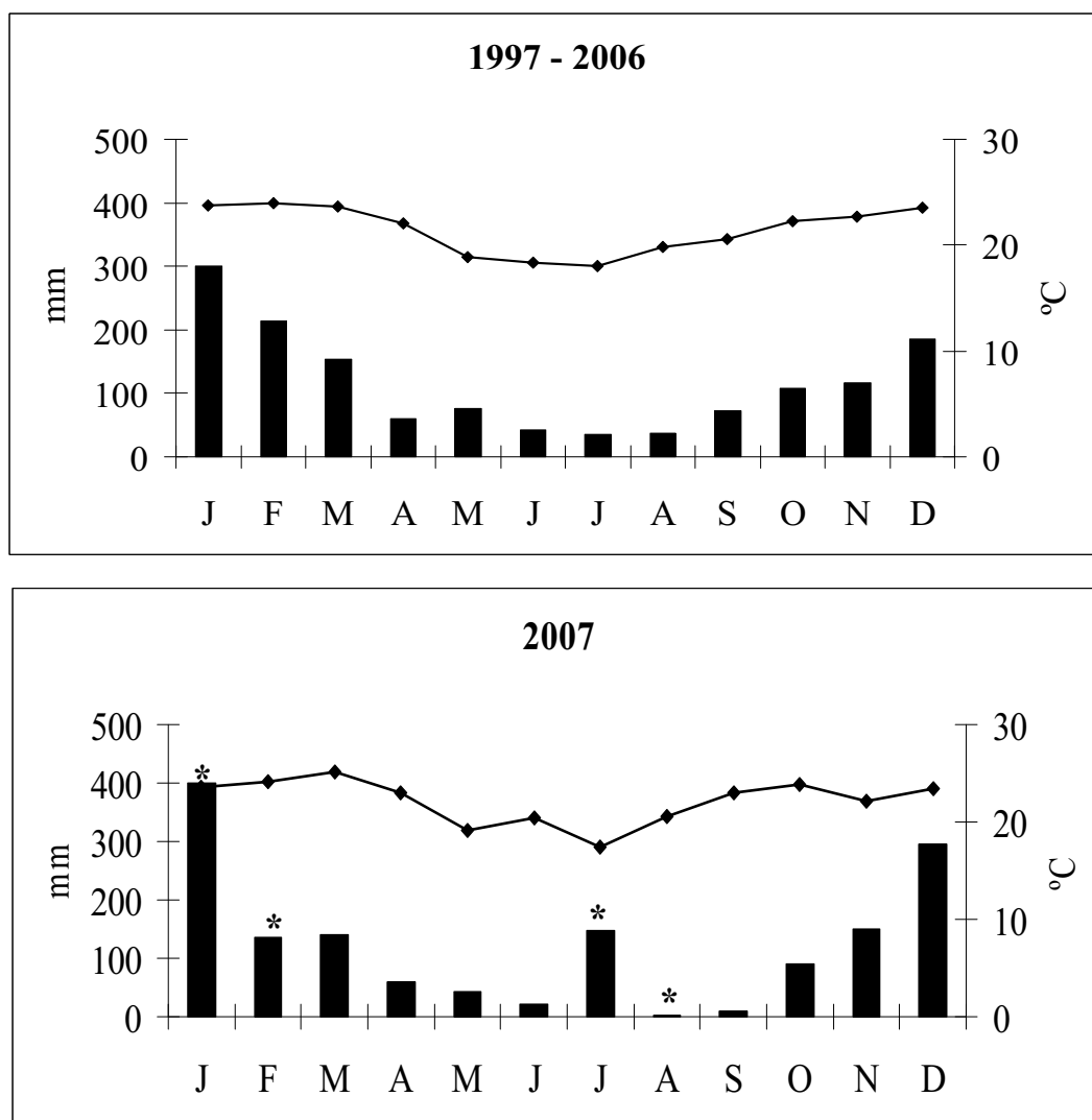
Figura 4. Pluviosidade mensal total (barras; mm) e temperatura média mensal (°C) referente à média de 10 anos (1997-2006) e ao ano de 2007 (* meses de coleta de dados). Fonte: CIIAGRO ( www.ciiagro.sp.gov.br ; estação de Botucatu).
