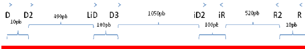
FIGURA 8A: representação do gene F-reticulon 4, com a região de anelamento dos primers que foram utilizados para amplificação e posterior seqüenciamento desse gene. (Primers Diretos: D,D2,LiD, D3 e iD2; Primers Reversos: iR, R2 e R).
