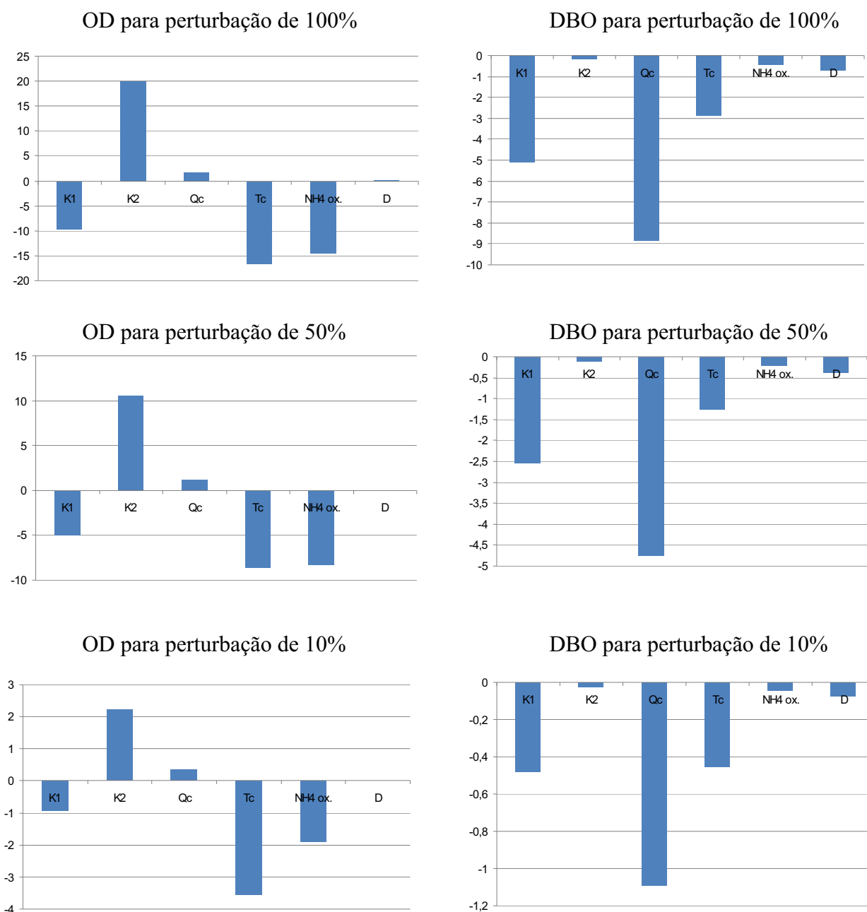
Figura 8: Valores médios da porcentagem da diferença causada pelas diferentes perturbações.
