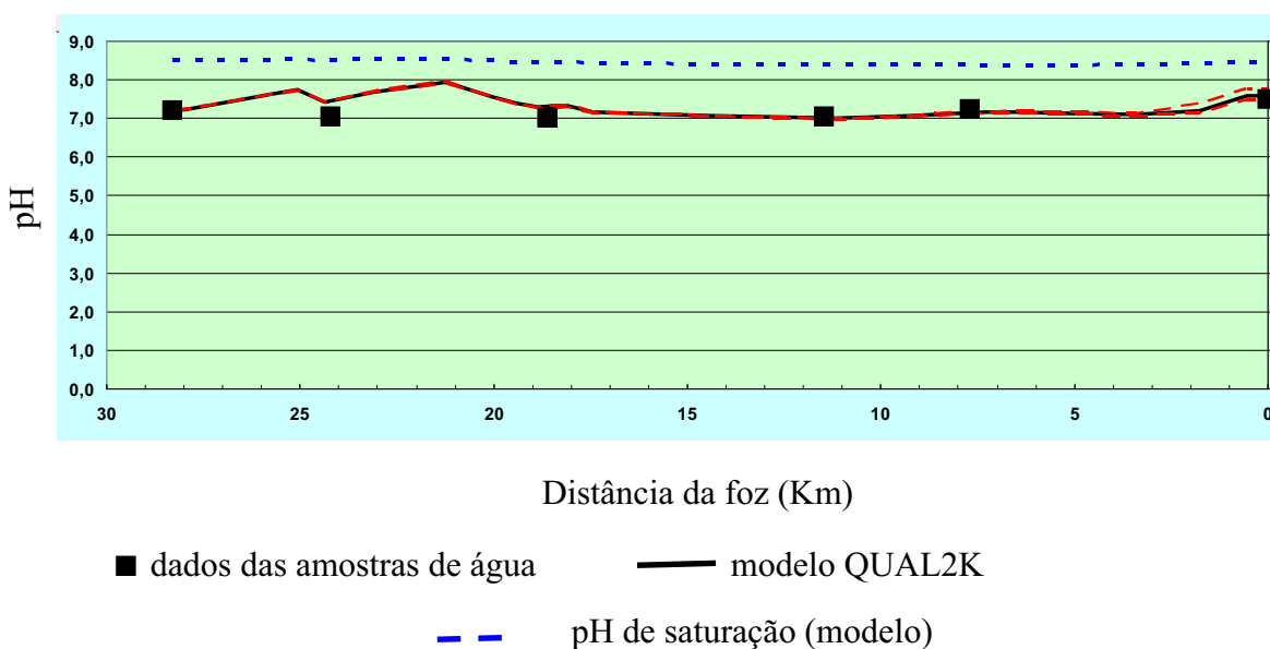
Figura 19: Comportamento do pH no segmento simulado do ribeirão Claro.
