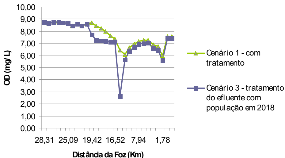
Figura 30: Comportamento da variável OD nos cenários 1 e 3.
