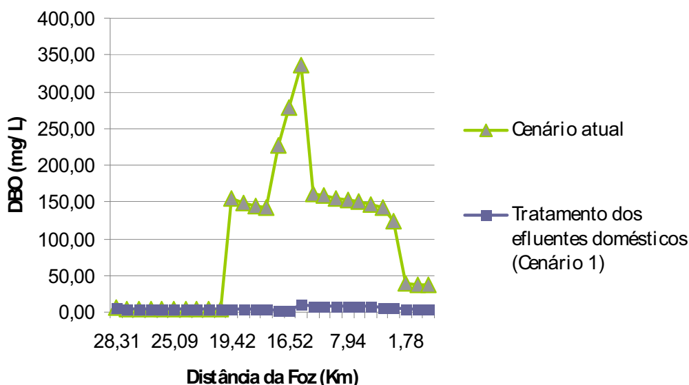
Figura 23: Gráfico do comportamento da DBO no cenário atual e no cenário considerando tratamento de 100% do efluente lançado (cenário 1).
