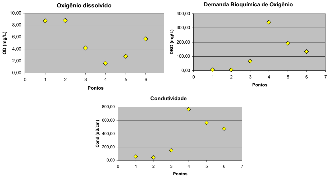
Figura 7: Comportamento de OD, DBO e condutividade.
