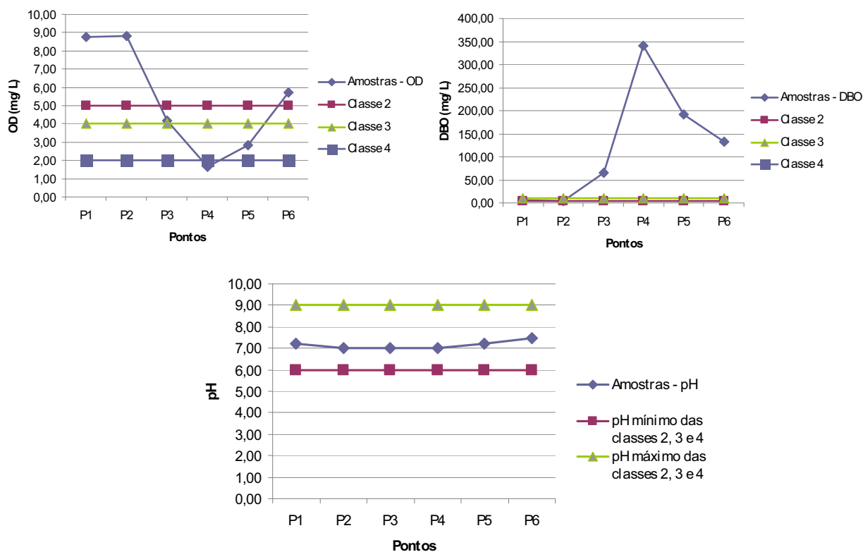
Figura 20: Comparação das variáveis de qualidade das amostras de água com os limites impostos pela Resolução CONAMA 357/05 para as diferentes classes
