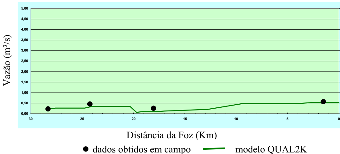
Figura 13: Comportamento da vazão no segmento simulado do ribeirão Claro.
