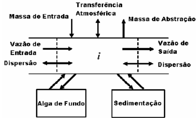
Figura 5: Balanço de massa (GONÇALVES & DIBIAZI, 2006).
