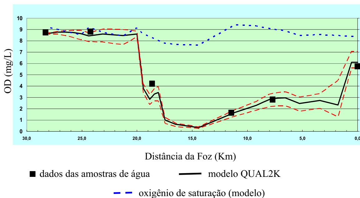
Figura 9: Ajuste do modelo QUAL2K ao ribeirão Claro para a variável OD.
