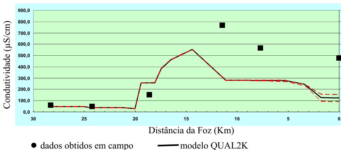
Figura 16: Comportamento da condutividade elétrica no segmento simulado do ribeirão Claro.
