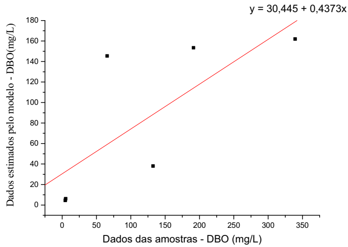
Figura 12: Regressão linear para os dados de DBO das amostras e aqueles estimados pelo modelo QUAL2K.
