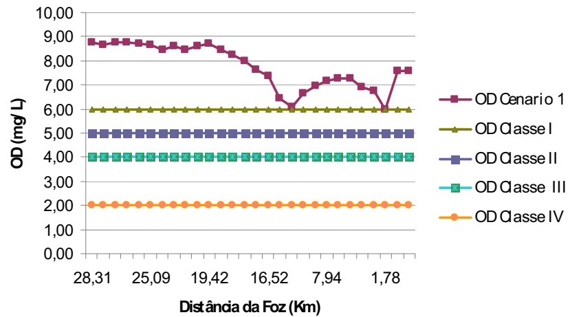
Figura 25: Comparação dos índices de OD observados no cenário 1 e os estabelecidos pela resolução CONAMA 357/05.
