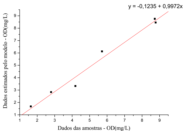
Figura 10: Regressão linear para os dados de OD das amostras e aqueles estimados pelo modelo QUAL2K.
