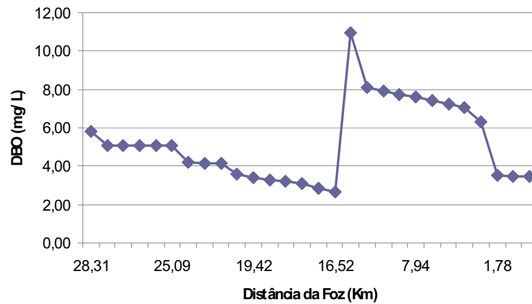
Figura 24: Detalhe do comportamento da DBO no cenário 1.
