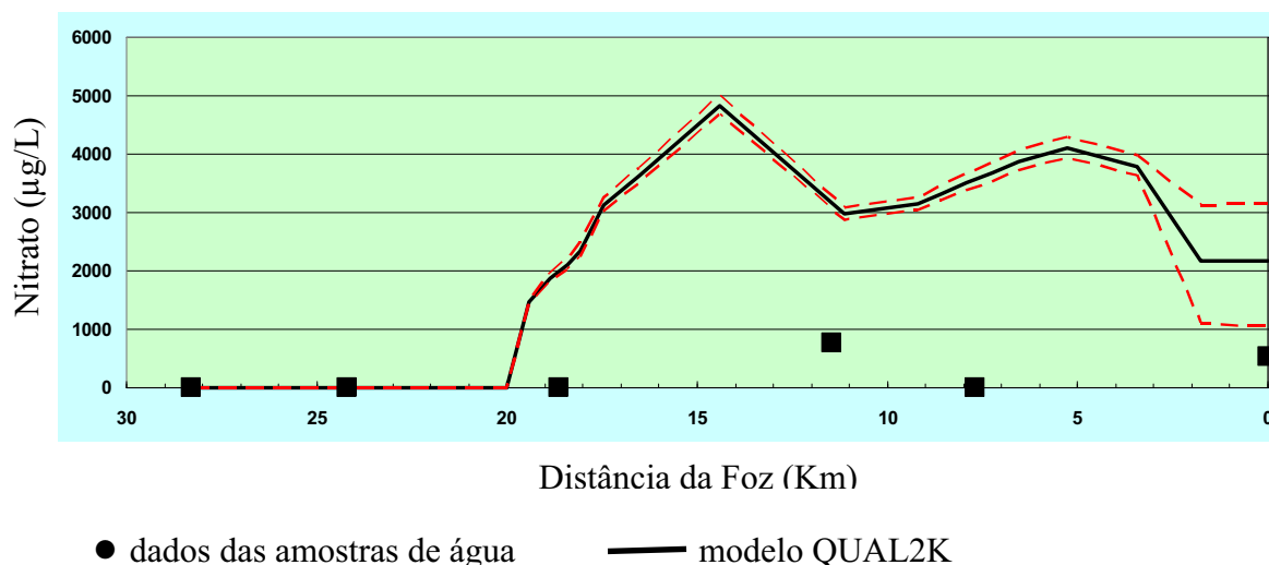
Figura 18: Comportamento da concentração de nitrato no segmento simulado do ribeirão Claro.
