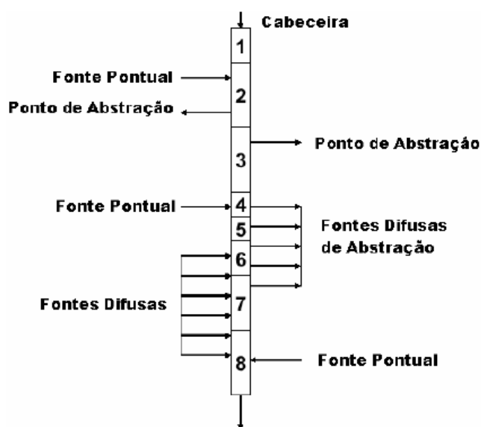
Figura 3: Representação de um corpo hídrico ausente de tributários (GONÇALVES & DIBIAZI, 2006).
