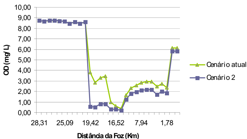
Figura 28: Comportamento da variável OD no cenário atual e em 2018 (Cenário 2).
