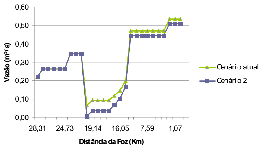
Figura 27 – Comportamento da vazão no cenário atual e no cenário futuro (ano de 2018)
