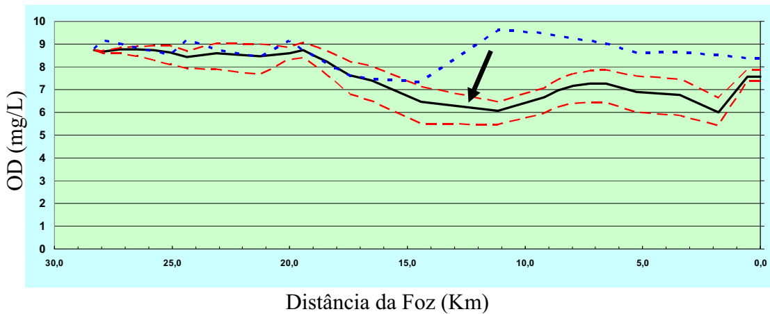
Figura 21: Comportamento da variável OD caso todo o efluente lançado no ribeirão Claro fosse tratado.
