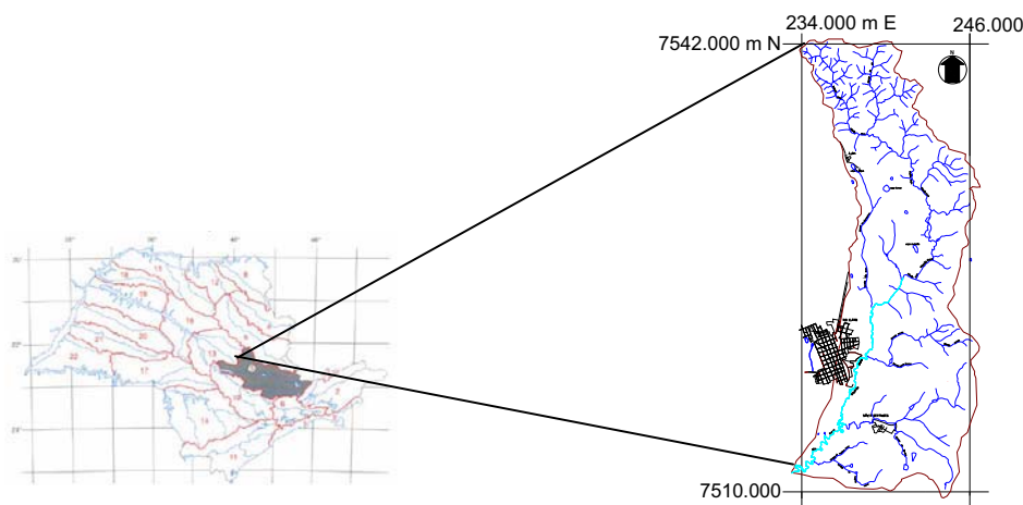
Figura 6: Bacia do ribeirão Claro na UGRHI nº 5 do Estado de São Paulo.
