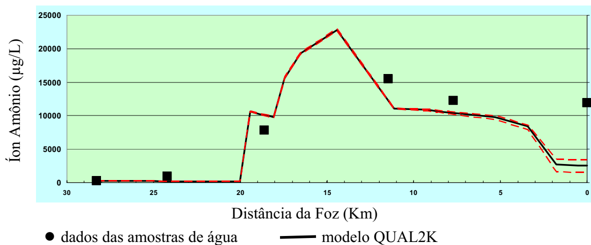
Figura 17: Comportamento da concentração de íons amônio no segmento simulado do ribeirão Claro.
