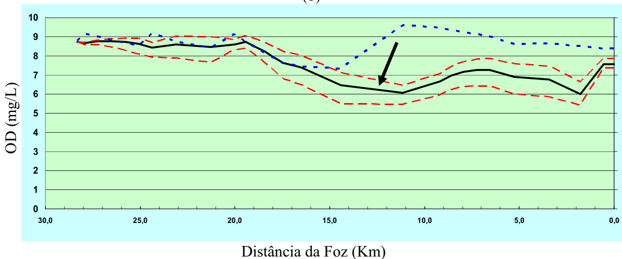
Figura 22: Comparação entre o perfil atual da variável OD (a) e o perfil de OD no primeiro cenário simulado (b).
