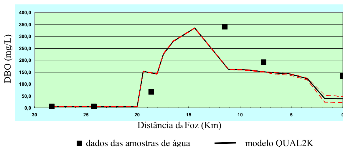
Figura 11 - Ajuste do modelo QUAL2K ao ribeirão Claro para a variável DBO
