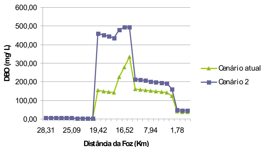
Figura 29-Comportamento da variável DBO no cenário atual e em 2018 (Cenário 2).
