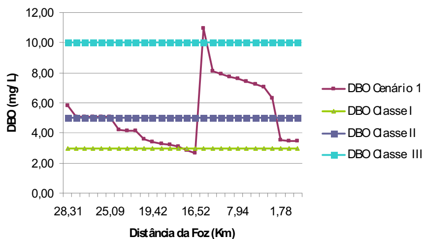
Figura 26: Comparação das concentrações de DBO do cenário 1 com os valores determinados pela resolução CONAMA 357/05.
