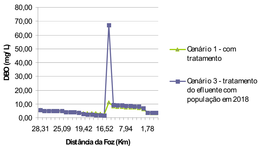
Figura 31: Comportamento da DBO no cenário 1 e 3.
