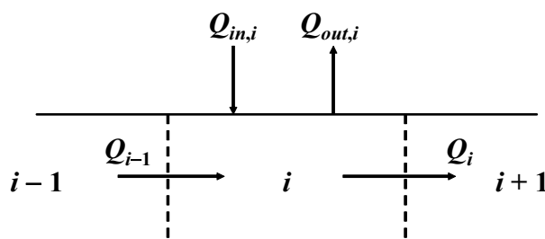
Figura 4: Balanço de vazão em um elemento i .
