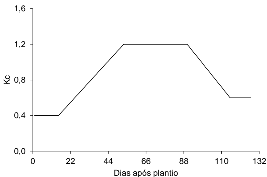
Figura 9 - Coeficiente de cultura (Kc) para a cultivar de milho AS 1555 PRO2.
