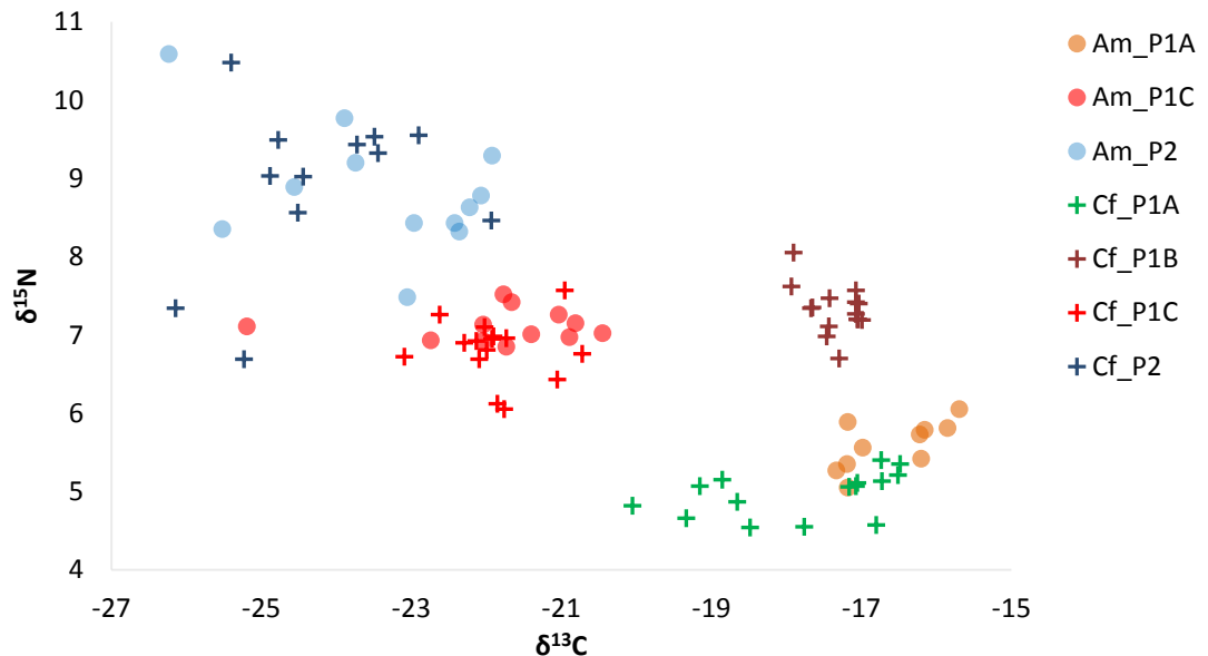
FIGURA 7. Valores de \delta^{13}\text{C} e \delta^{15}\text{N} de A. minuano (Am) e C. fulgens (Cf) entre os banhados amostrados (P1A, P1B, P1C e P2).
