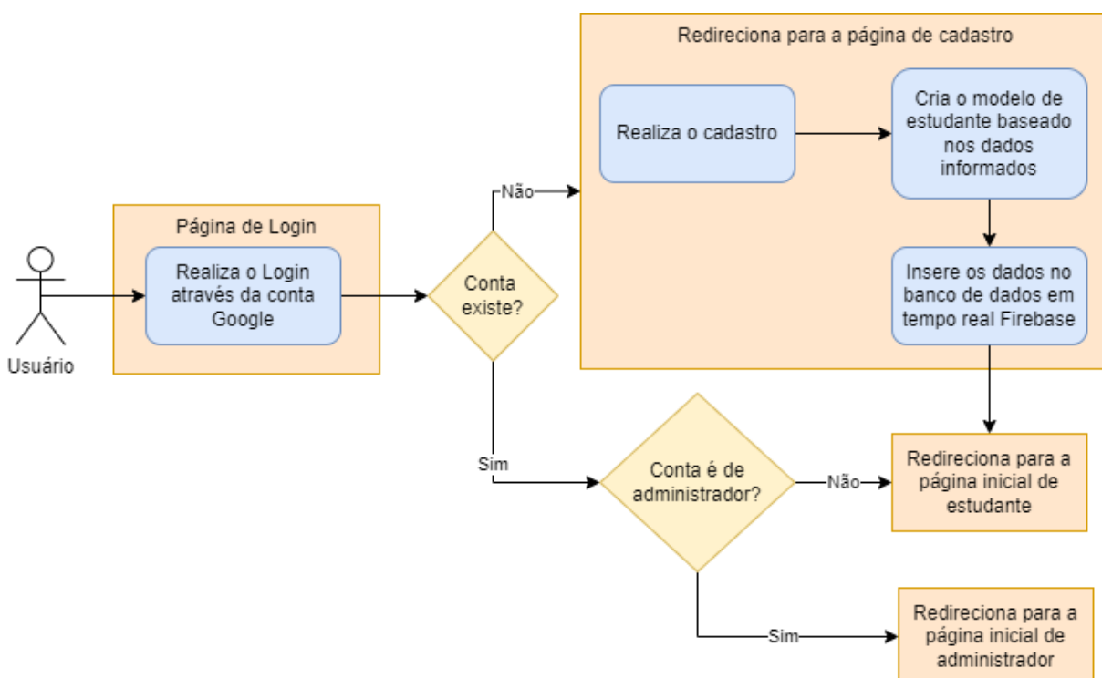
Figura 13 – Fluxo geral
