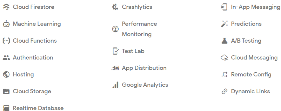
Figura 12 – Produtos Firebase
