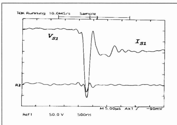
Figura 9 - Detalhe do disparo da chave S_1 Escala de tensão :50V/div Escala de corrente:2,5A/div Escala de tempo :500ns/div
