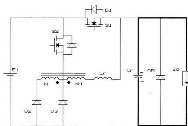
Figura 3h - 8ª etapa ( t_7, t_0 )
