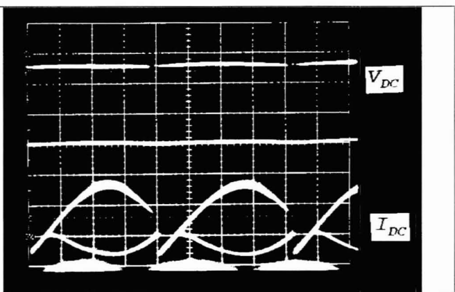
Figura 13 - Tensão e corrente no elo DC
