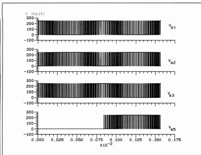
Figura 6 - Tensões nas chaves
