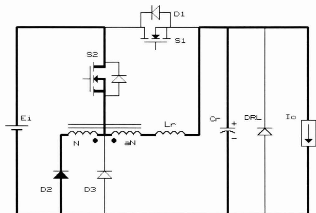
Figura 3c - 3ª etapa ( t_2, t_3 )
