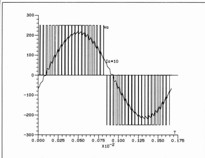
Figura 7 - Modulação com 40 pulsos por período
