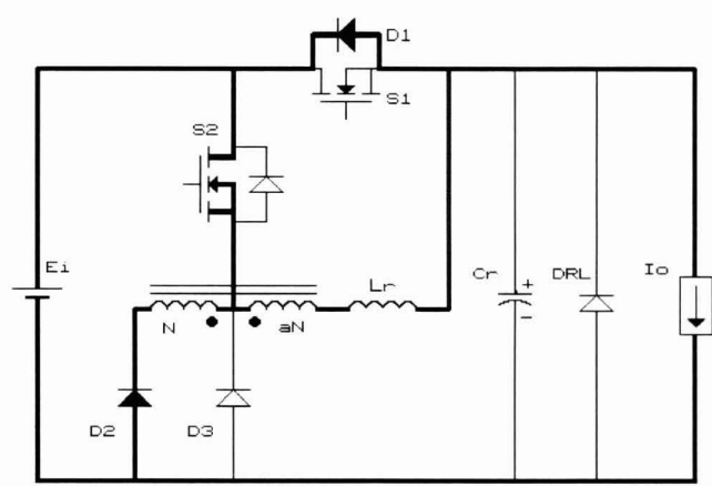
Figura 3d - 4ª etapa ( t_3, t_4 )
