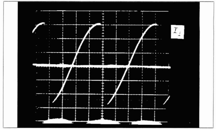
Figura 14 - Corrente na fonte para carga indutiva
