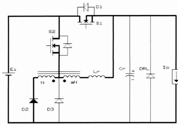
Figura 3e - 5ª etapa ( t_4, t_5 )
