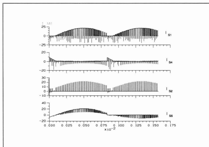
Figura 5 - Correntes nas chaves
