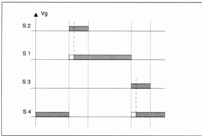
Figura 4 - Comando das chaves do estágio DC-DC
