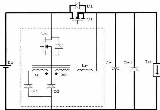
Figura 1 - Conversor buck com célula de comutação ZVS
