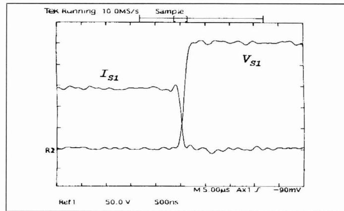
Figura 10 - Detalhe do bloqueio da chave S_1 Escala de tensão :50V/div Escala de corrente :2,5A/div Escala de tempo :500ns/div
