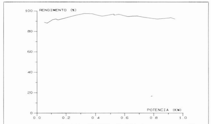
Figura 15 - Característica de rendimento do conversor
