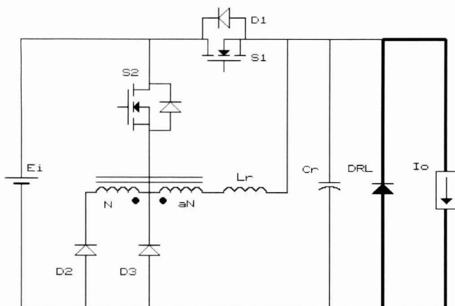
Figura 3a - 1ª etapa ( t_0, t_1 )
