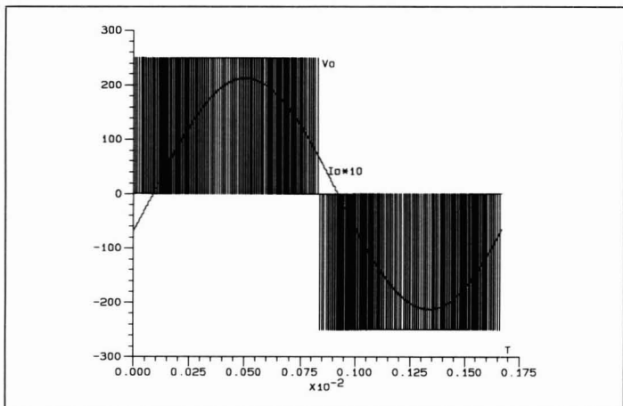
Figura 8 - Modulação com 168 pulsos por período
