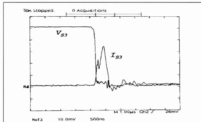
Figura 11 - Detalhe da comutação da chave S_3 Escala de tensão :50V/div Escala de corrente:5A/div Escala de tempo :500ns/div
