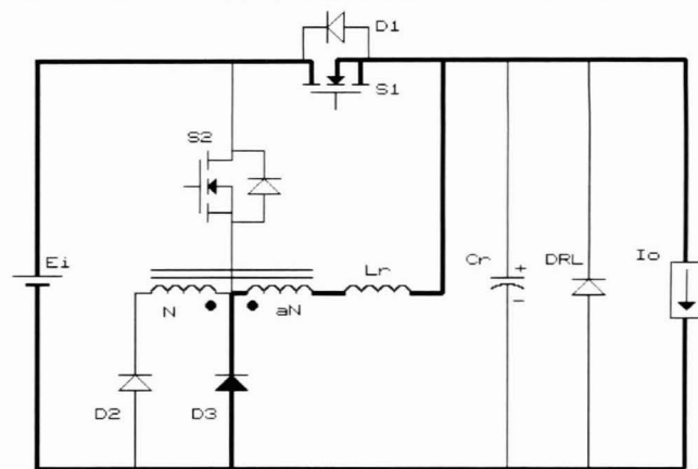
Figura 3f - 6ª etapa ( t_5, t_6 )
