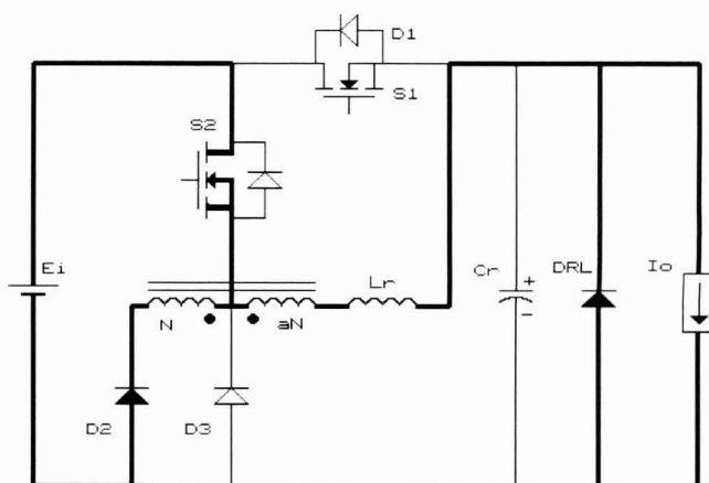
Figura 3b - 2ª etapa ( t_1, t_2 )
