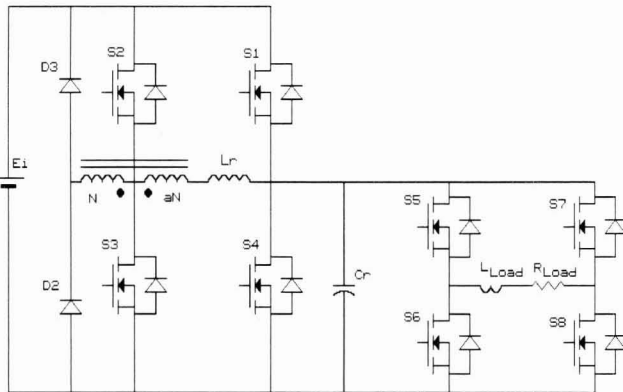
Figura 2 - Conversor DC-AC proposto
