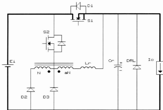
Figura 3g - 7ª etapa ( t_6, t_7 )
