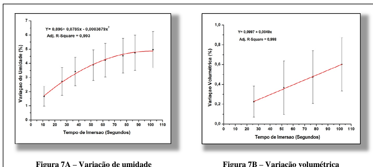
Figura 7. Variação média de umidade ( \Delta_U ) e da variação volumétrica ( \Delta_V ) determinados pelo método de imersão em função do tempo em segundos
