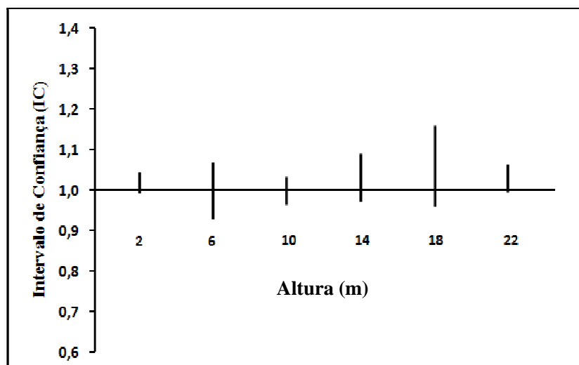
Figura 12. Gráfico de intervalo de confiança ( IC ) entre as determinações da densidade básica pelo Método de atenuação da radiação gama e o Método de imersão em água, para as amostras selecionadas por região a cada quatro metros.
