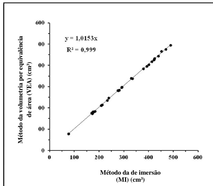
Figura 9. Gráfico de correlação do volume ( V ) determinado, pelo método de imersão ( MI ) e método da volumetria por equivalência de área ( VEA ), das amostras G_i da espécie de Eucalyptus sp.
