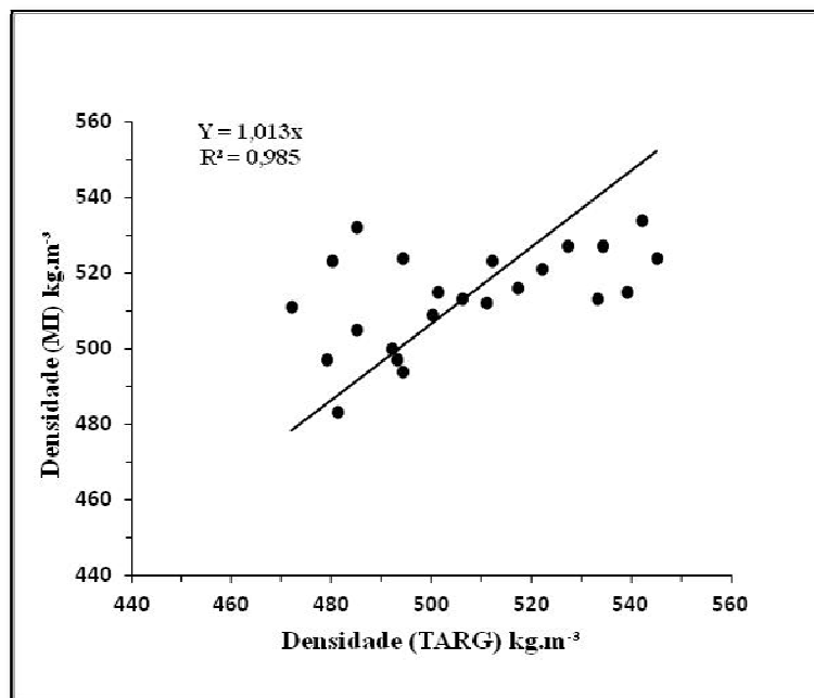
Figura 11. Comparação da densidade básica determinada pelo Método de imersão e o Método de atenuação da radiação gama das amostras da espécie de Eucalyptus sp.
