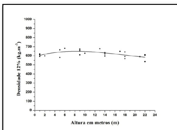
Figura 14. Variação média da densidade aparente a 12% em ( \text{kg.m}^{-3} ) das amostras A_i , B_i , C_i , e D_i na direção longitudinal em função da altura (m) da espécie de Eucalyptus sp.
