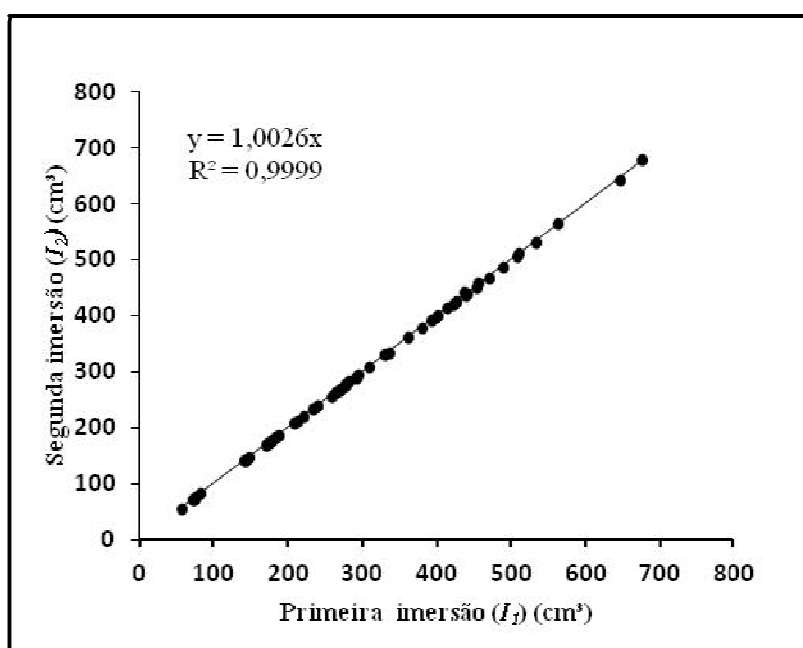
Figura 8. Variação do volume (cm 3 ) em consecutivas imersões em água, primeira ( I_1 ) e a segunda ( I_2 ), pelo método de imersão de amostras de Eucalyptus sp.
