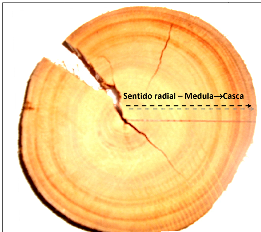
Figura 6. Linha radial no sentido medula-casca, por onde o feixe de radiação incide perpendicularmente, para mensuração da densidade das amostras
