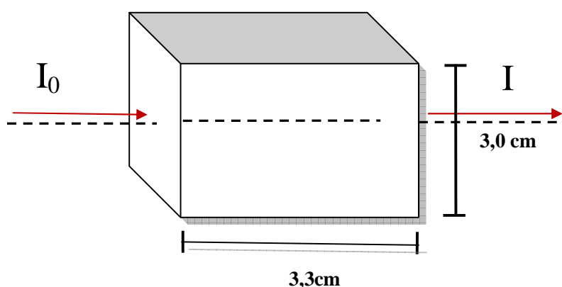
Figura 5. Recipiente para a calibração do aparelho utilizado para determinar o coeficiente de atenuação de massa ( \mu ) pelo Método de atenuação da radiação gama
