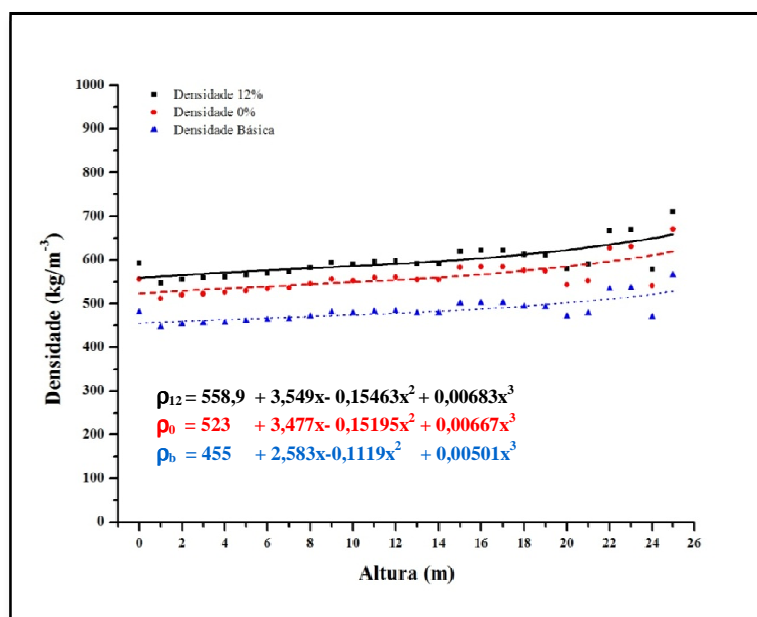
Figura 16. Variação média de densidade (kg.m -3 ) a 12%, 0% e básica de discos coletados a cada metro da altura de árvores da espécie de Eucalyptus sp.
