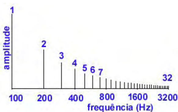
Figura 15: Configuração de um som com uma frequência fundamental de 100 Hz Fonte: Campos (2006)
