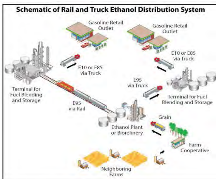
Ilustração 4 - Esquema do sistema de distribuição do etanol por trens e caminhões
