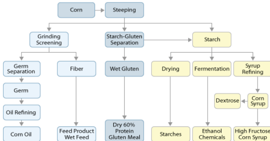
Ilustração 2- Processo de moagem úmida do milho para fabricação de etanol
