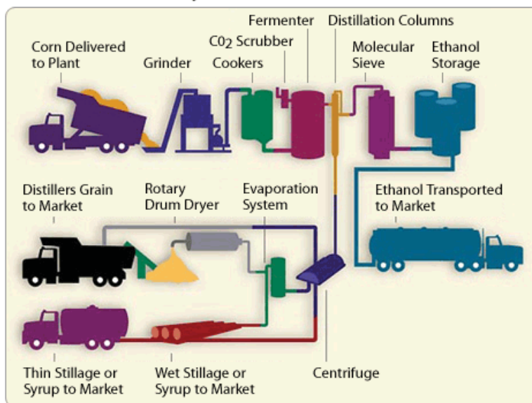
Ilustração 3 - Processo de moagem seca do milho para fabricação de etanol
