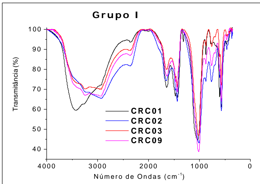
Figura 83 – Sobreposição dos espectros de absorção na região do infravermelho das amostras de cálculos renais do grupo I.
