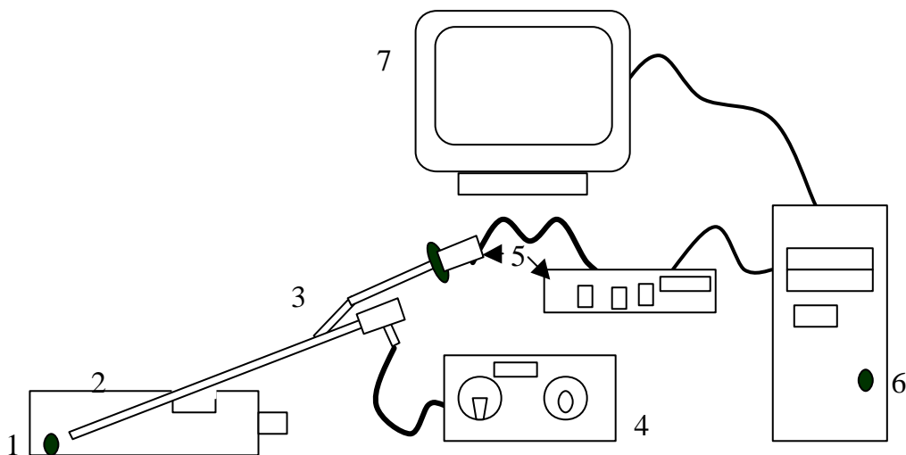
Figura 28 - Esquema demonstrando o equipamento montado
