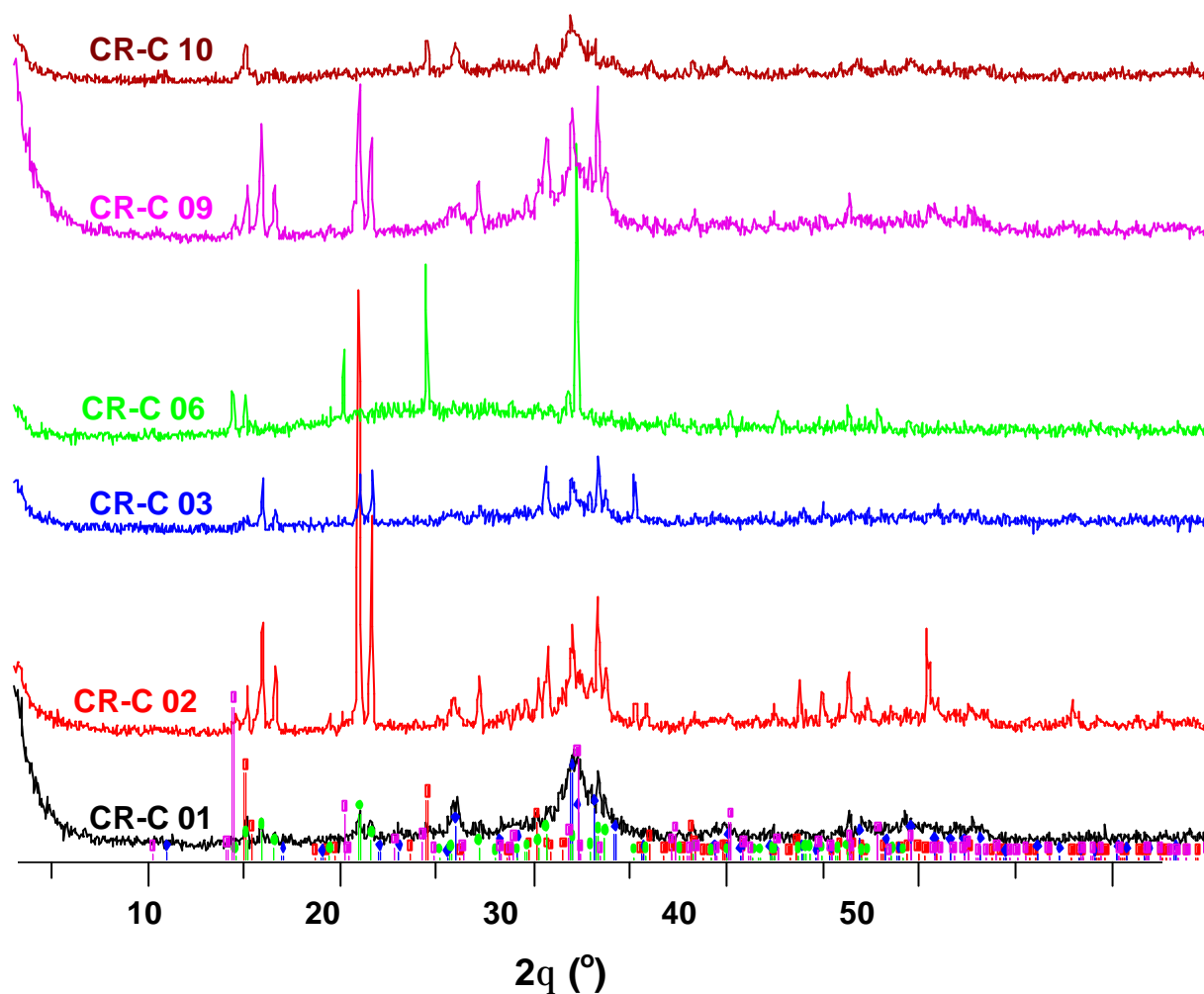
Figura 89 – Sobreposição dos difratogramas de raios X das amostras CR-C 01, CR-C 02, CR-C 03, CR-C 06, CR-C 09 e CR-C 10.
