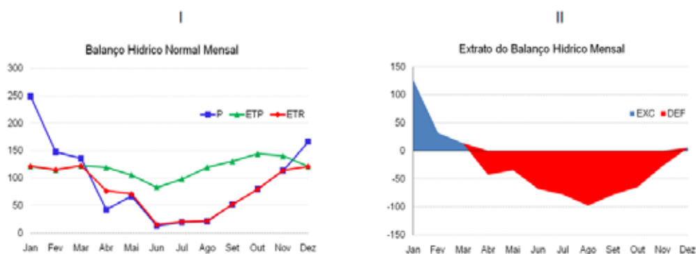
Figura 2 - Variação dos dados mensais meteorológicos de precipitação (P), evapotranspiração potencial (ETP) e evapotranspiração real (ETR) (I) e extrato do balanço hídrico mensal (II) através do método de Thorthwaite e Mather (1955).
