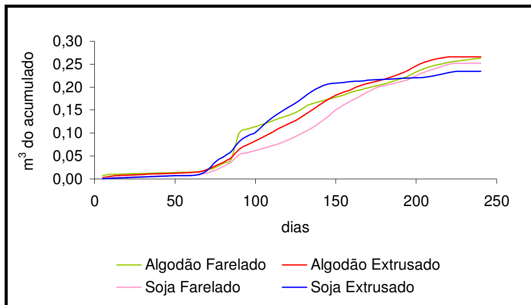
Figura 2. Produção acumulada de biogás em m 3 , produzido por dejetos de animais em terminação, em função dos tratamentos.
