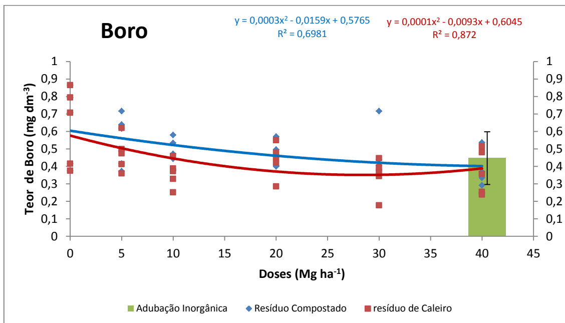
Figura 27. Teores de boro observados nos solos e ajuste das regressões para as médias dos teores de boro nos solos com eucalipto, em função das doses de resíduo compostado e resíduo de caleiro, e teor médio de boro em solos com eucalipto submetido à adubação inorgânica, após 5 meses.
