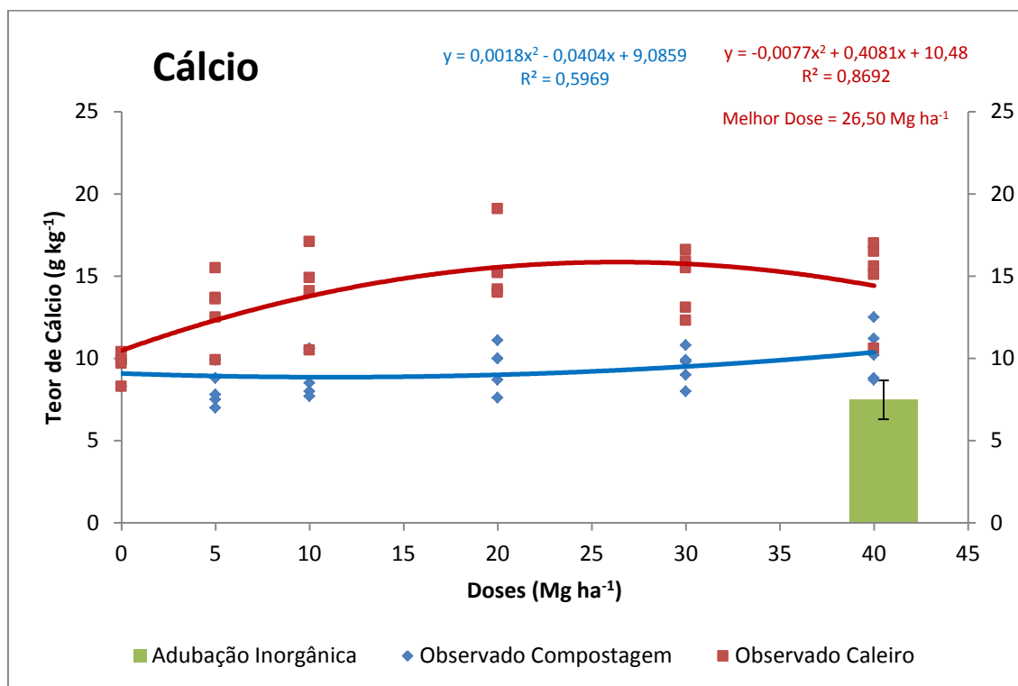
Figura 34. Teores de cálcio observados das folhas de eucalipto e ajuste das regressões para as médias dos teores de cálcio nas folhas de eucalipto, em função das doses de resíduo compostado e resíduo de calcário, e teor médio de cálcio em folhas de eucalipto submetido à adubação inorgânica, após 5 meses.
