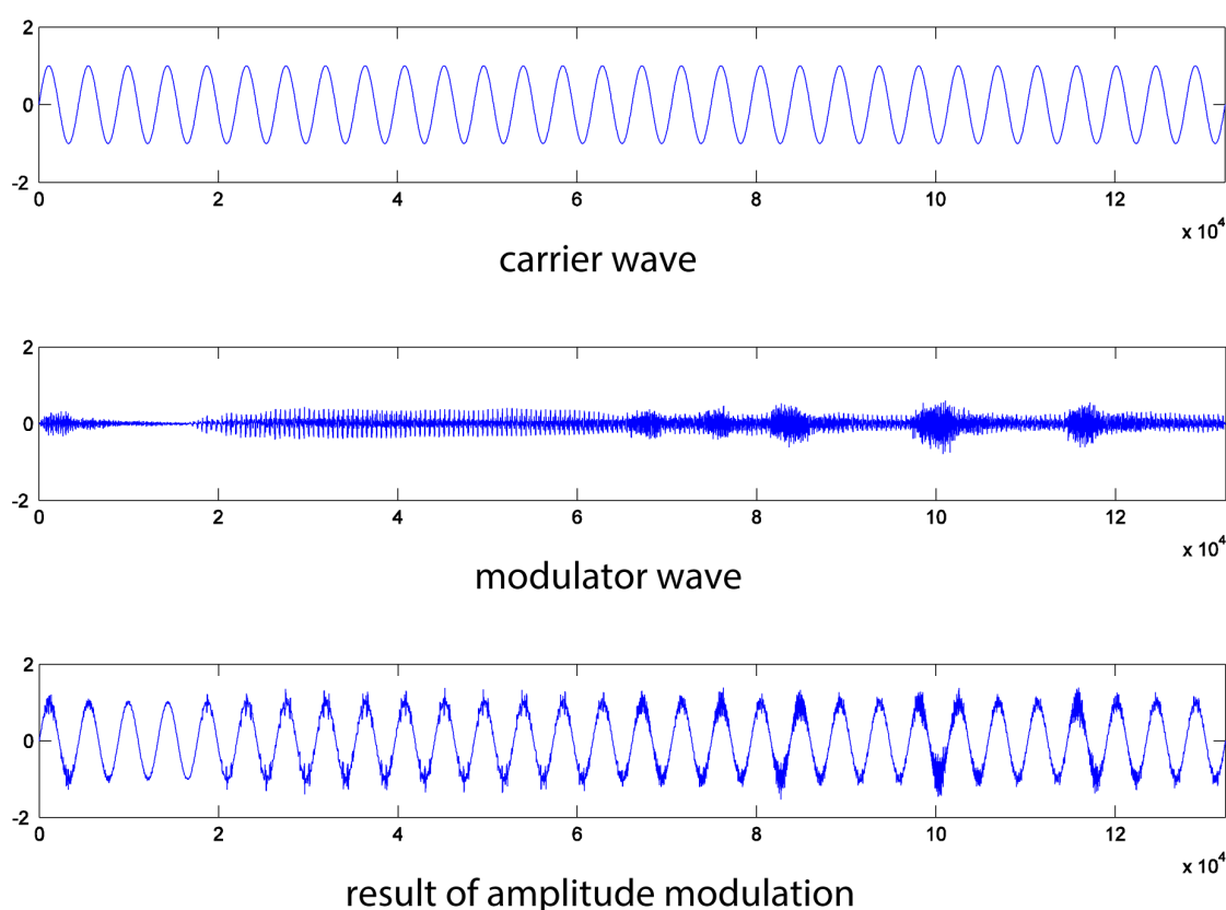
Figura 12 – Gráfico de modulação de uma forma de onda digital.
