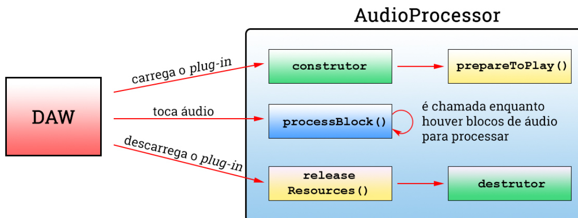
Figura 30 – Ciclo de vida de um objeto do tipo AudioProcessor.
