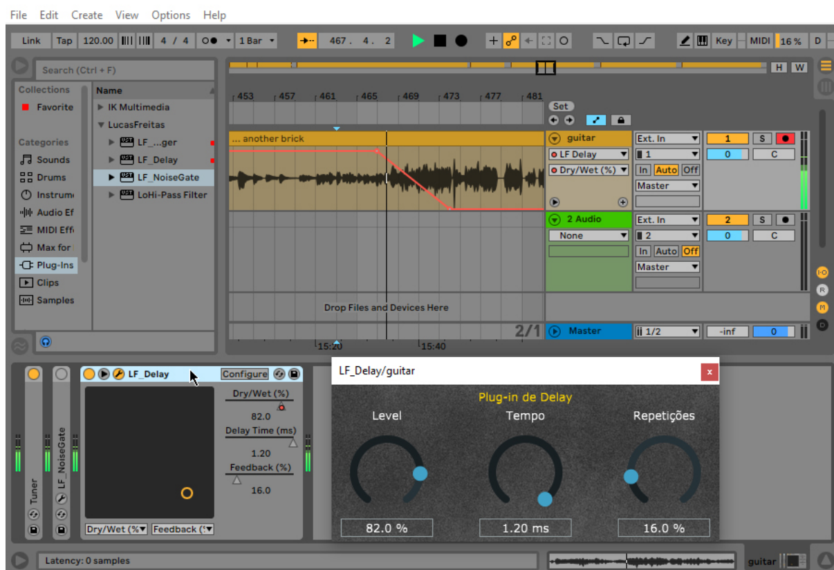
Figura 24 – Automação de parâmetro com o Ableton Live 10.
