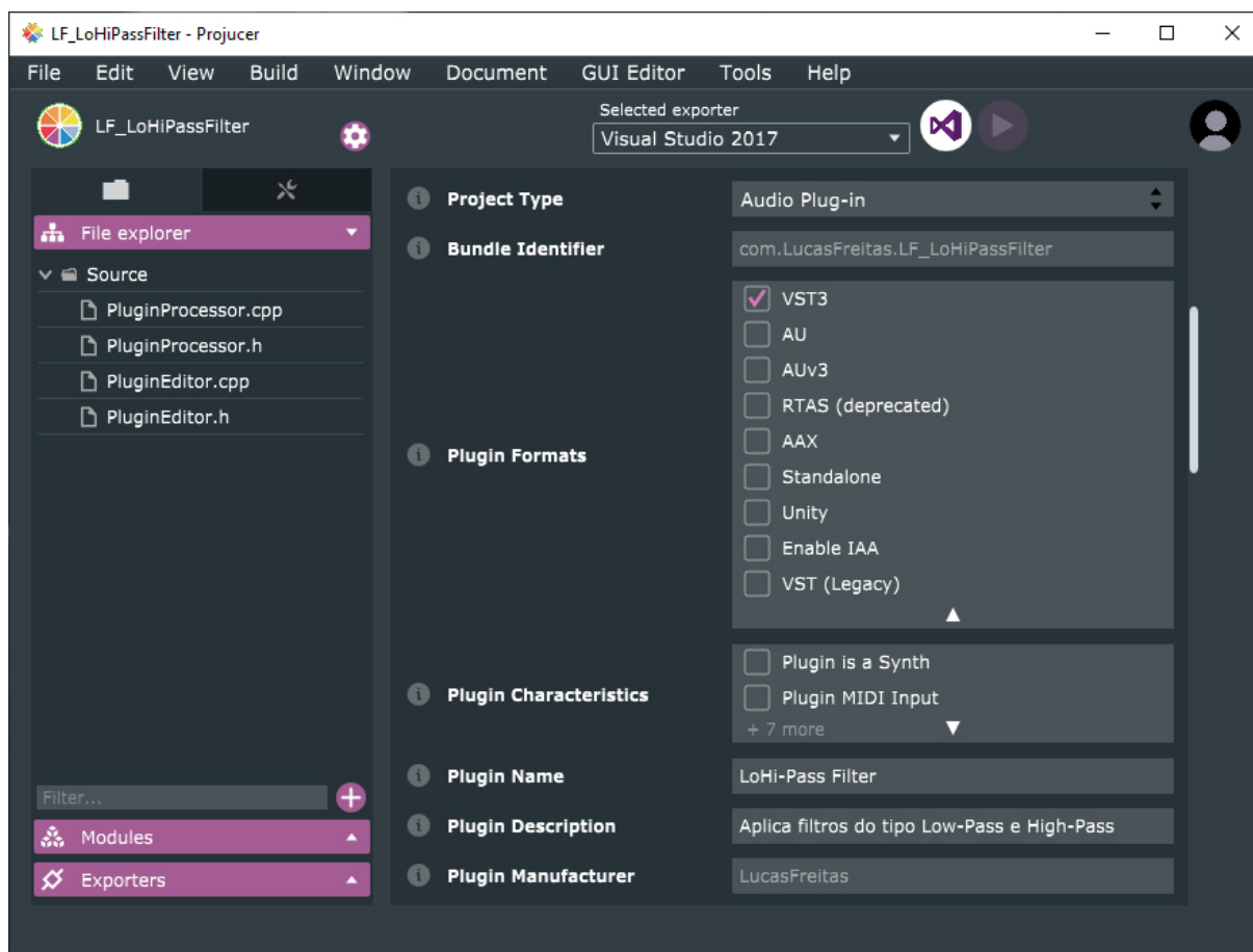
Figura 23 – Configurações de um projeto no Projucer.
