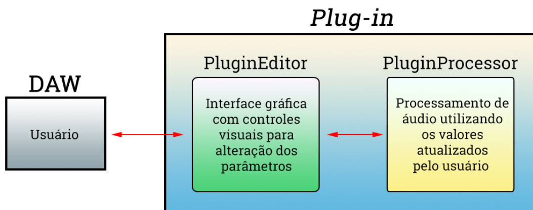
Figura 29 – Diagrama de interface do plug-in com a DAW.
