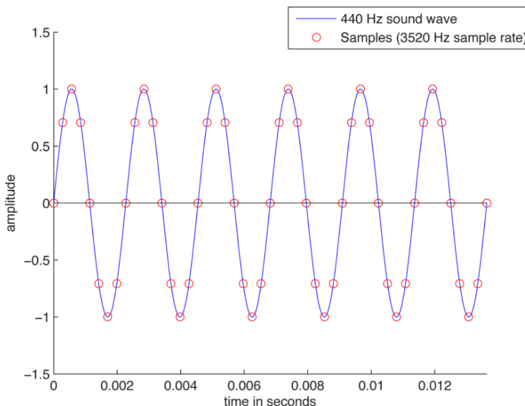
Figura 19 – Processo de amostragem de um sinal.
