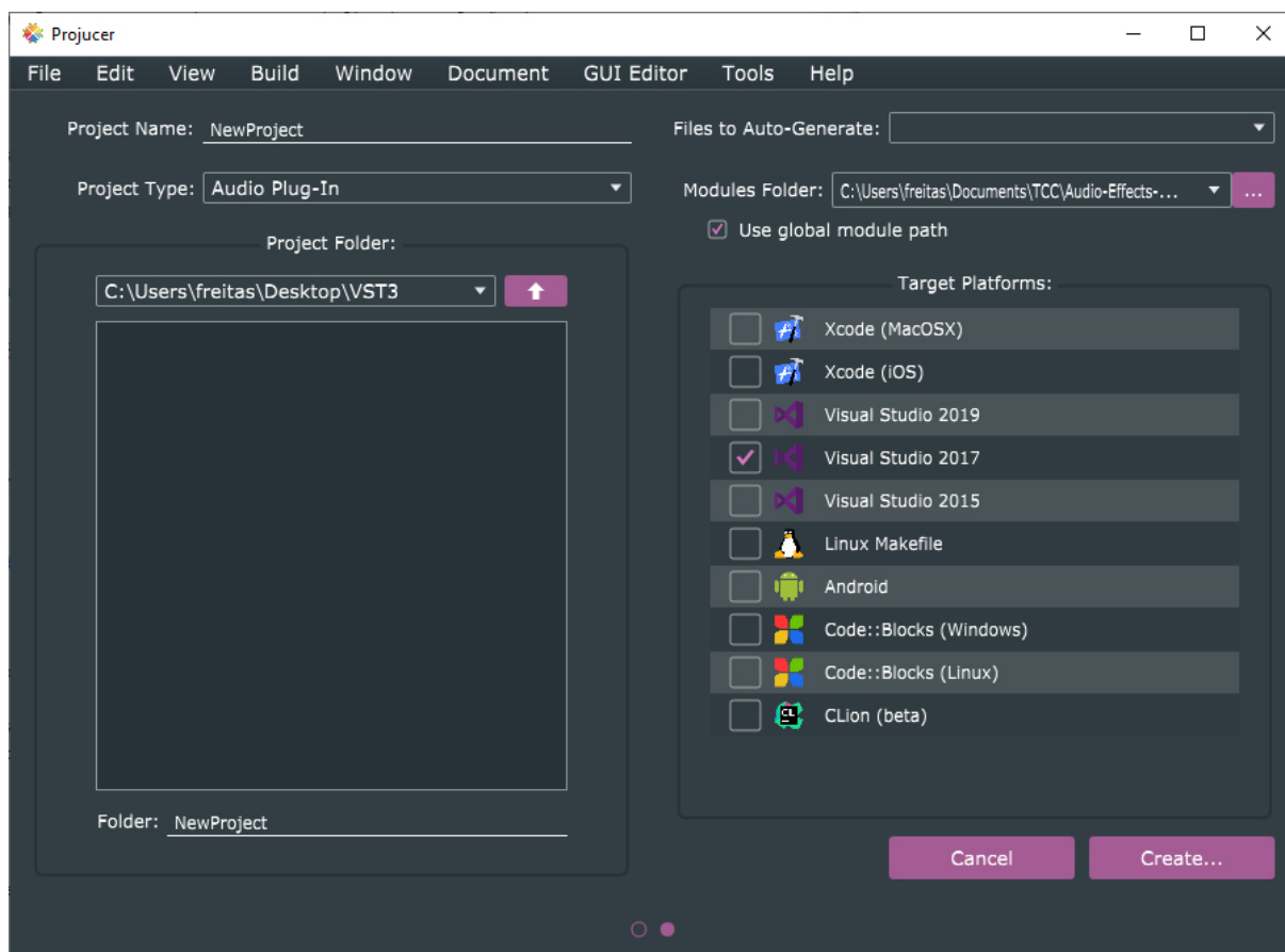
Figura 22 – Plataformas-alvo para exportação no Projucer.
