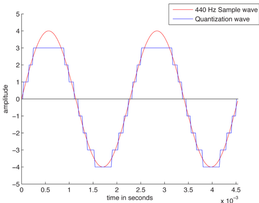
Figura 20 – Processo de quantização de um sinal com 3 bits de resolução.
