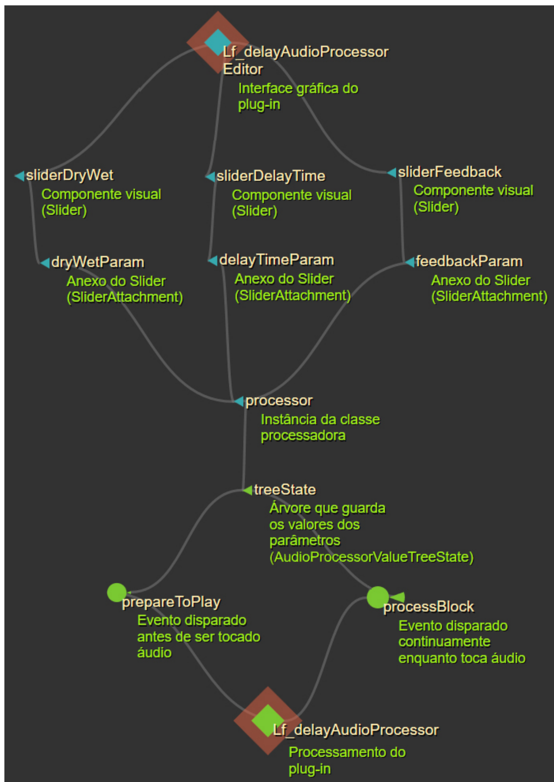
Figura 31 – Fluxograma de comunicação entre a classe editora visual e a processadora.
