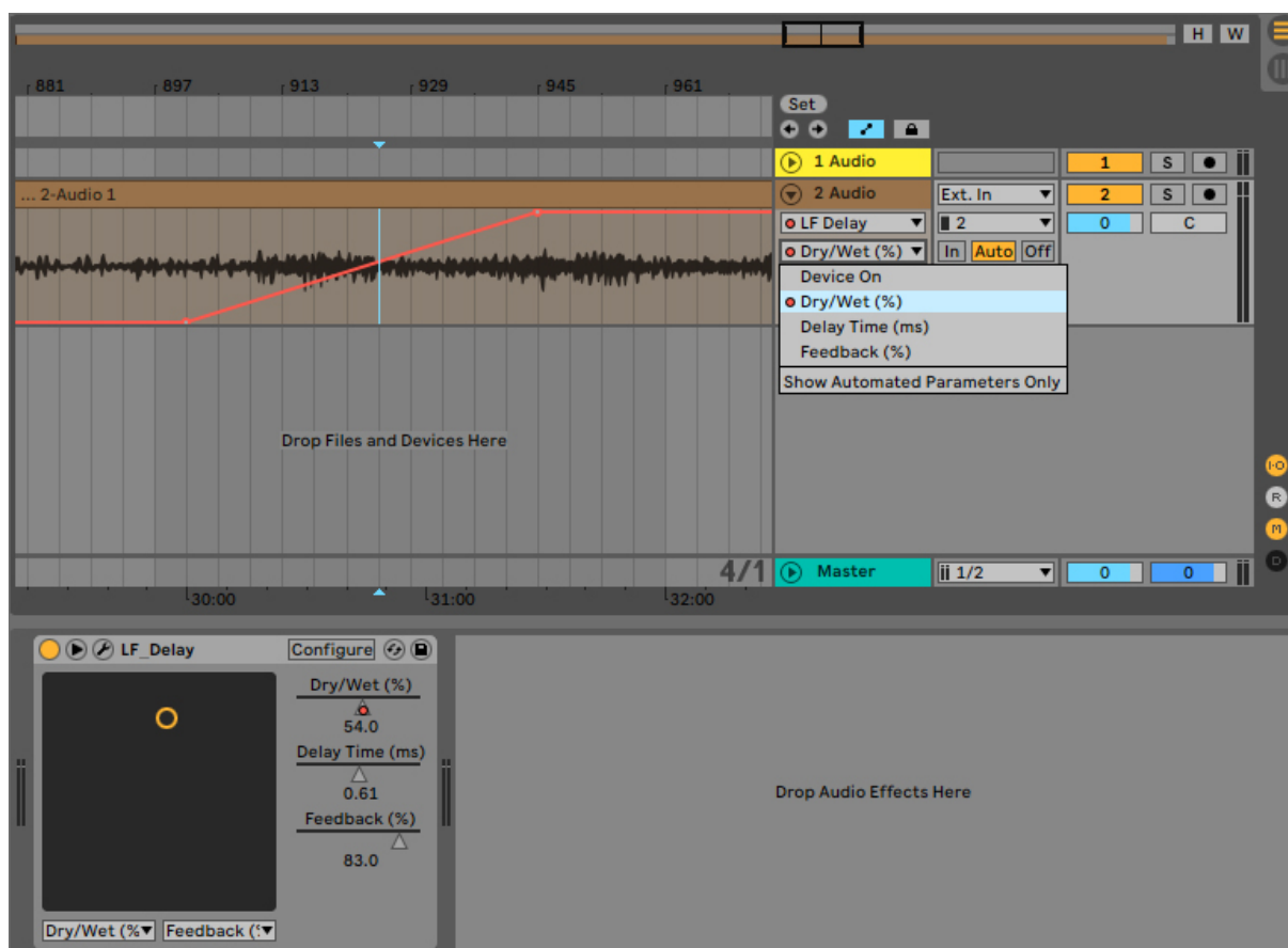
Figura 18 – Automação de parâmetros pela DAW.
