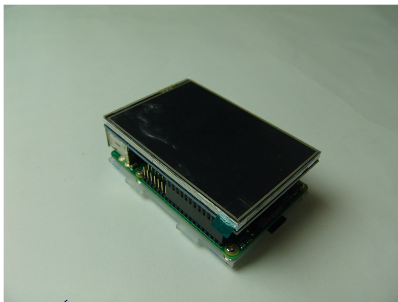
Figura 13 – Raspberry Pi somente com a tela sensível ao toque.
