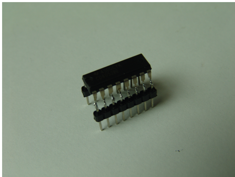
Figura 10 – Foto do multiplexador CD4052 utilizado no dispositivo com terminais soldados para facilitar a ligação com os jumpers.
