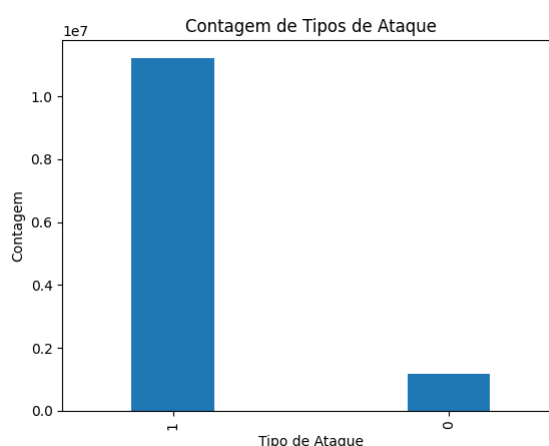
Figura 8 – Comparação das amostras desbalanceadas de sessão normal e ataque
