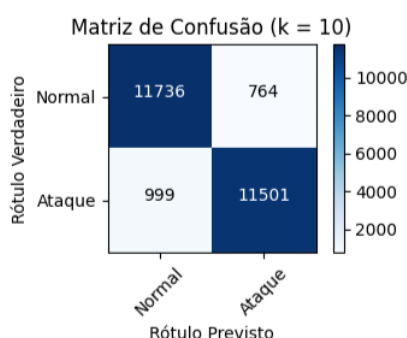
Figura 16 – KNN: matriz de confusão para número de vizinhos igual a 10
