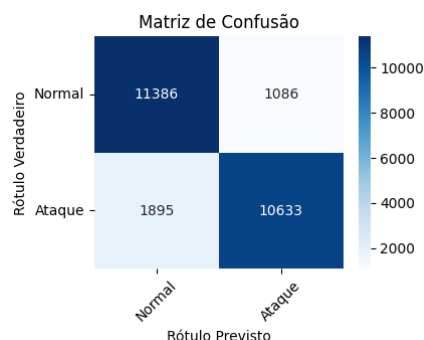
Figura 15 – MLP: matriz de confusão para ativador ReLU e otimizador Adam
