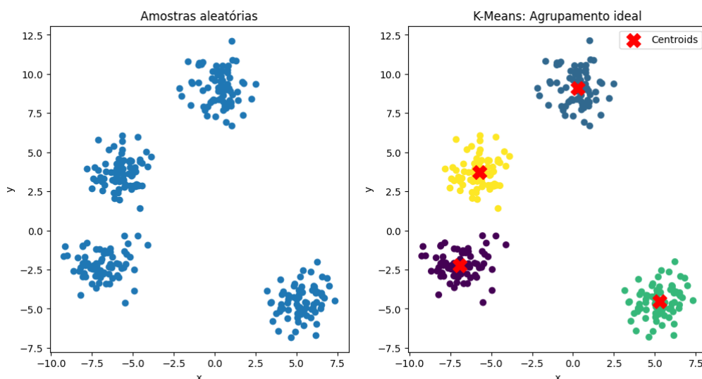
Figura 3 – K-Médias: um exemplo de clusterização
