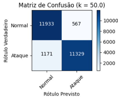
Figura 13 – SVM: matriz de confusão para valor de C igual a 50
