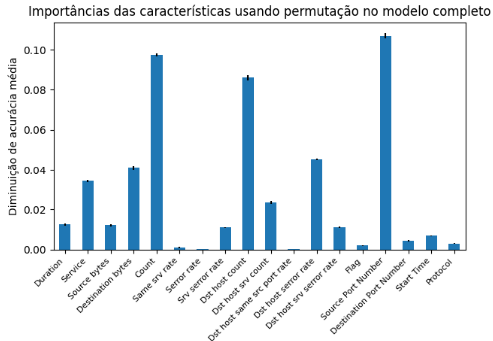
Figura 11 – Importância das características usando Feature Permutation
