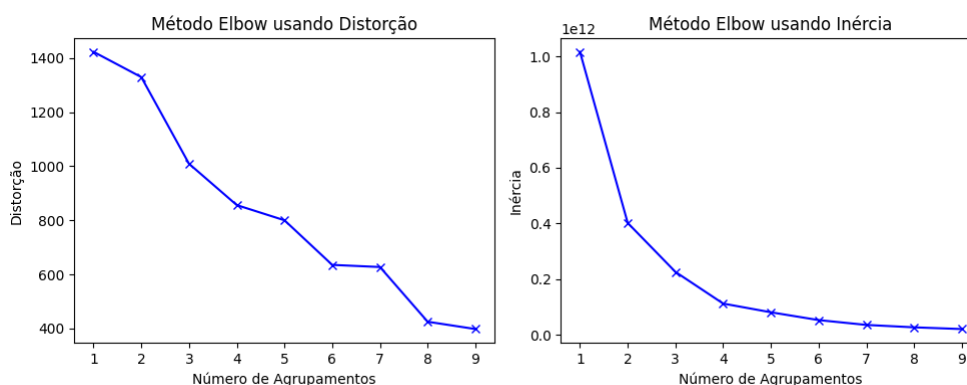
Figura 17 – Método Elbow: encontrando o número ideal de clusters
