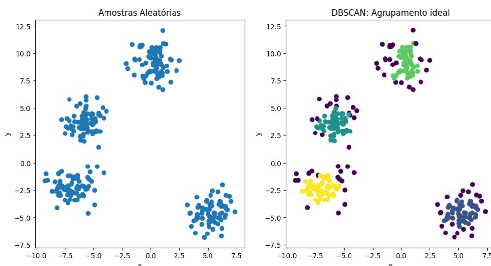
Figura 4 – DBSCAN: um exemplo de clusterização
