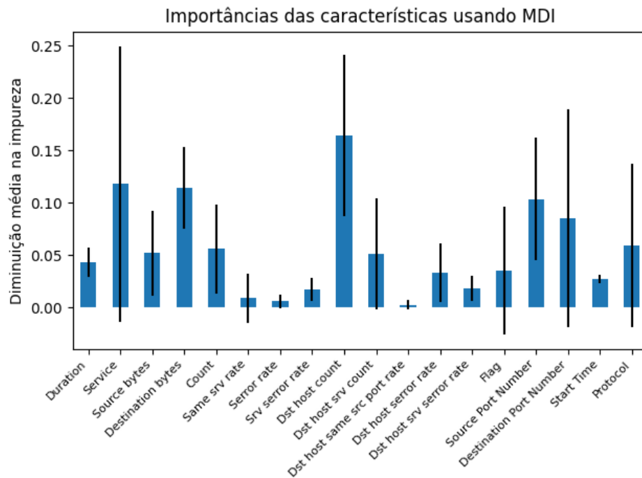
Figura 10 – Importância das características usando Mean Decrease in Impurity
