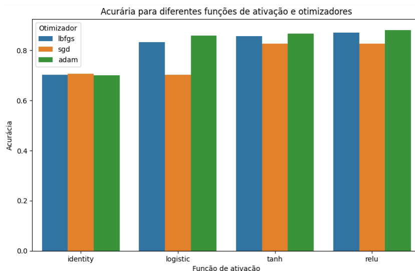
Figura 14 – MLP: comparação dos modelos para diferentes combinações de ativação e otimização
