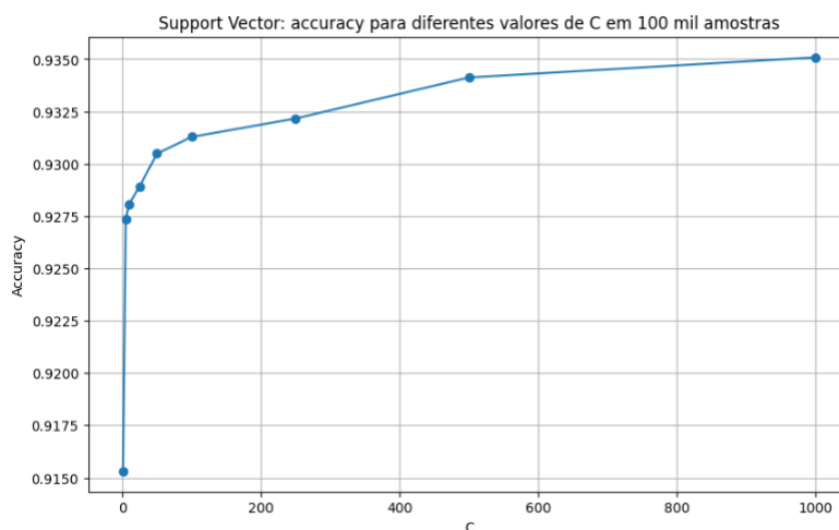
Figura 12 – SVM: accuracy para diferentes valores de C em 100 mil amostras
