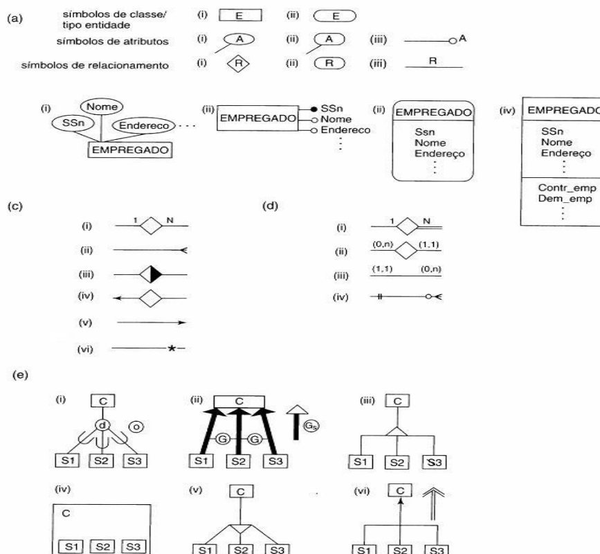
Figura 5 – Exemplos de Fluxos de Entidades-Relacionamentos (ELMASRI; NAVATHE, 2005).
