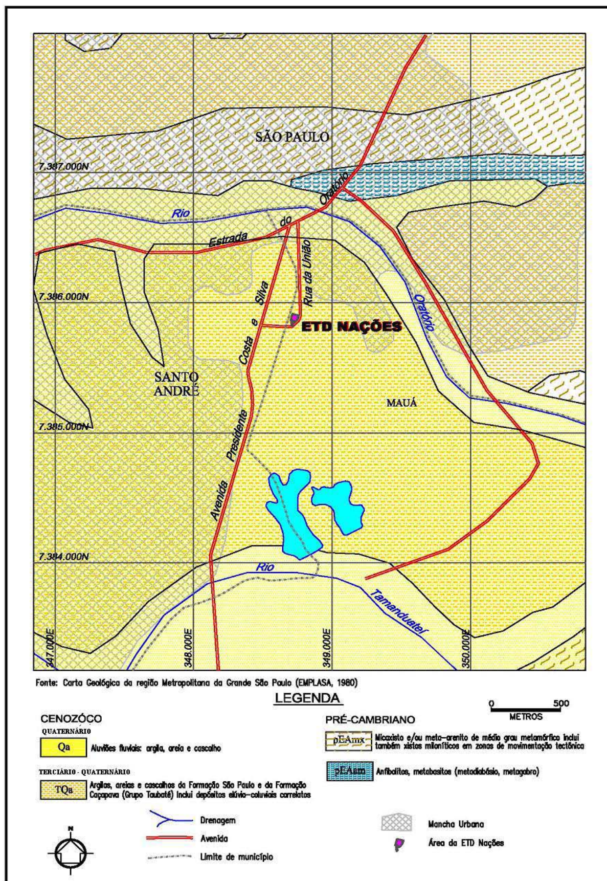
Figura 73 – Carta Geológica Regional (EMPLASA, 1980).
