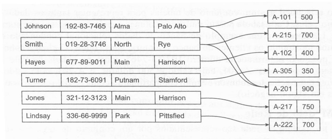
Figura 7 – Exemplo de banco de dados sob o modelo relacional (SILBERSCHATZ et al., 1999).
