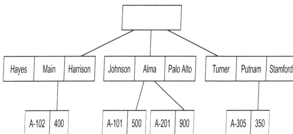
Figura 6 – Exemplo de banco de dados em formato hierárquico (SILBERSCHATZ et al., 1999).
