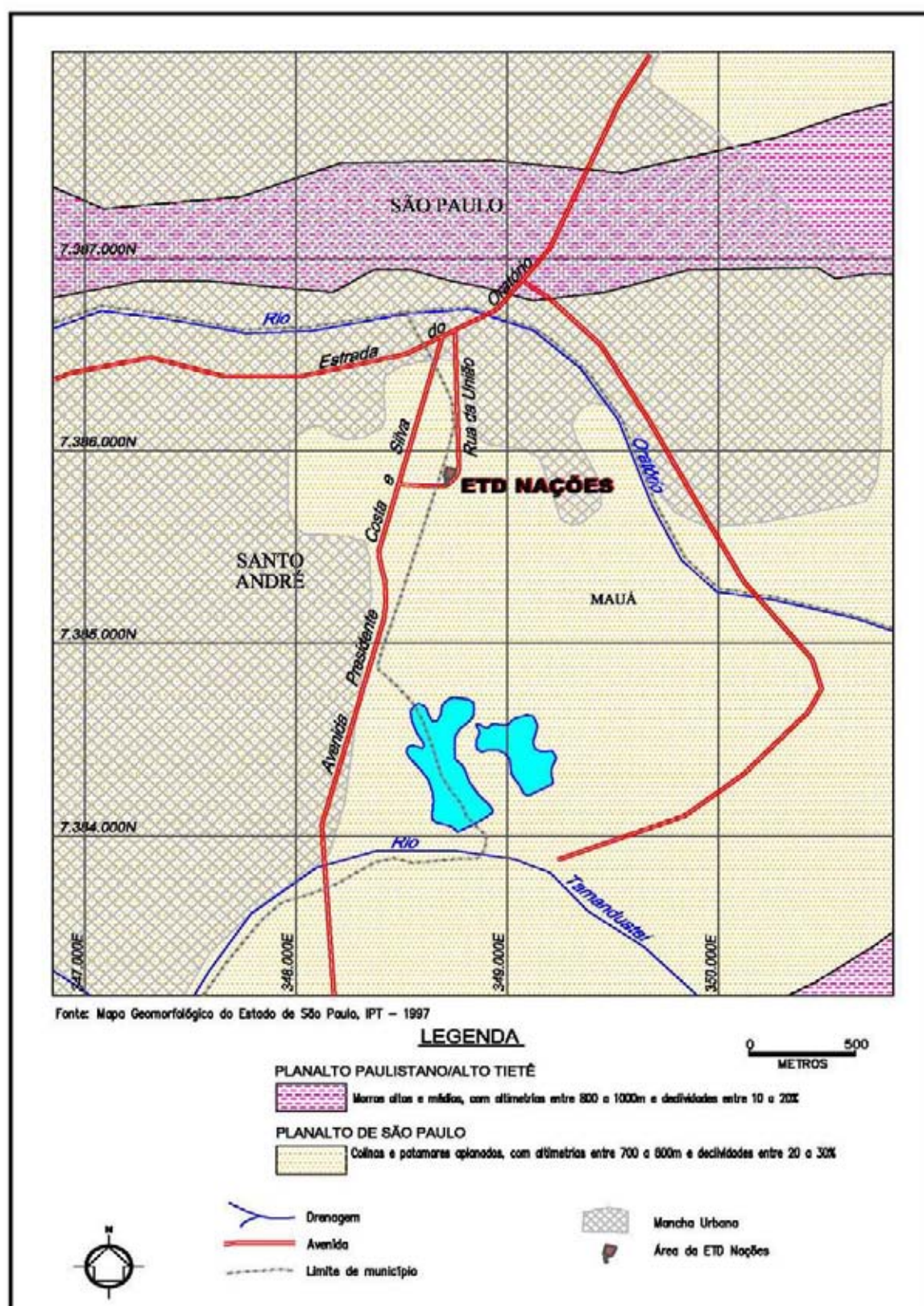
Figura 74 – Compartimentação das unidades de relevo em que se insere o perfil geomorfológico da região do empreendimento (ROSS; MOROZ, 1997).
