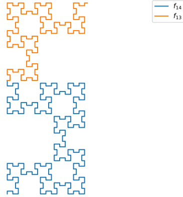
Fractal da palavra de Fibonacci f_{15} de comprimento F_{15} = 610
