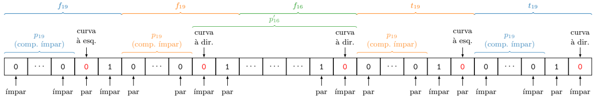
Figura 4.21: Decomposição de f_{22} em palíndromos
