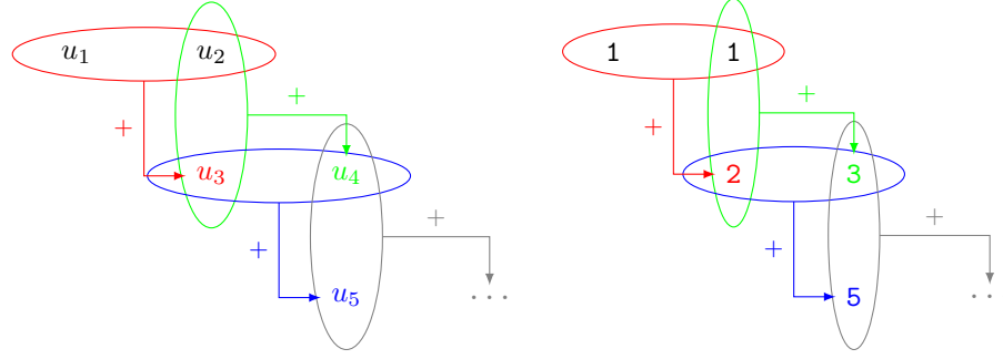
Figura 2.1: Construção da sequência de Fibonacci
