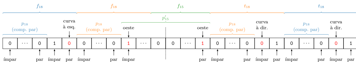
Figura 4.26: Decomposição de f_{21} em palíndromos
