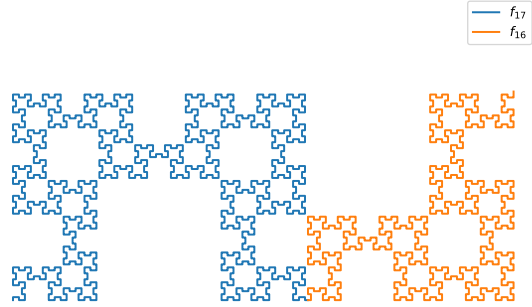
Fractal da palavra de Fibonacci f_{18} de comprimento F_{18} = 2584
