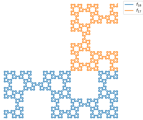
Fractal da palavra de Fibonacci f_{19} de comprimento F_{19} = 4181
