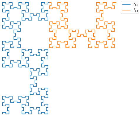
Fractal da palavra de Fibonacci f_{16} de comprimento F_{16} = 987
