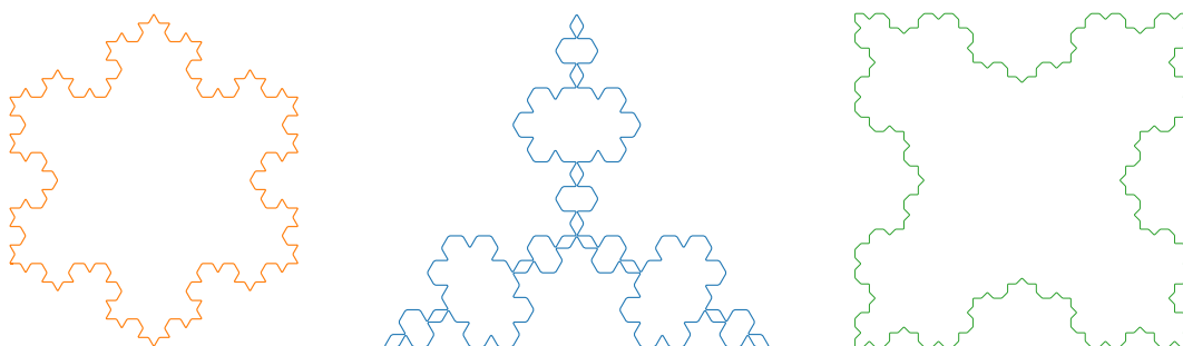
Figura 4.38: Floco de neve de Koch e suas variações
