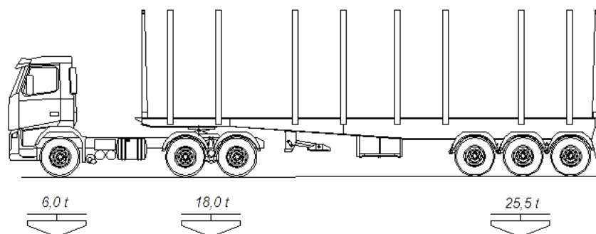
Figura 5. CVC T12-S3 utilizada no transporte rodoviário da madeira no Uruguai.
