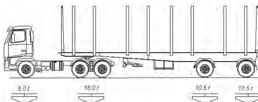
Figura 4. CVC T12-S2 utilizada no transporte rodoviário da madeira no Uruguai.
