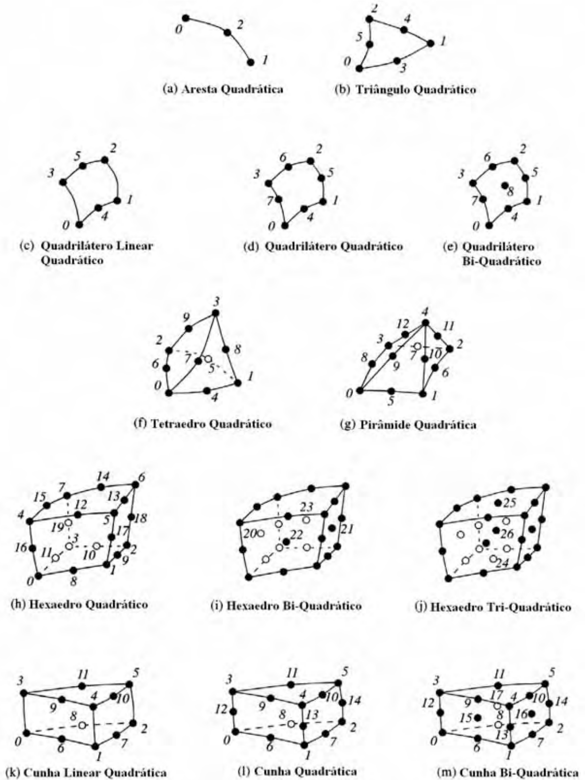
Figura 4.12 – Células não-lineares encontradas no VTK.
