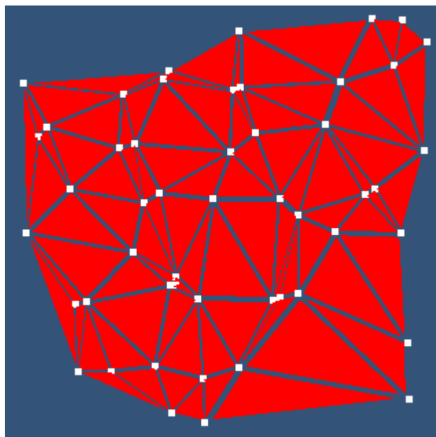
Figura 4.14 – Exemplo de uma malha não-estruturada, gerada com bioMeshCreate.
