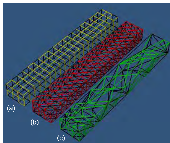
Figura 5.9 – (a) Viga constituída por malha poligonal; (b) malha triangular gerada sobre a viga; (c) simplificação de 60% da malha triangular gerada. / Fonte: O autor.
