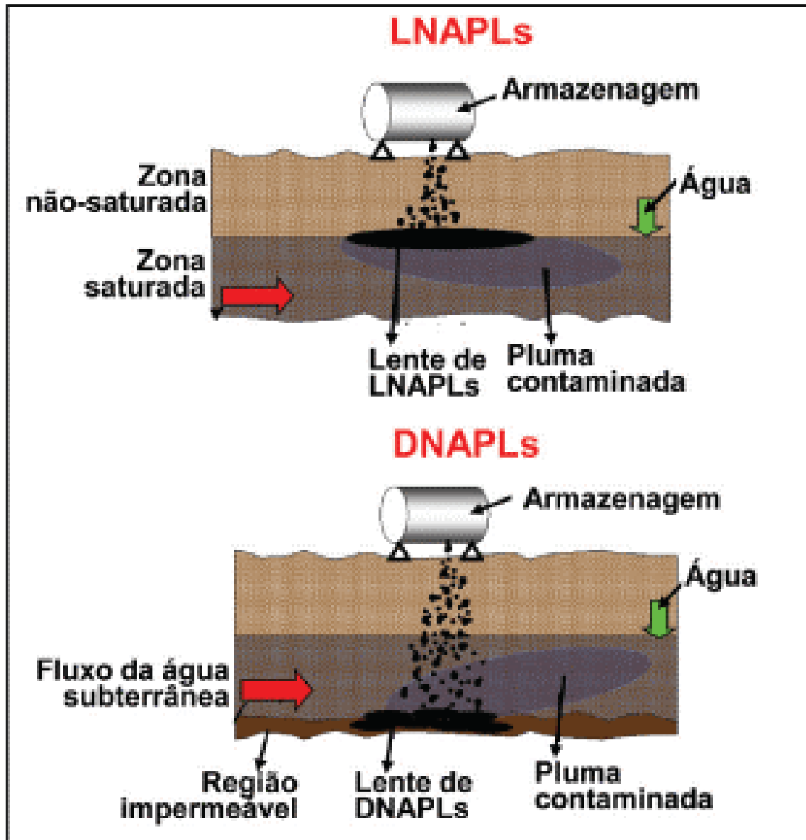
Figura 1: Esquema representando a contaminação do subsolo e de aquíferos causada por vazamentos de LNAPLs e DNAPLs.
