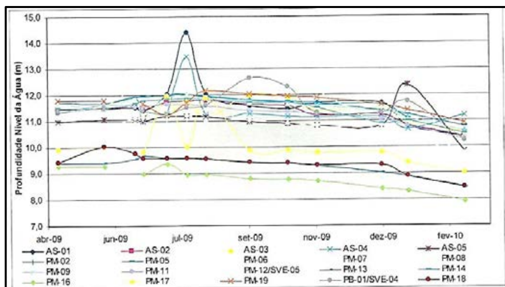
Figura 31: Evolução dos Níveis de Água nos Poços
