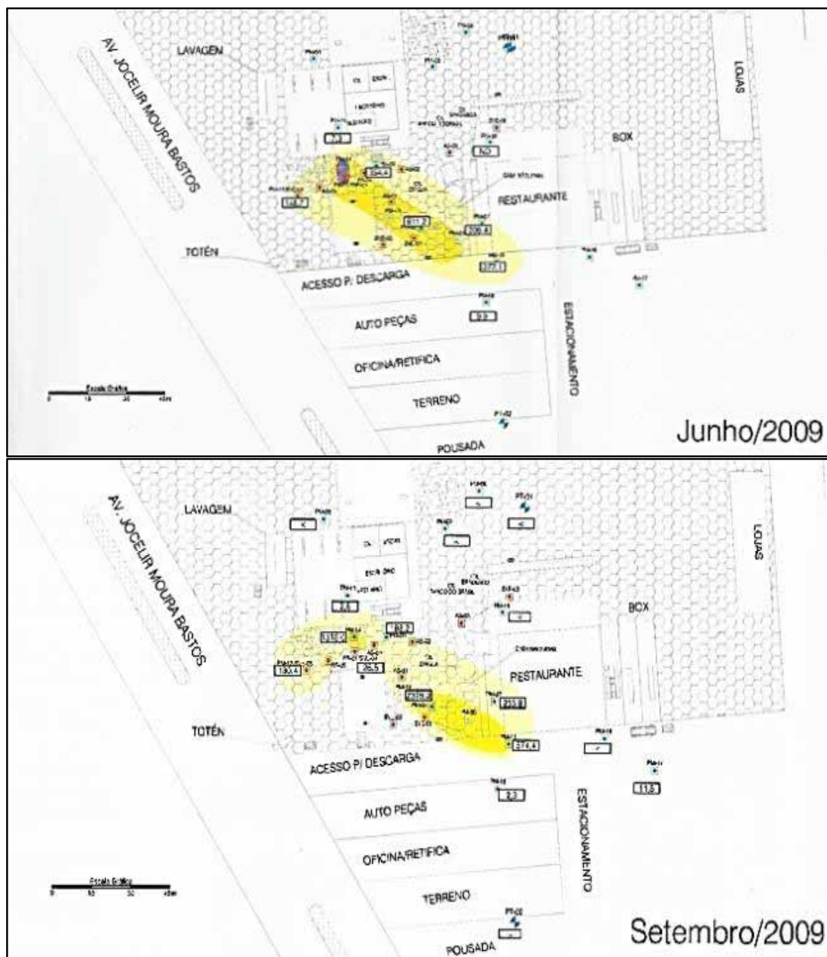
Figura 36: Evolução das Concentrações de Benzeno na Área (cont.) Fonte: Relatório CETESB 2010
