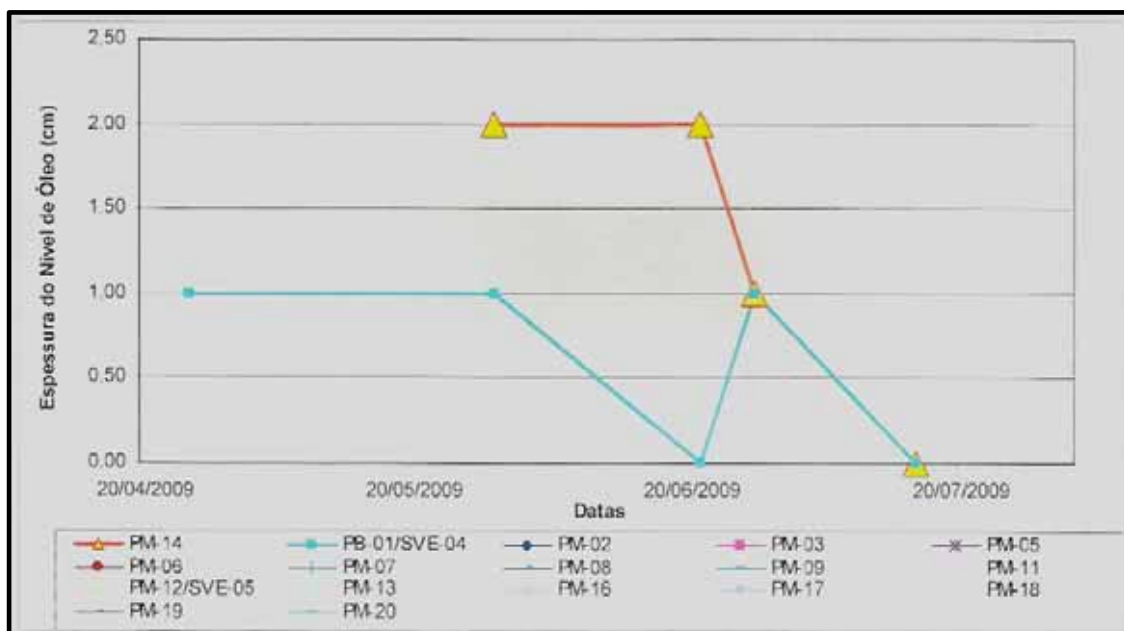
Figura 25: Evolução da espessura de fase livre
