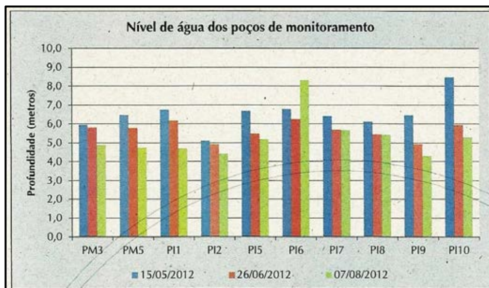
Figura 46: Medição dos níveis de água dos poços de monitoramento.
