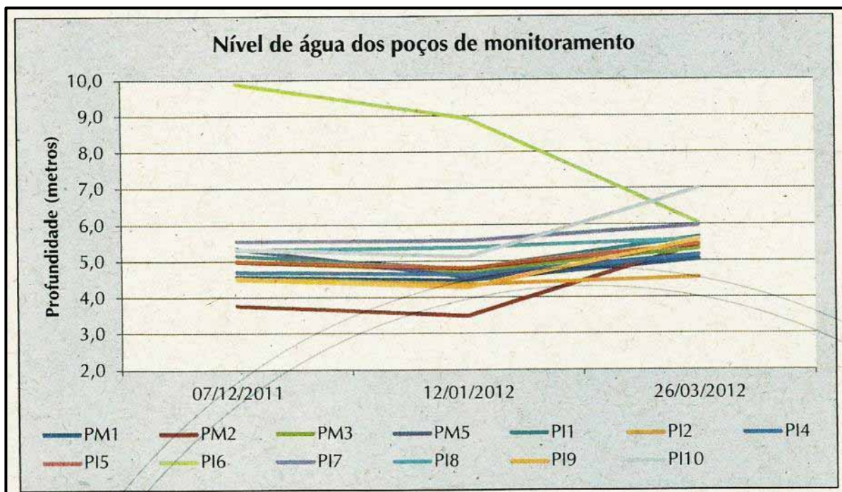
Figura 43: Medição dos níveis de água dos poços de monitoramento.
