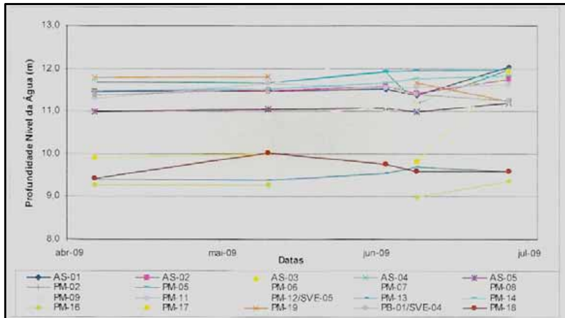
Figura 24: Evolução dos níveis de água
