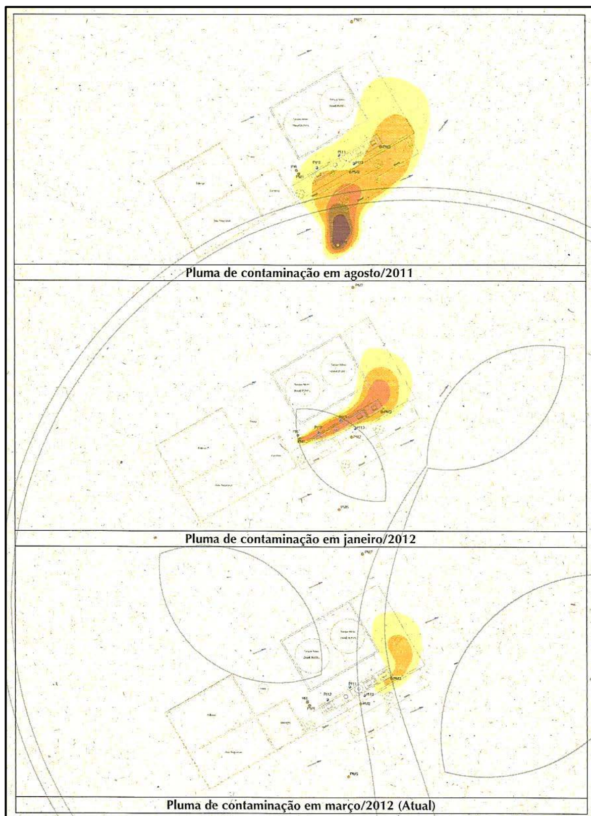
Figura 45: Comparação entre as plumas de contaminação Fonte: Relatório CETESB, 2012
