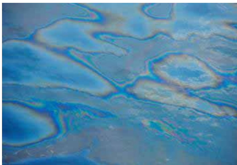
Figura 8: Iridescência na água causada por mancha de óleo.
