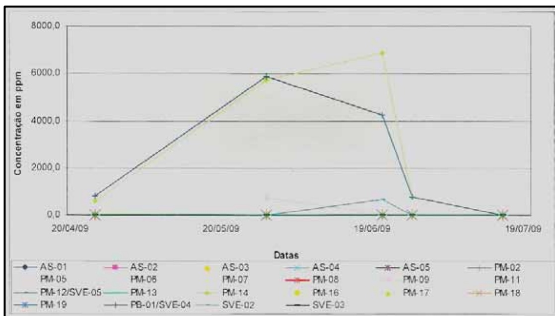
Figura 26: Evolução das Concentrações de VOC
