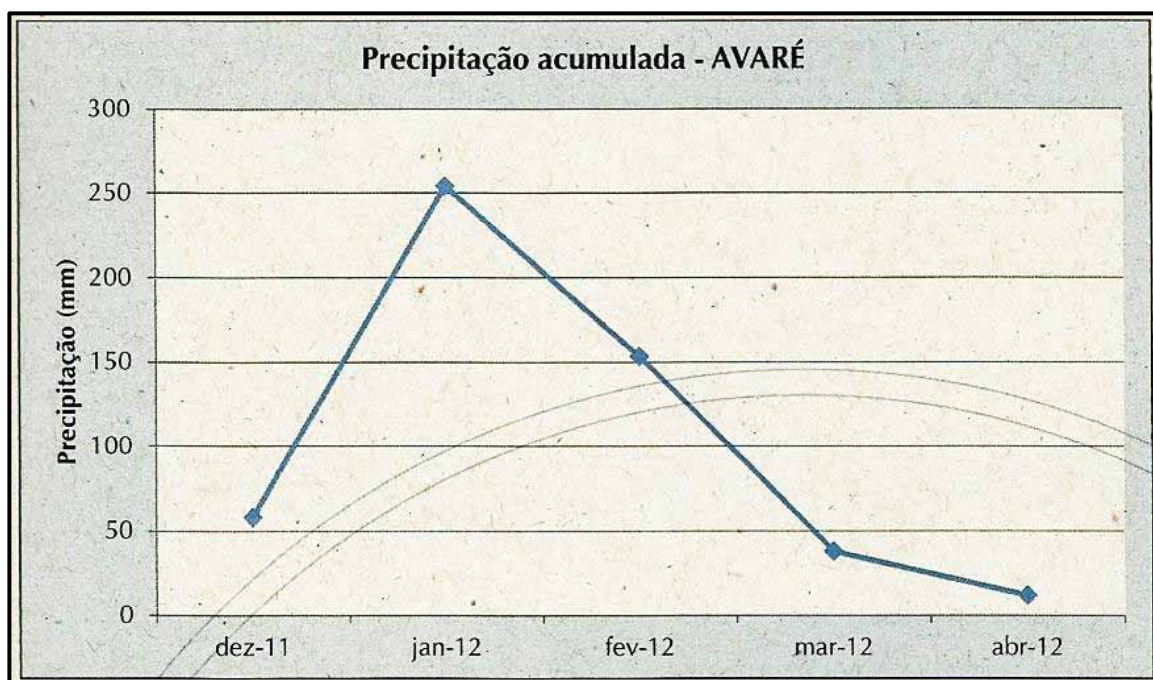
Figura 44:: Precipitação acumulada na região de Itai. Fonte: Relatório CETESB, 2012
