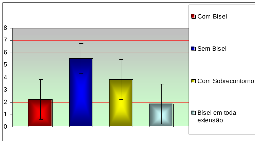
GRÁFICO 2 - Representação gráfica dos resultados médios nas diferentes técnicas de preparos cavitários empregadas e respectivo desvio padrão.
