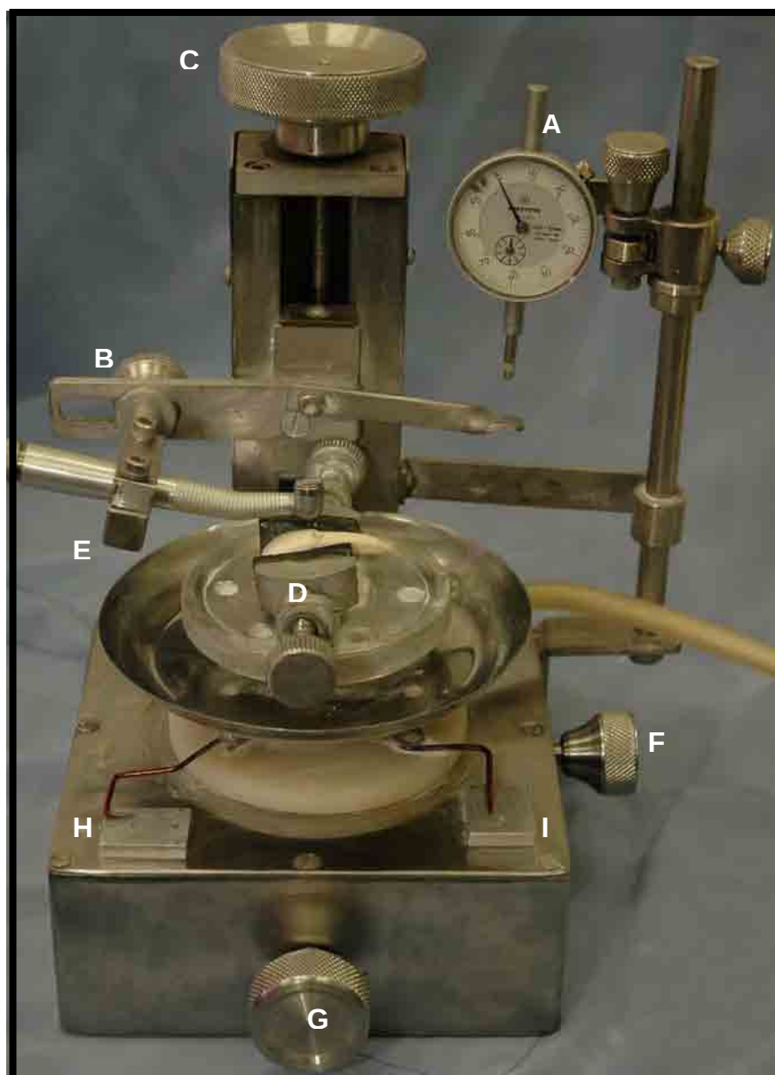
FIGURA 3- Máquina de preparo cavitário.
