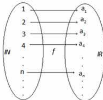
Figura 2.1.1 - Diagrama da sequência a_n .
