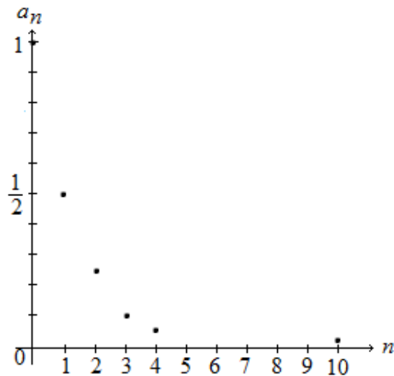
Figura 3.2.1 - Gráfico da sequência a_n .
