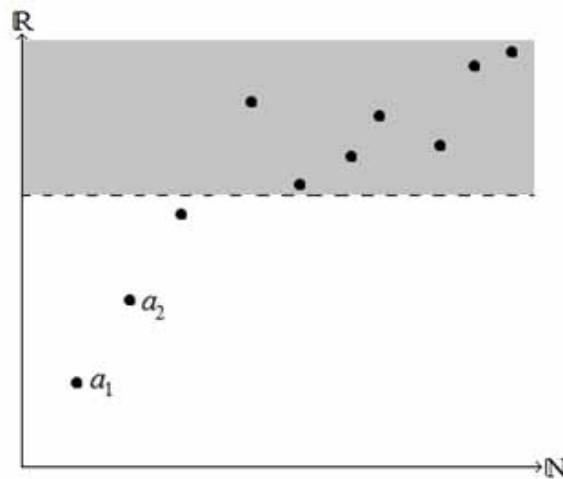
Figura 3.2.6 - A sequência (a_n) diverge para mais infinito
