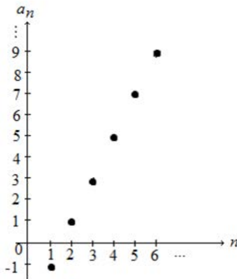
Figura 3.2.7 - Gráfico da sequência a_n .
