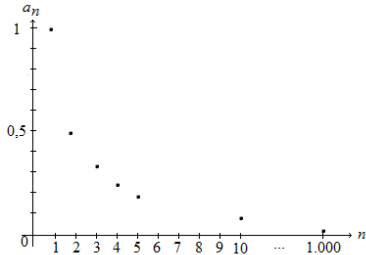
Figura 3.1.4 - Gráfico da sequência a_n .
