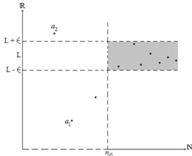
Figura 3.2.2: Gráfico da sequência convergente a_n .
