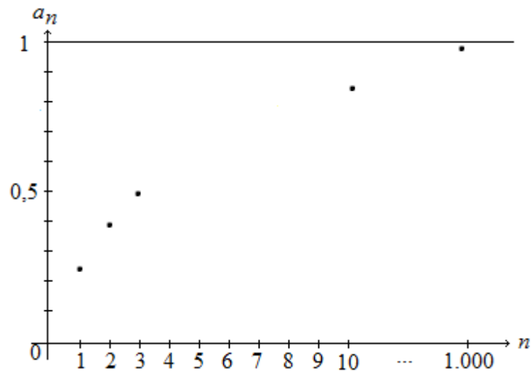
Figura 3.1.3 - Gráfico da sequência a_n .
