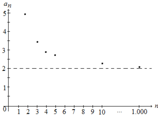
Figura 3.2.5 - Gráfico da sequência a_n .
