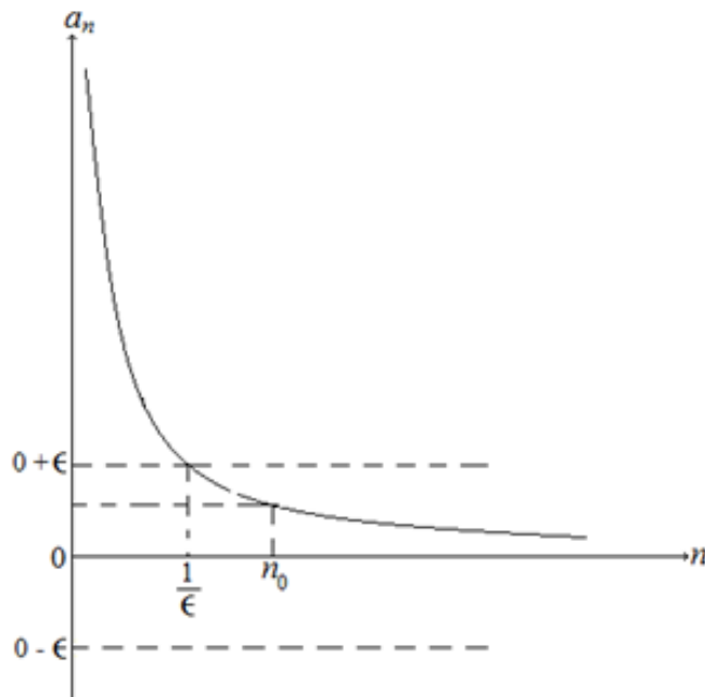
Figura 3.2.4 - Gráfico da sequência a_n
