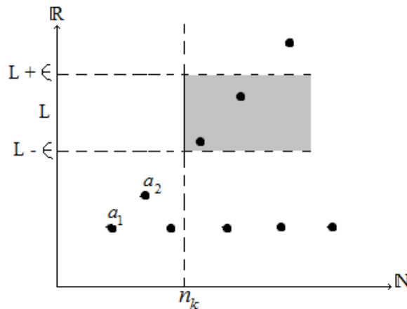
Figura 3.2.3 - Gráfico da sequência divergente a_n .
