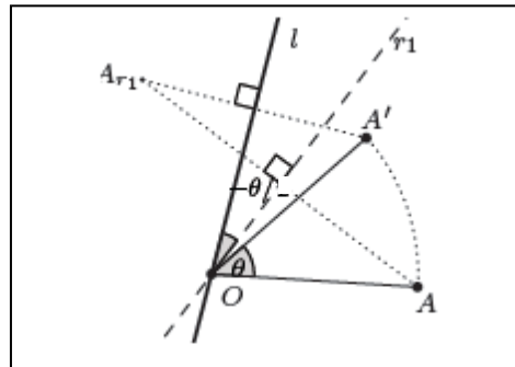
Figura 2.14: Representação de \mathcal{R}_{\theta,0} = \varphi_{l_1} \circ \varphi_{r_1} .
