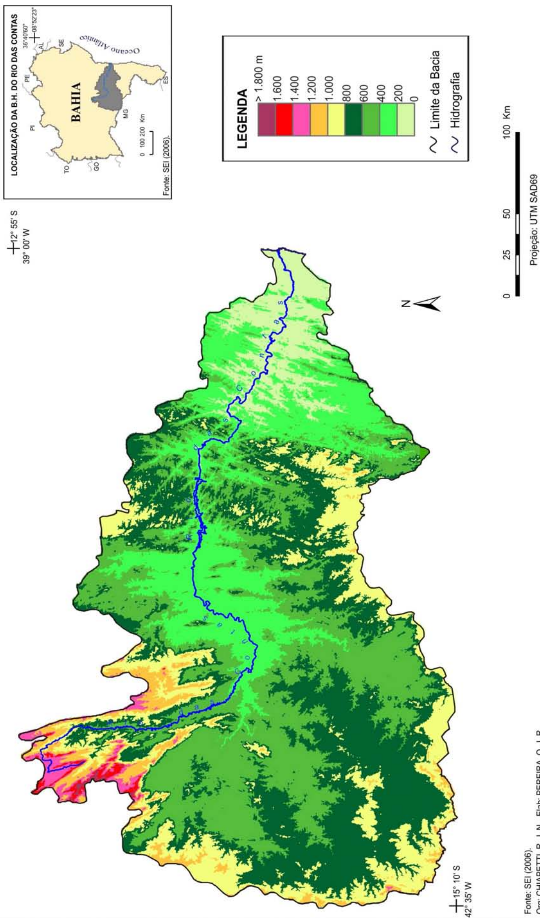
Figura 4 - Hipsometria da BH do rio das Contas, BA.
