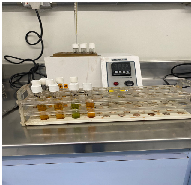
Figura 3 -Tubos de digestão durante o ensaio de Demanda Química de Oxigênio
