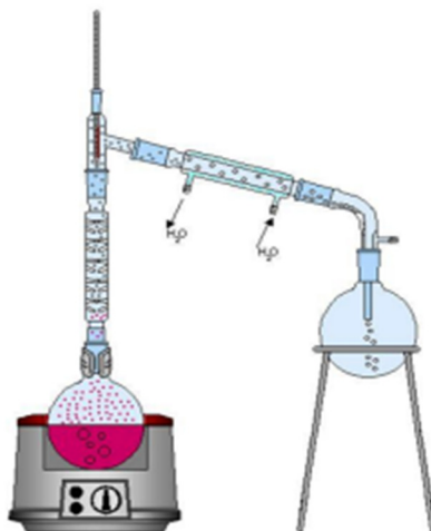
Figura 6: Sistema de destilação fracionada.
