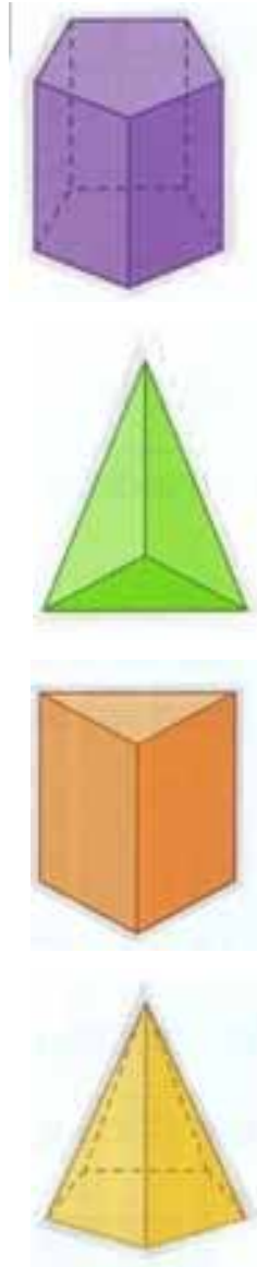
Figura 42: Poliedros para planificação.
