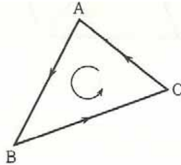
Figura 28: Triângulo orientado positivamente.
