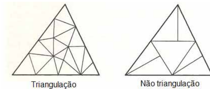
Figura 27: Decomposição triangular.
