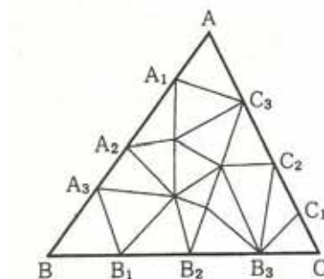
Figura 31: Triangulação do triângulo.
