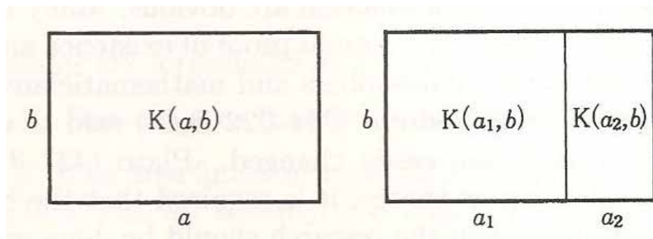
Figura 26: Retângulo e sua decomposição.
