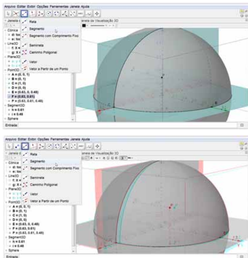
Figura 36: Definindo segmentos de reta
