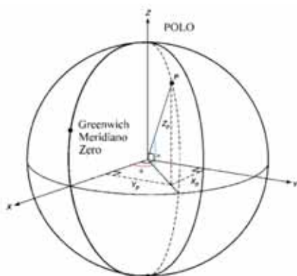
Figura 13: Representação de coordenadas geográficas
