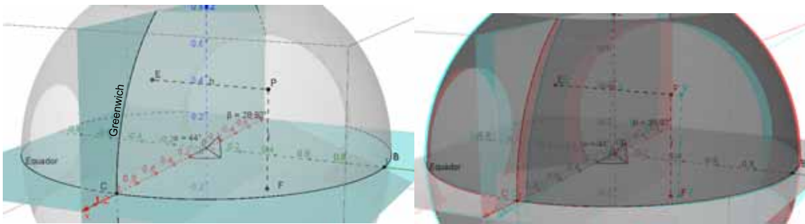
Figura 51: Ponto P sobre a superfície esférica - Latitude e Longitude
