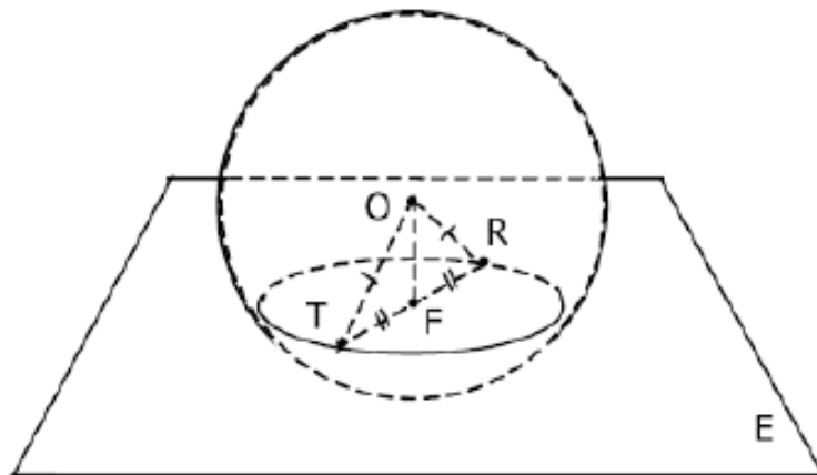
Figura 2: Superfície esférica S e plano E
