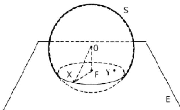
Figura 4: Plano E , secante à superfície esférica S
