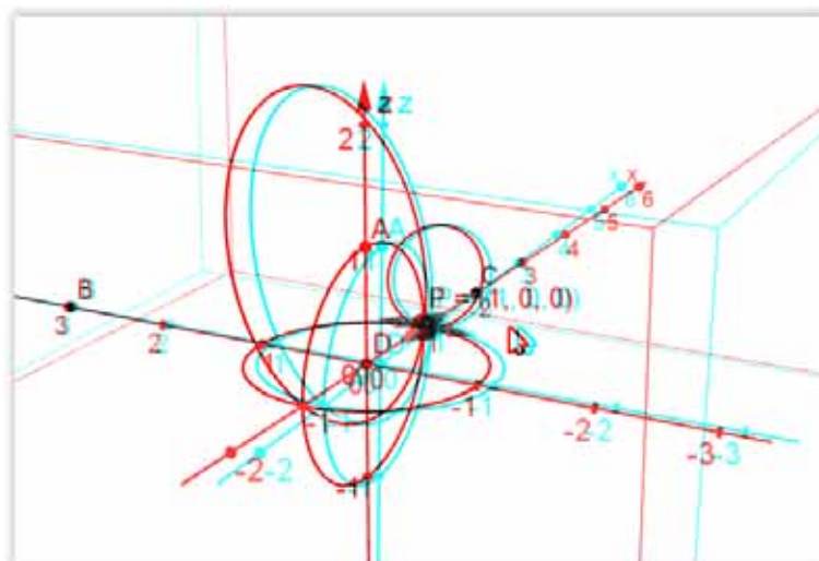
Figura 79: Intersecção das superfícies esféricas propostas no problema
