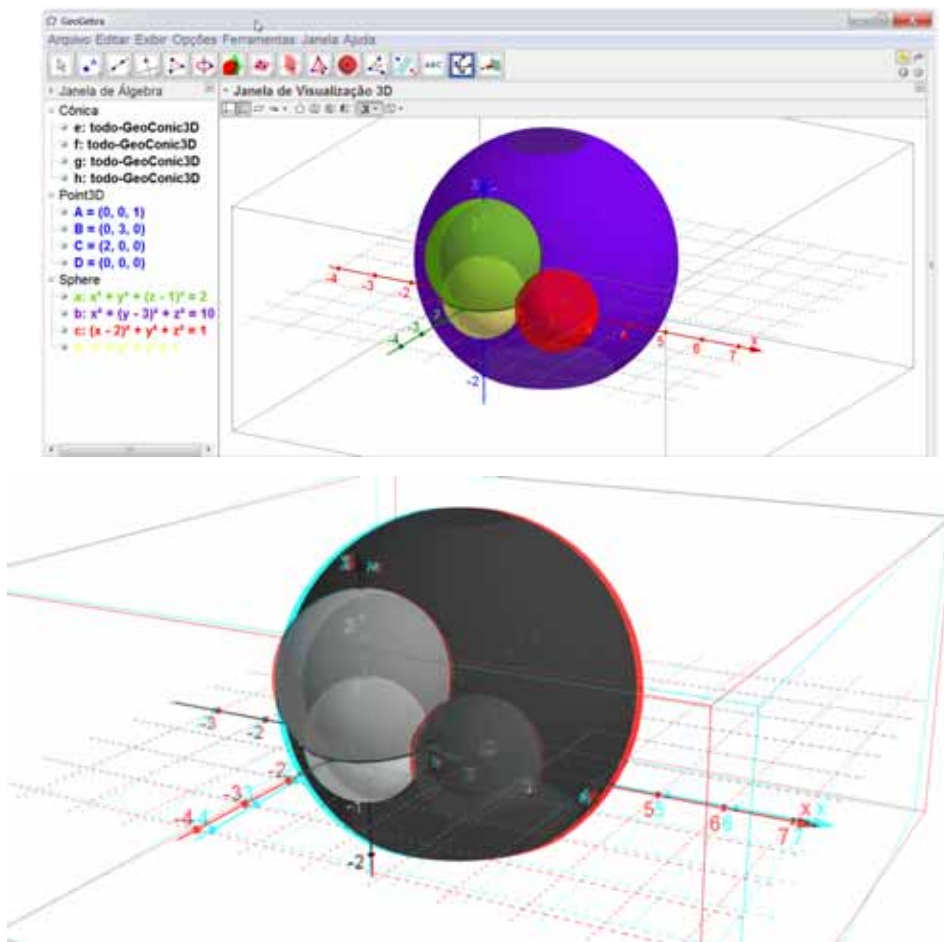
Figura 78: Modelo 3D do problema proposto
