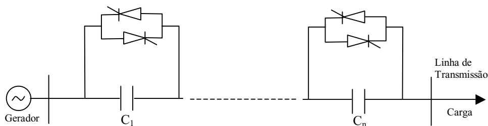
Figura 3.3. Capacitor série chaveado a tiristor.
