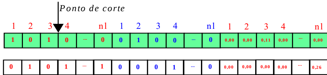
(a) Pais escolhidos
