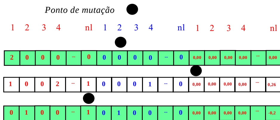
(a) Antes da mutação
