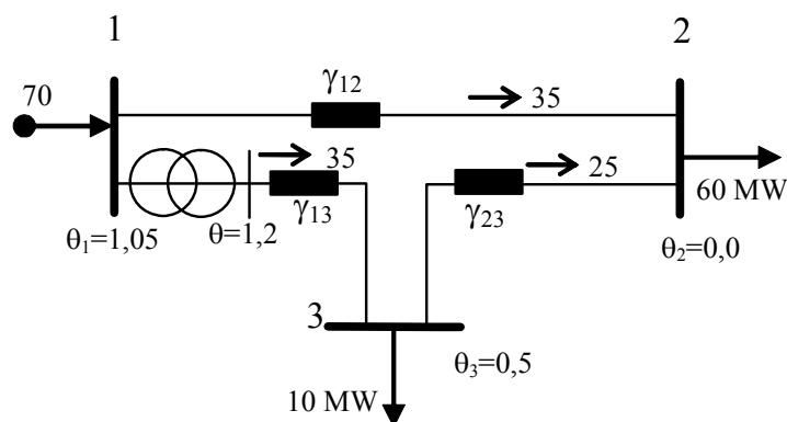
Figura 5.4: Solução do sistema com transformador defasador.
