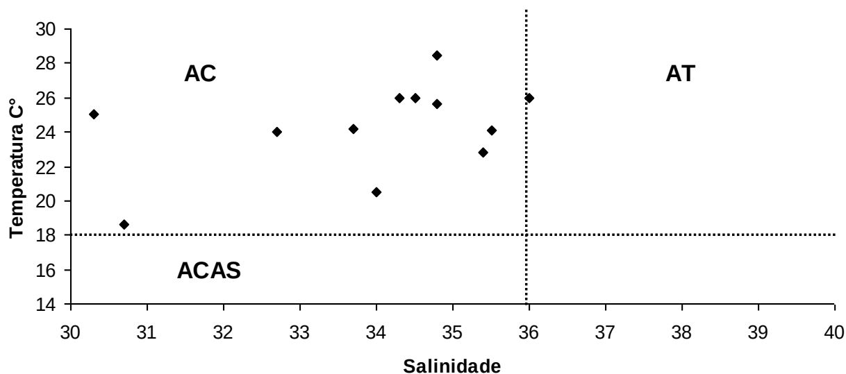
Figura 29- Diagrama T-S indicando a presença das massas de água na região de estudo durante os períodos de maio de 2002 a abril de 2003.
