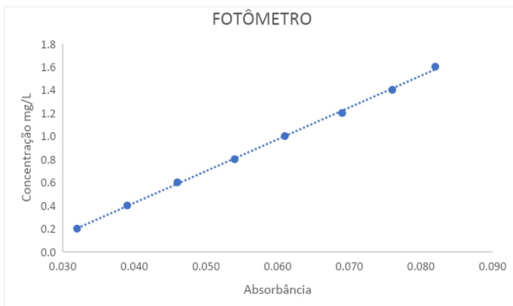
Figura 18. Curva de calibração do fotômetro (Fonte: Autor)
