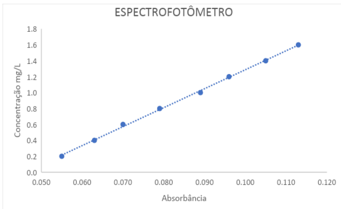
Figura 17. Curva de calibração do espectrofotômetro (Fonte: Autor)
