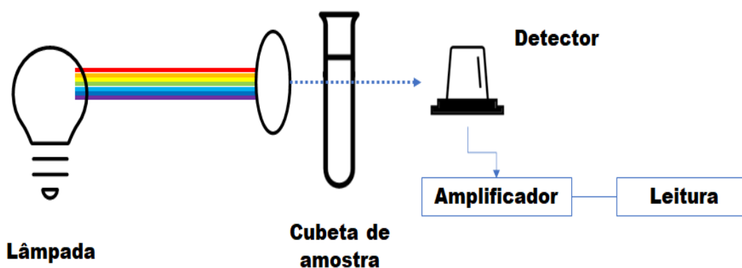
Figura 3. Esquema de um fotômetro químico (Fonte: Autor)
