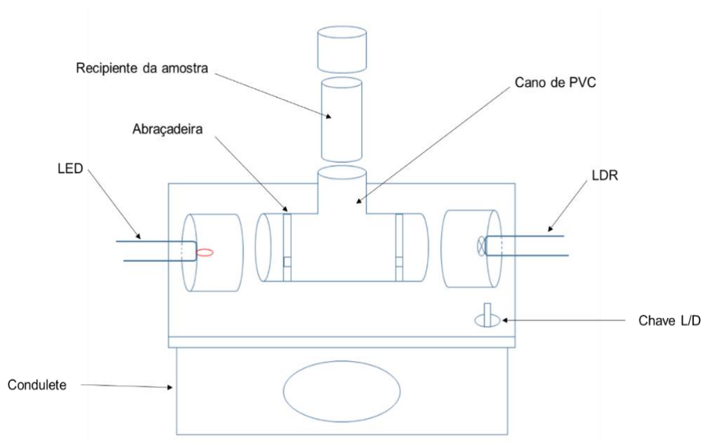
Figura 5. Esquema da montagem do fotômetro (Fonte: Autor)
