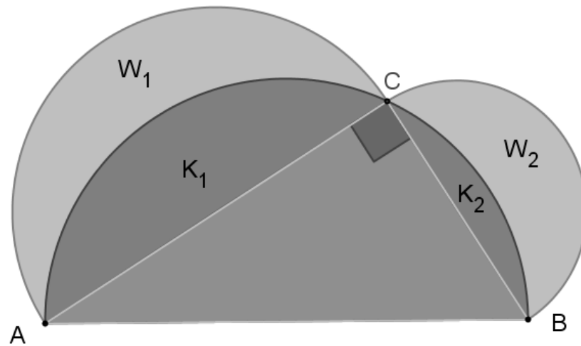
Lúnulas de Hipócrates
