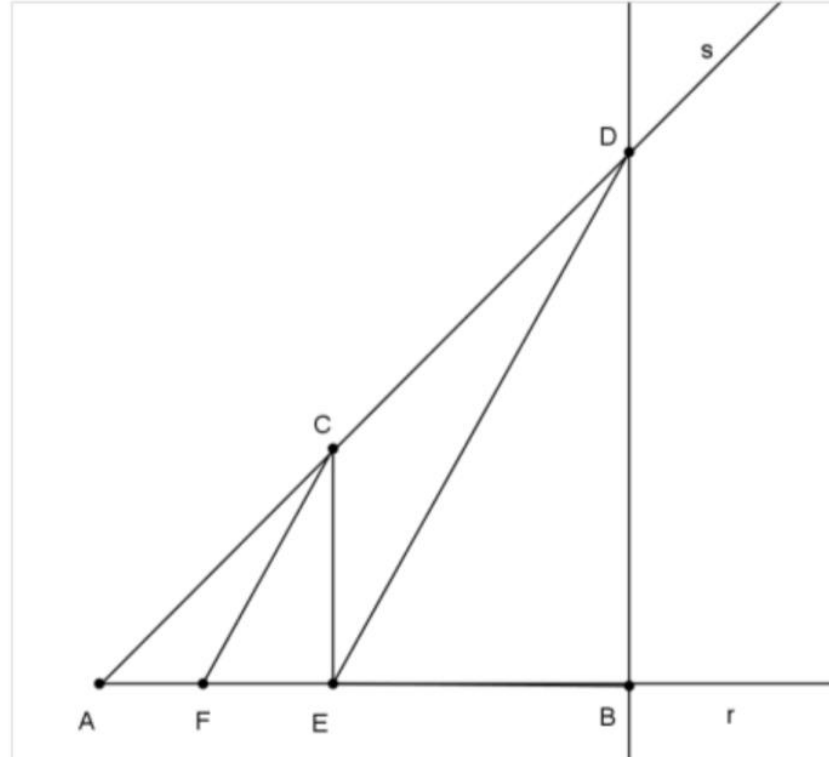
Construção de \frac{1}{a}
