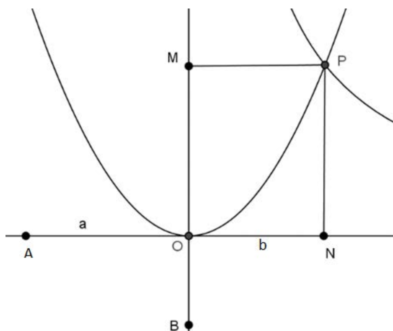
Primeira solução de Menaecmo
