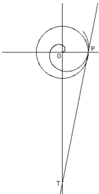
Solução de Arquimedes
