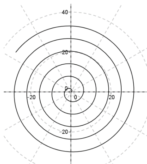
Espiral de Arquimedes com várias voltas
