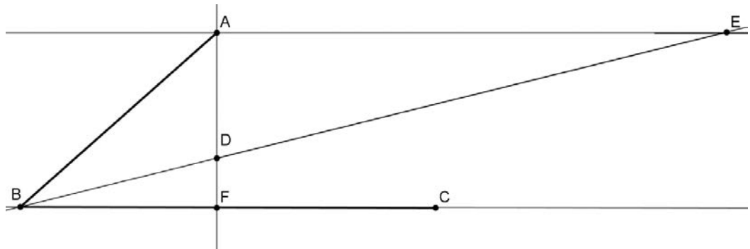
Construção, por nêusis, no software GeoGebra
