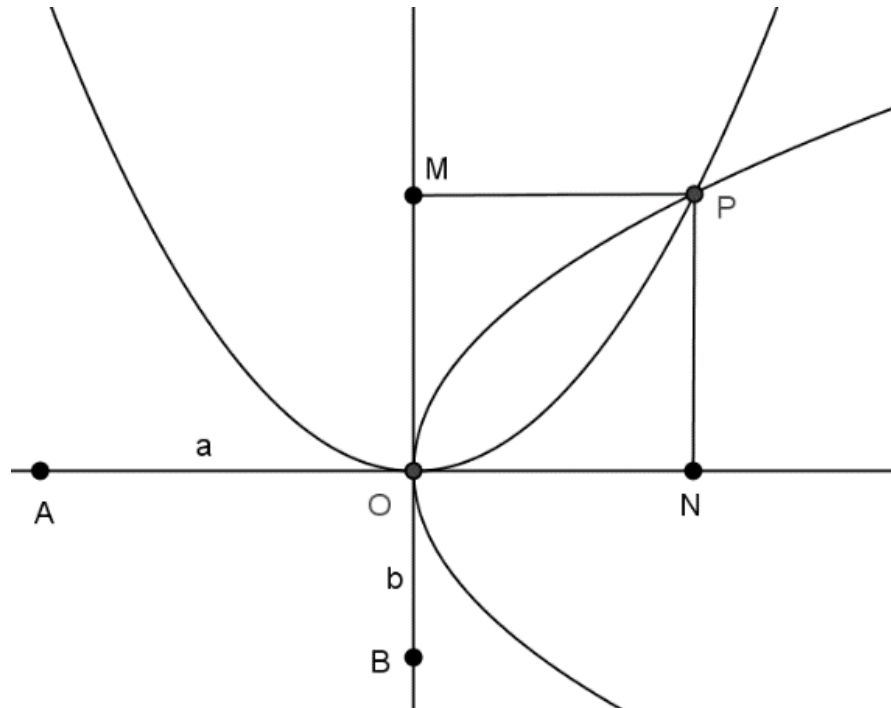
Segunda solução de Menaecmo
