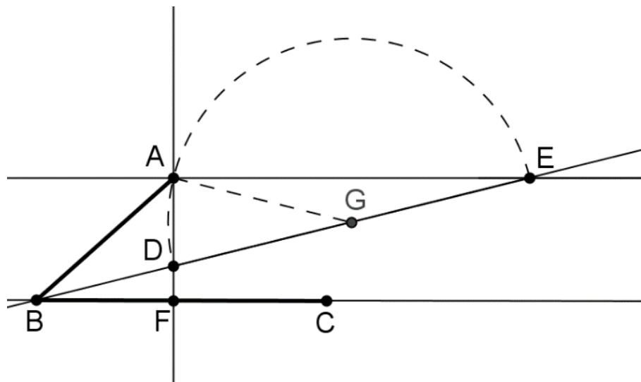
Construção, por nêusis, no software GeoGebra
