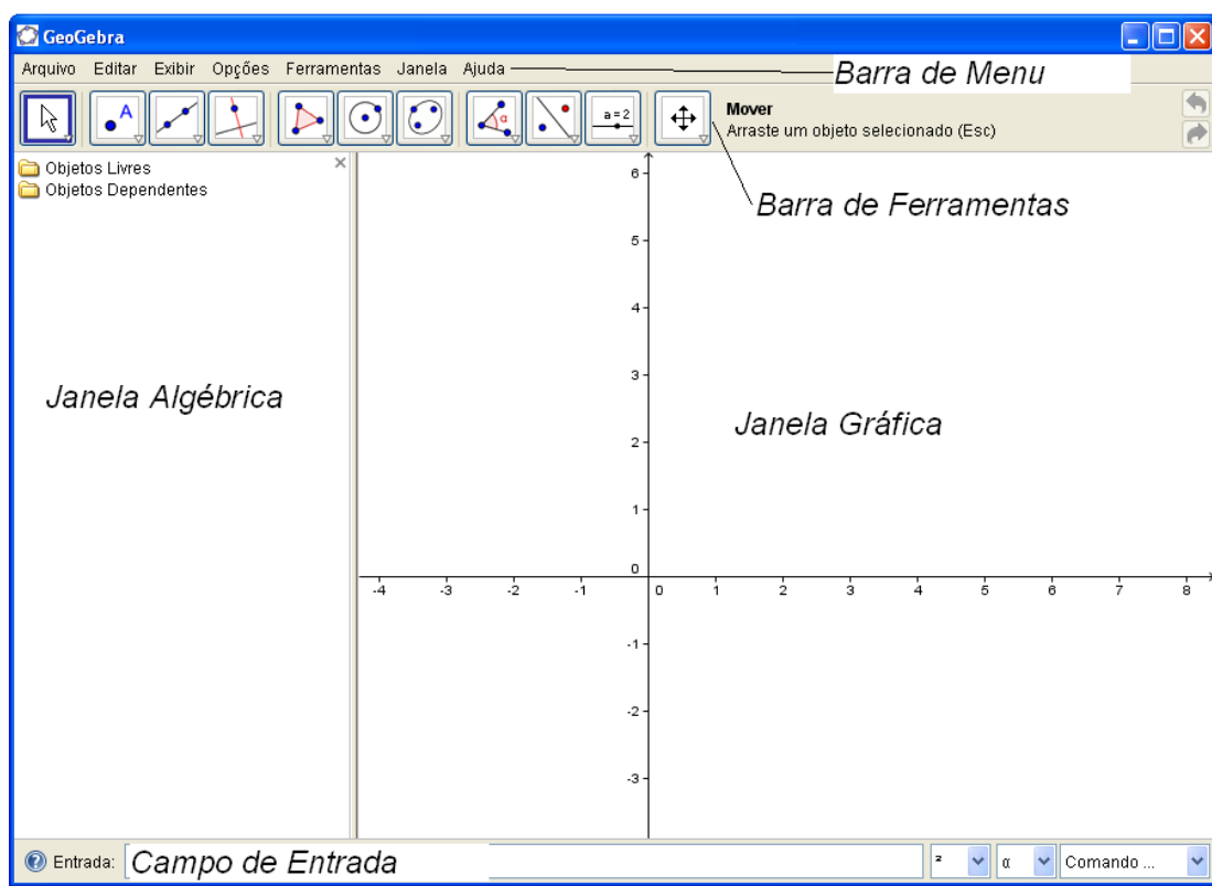
Tela inicial do geogebra
