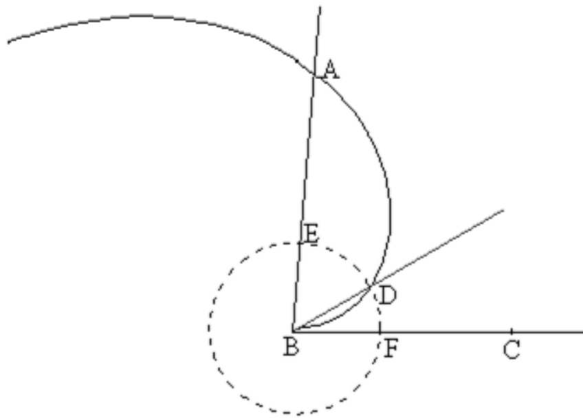
Uso da espiral de Arquimedes na trisseção de um ângulo
