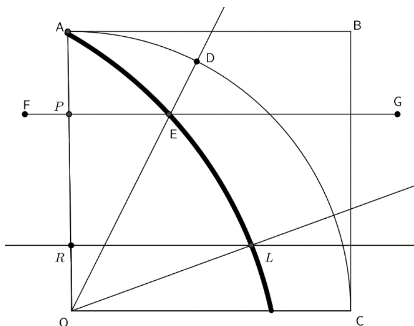
Construção da curva de Hípias (trisseção)
