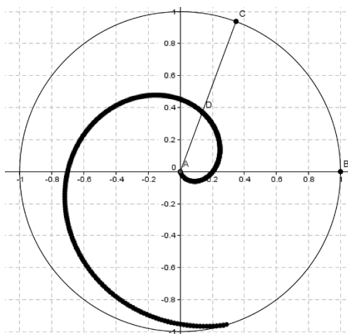
Espiral de Arquimedes com uma volta
