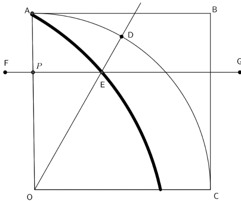
Construção da curva de Hípias
