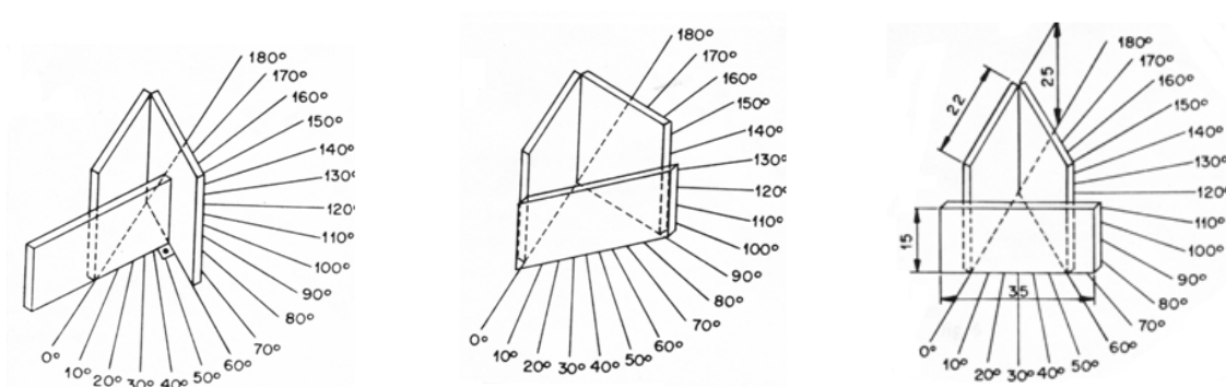
Figura 21: Estrutura dos ângulos dos caleidoscópios modificados
