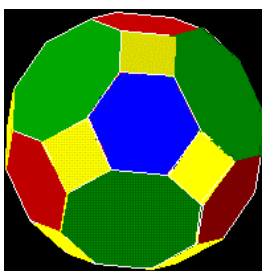
Figura 39: Sólido (4,6,8)
