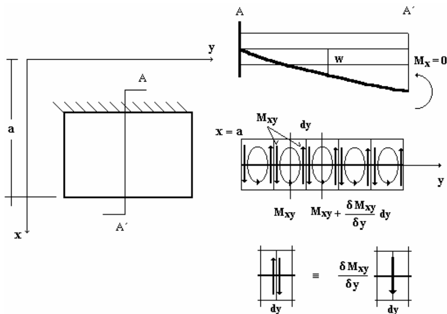
Figura 9. Borda livre (Fonte:UFRGS)
