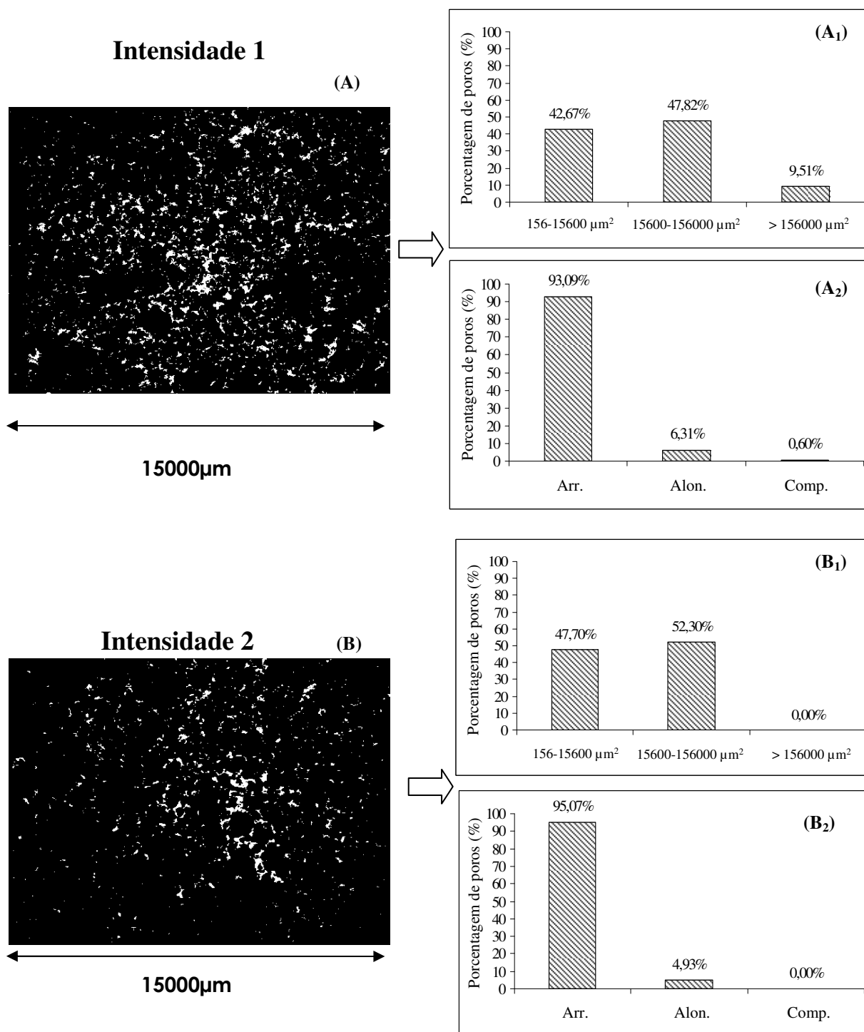
Figura 30. Imagens binarizadas (porosidade em branco e fase sólida em preto) das intensidades de compactação 1 (A) e 2 (B) no tratamento com 30 t ha -1 de BIOMIX®. Detalhamento da porosidade quanto ao tamanho (A 1 e B 1 ) e quanto a forma (A 2 e B 2 ).
