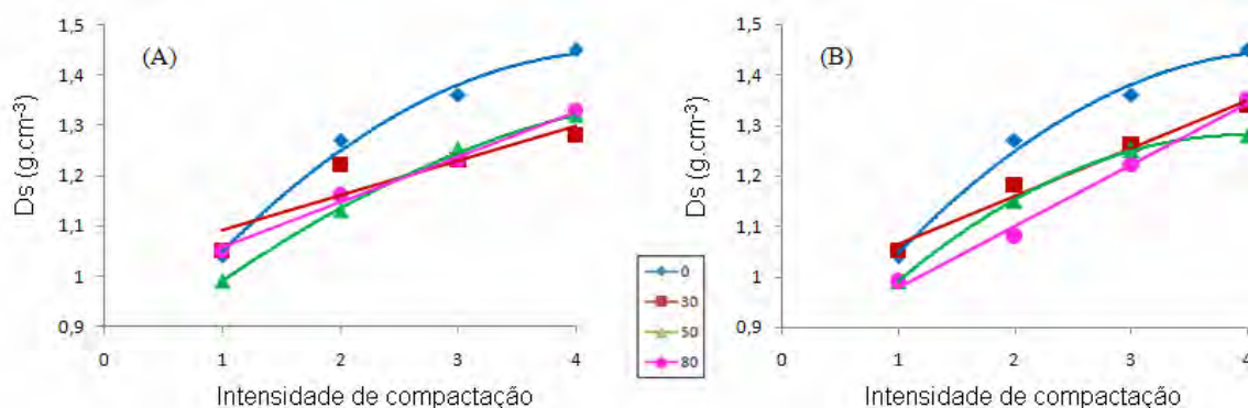
Figura 8. Variação da densidade do solo ( \text{g cm}^{-3} ), em função da intensidade de compactação, para as diferentes doses de serragem (A) e BIOMIX ® (B).
