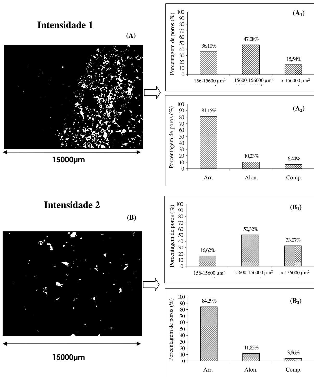
Figura 34. Imagens binarizadas (porosidade em branco e fase sólida em preto) das intensidades de compactação 1 (A) e 2 (B) no tratamento com 80 t ha -1 de BIOMIX ® . Detalhamento da porosidade quanto ao tamanho (A 1 e B 1 ) e quanto a forma (A 2 e B 2 ).
