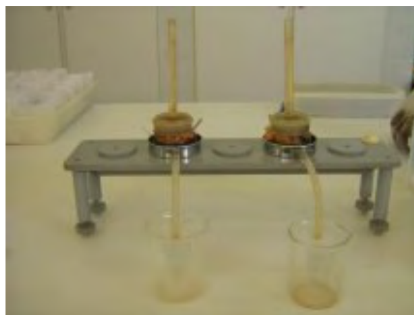
Figura 4. Permeâmetro de carga variável.
