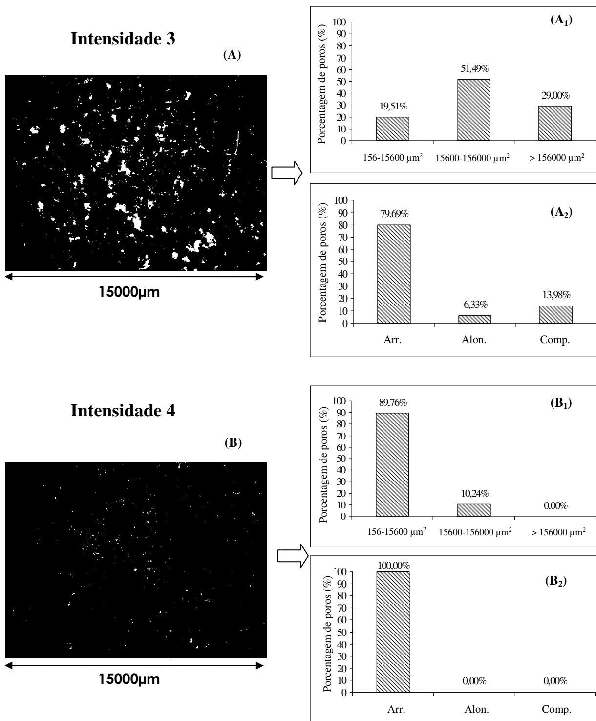
Figura 31. Imagens binarizadas (porosidade em branco e fase sólida em preto) das intensidades de compactação 3 (A) e 4 (B) no tratamento com 30 t ha -1 de BIOMIX®. Detalhamento da porosidade quanto ao tamanho (A 1 e B 1 ) e quanto a forma (A 2 e B 2 ).
