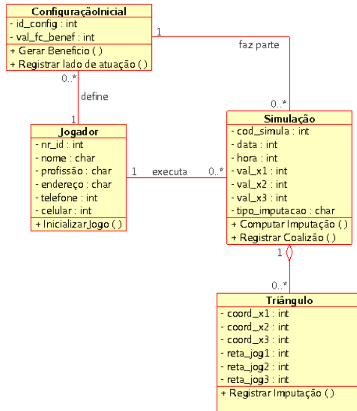
Figura 4.8: Diagrama de classes (JCE).
