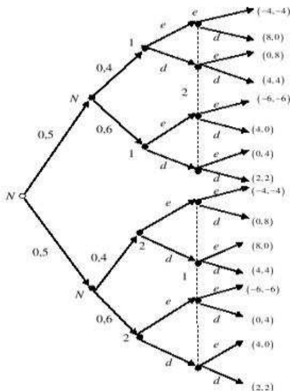
Figura 2.9: Jogo “hawk-dove” na forma extensiva.
