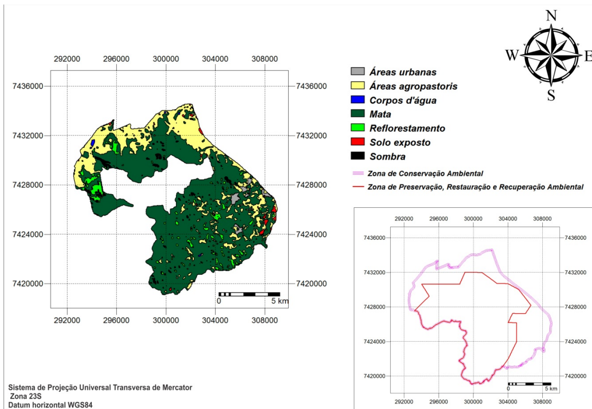
Figura 7. Cobertura do solo da Zona de Amortecimento da Reserva Biológica da Serra do Japi em 2010.
