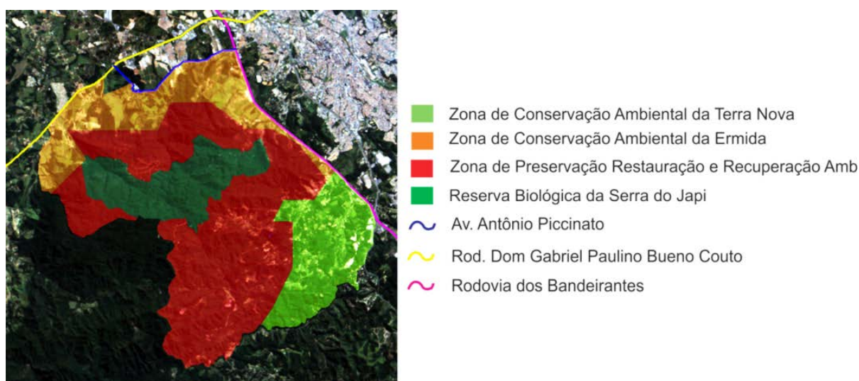
Figura 2. Divisão da Zona de Amortecimento da Reserva Biológica da Serra do Japi em 2010.
