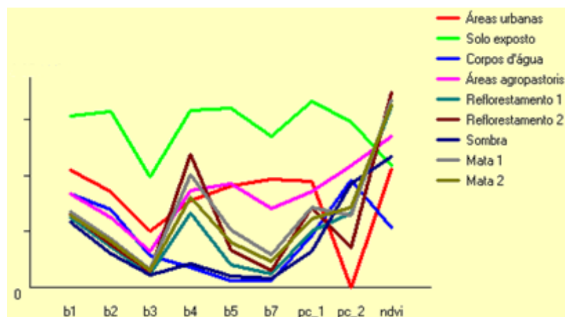
Figura 4. Assinatura espectral das amostras selecionadas para a imagem de 1989, sendo que b1, b2, b3, b4, b5 e b7 correspondem as bandas 1; 2, 3, 4, 5 e 7 respectivamente; pc_1 corresponde ao principal componente 1; e pc_2 corresponde ao principal componente 2.
