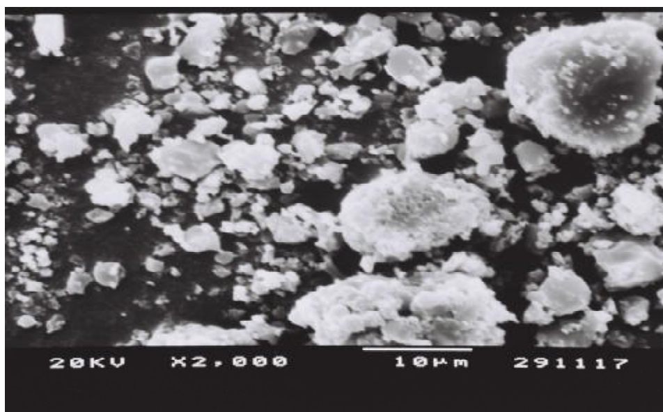
Figura 30: Microscopia eletrônica de varredura (2000X) do \text{Zn(2-MeO-BP)}_2 anidro.
