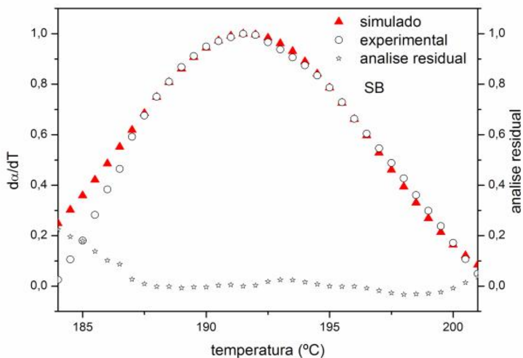
Figura 153: Curvas DTG simulada, experimental e analise residual para a decomposição do \text{Zn(2-MeO-BP)}_2 \cdot \text{H}_2\text{O} para massa de 5mg.
