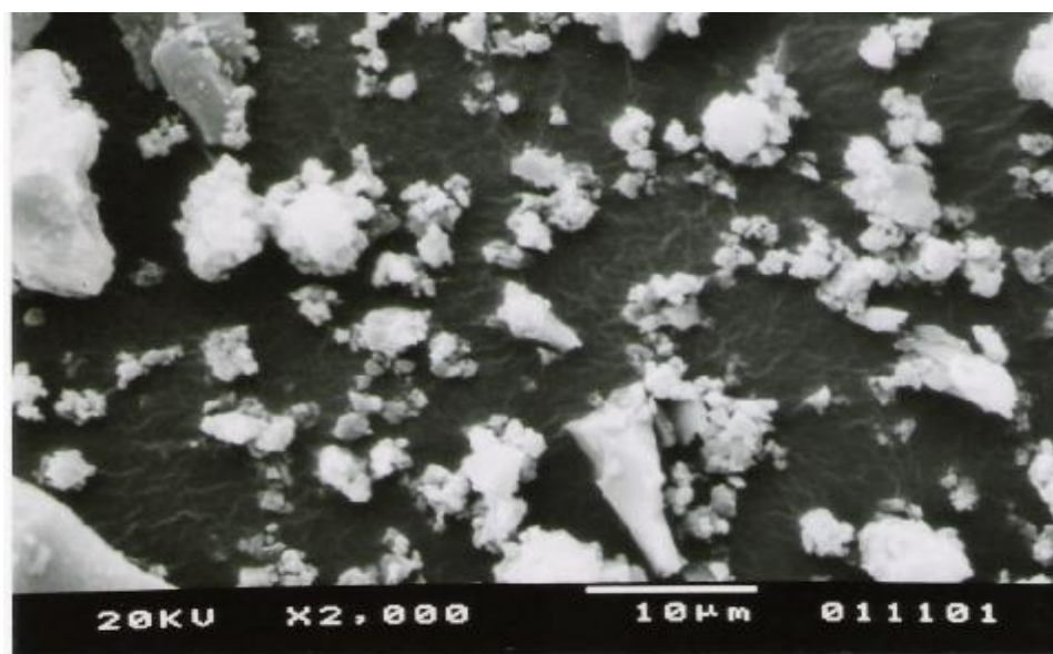
Figura 29: Microscopia eletrônica de varredura (2000X) do \text{Zn(2-MeO-BP)}_2 \cdot 2\text{H}_2\text{O} .
