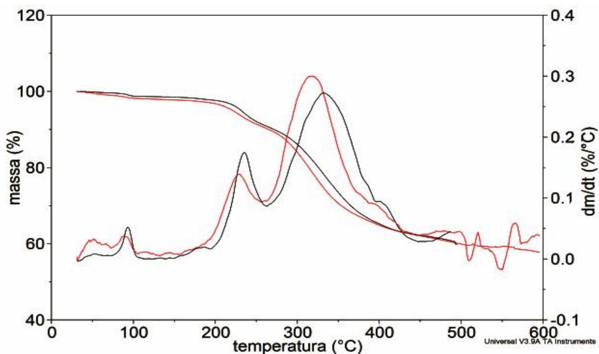
Figura 48: Curvas TG/DTG do 2-MeO-BPNa + em atmosfera de nitrogênio, razão de aquecimento de 10°C/min massa da amostra em torno de 1mg (vermelho) e 5mg (preto) em cadinho de \alpha -Al 2 O 3 .
