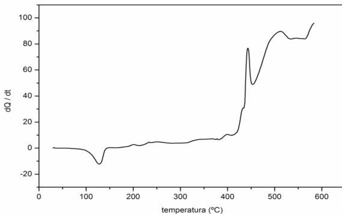
Figura 64: Curva DSC do \text{Co}(2\text{-MeO-BP}) \cdot 2,5\text{H}_2\text{O} em atmosfera de ar sintético, razão de aquecimento de 20^\circ\text{C}/\text{min} em cadinho de alumínio com tampa perfurada e massa de 3,560 mg.
