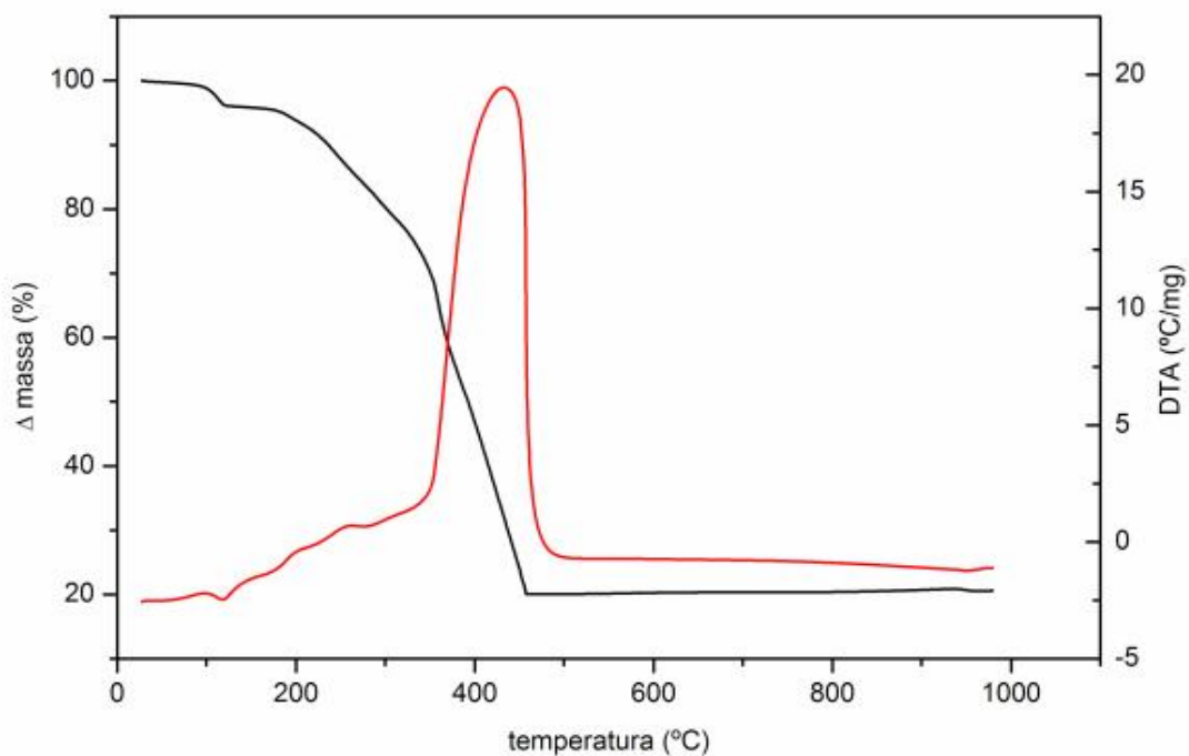
Figura 51: Curvas TG-DTA do \text{Mn}(2\text{-MeO-BP})_2 \cdot 1,5\text{H}_2\text{O} em atmosfera de ar sintético, razão de aquecimento de 20^{\circ}\text{C}/\text{min} em cadinho de \alpha\text{-Al}_2\text{O}_3 e massa de 7,410mg.
