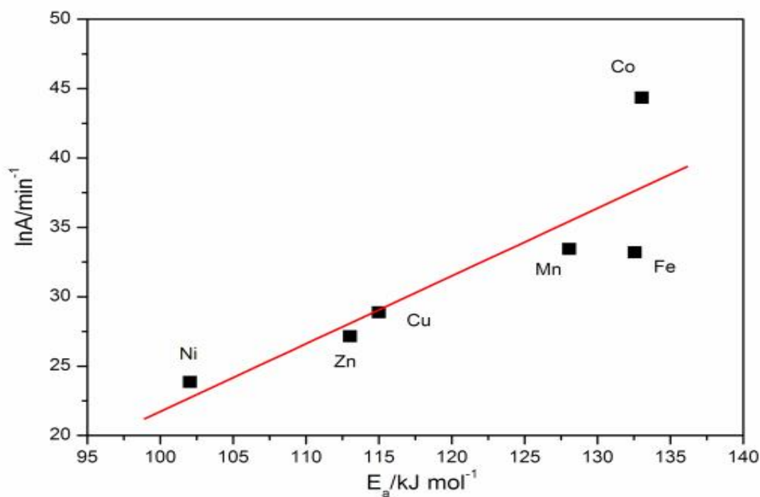
Figura 93: Dependência linear do fator pré-exponencial ( \ln A/\text{min}^{-1} ) vs energia de ativação ( E_a/\text{kJ mol}^{-1} ) para a desidratação dos compostos em alto grau de conversão ( 0.05 > \alpha < 1 ) para a massa de 5mg.
