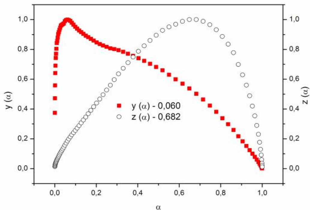
Figura 107: Funções y(\alpha) e z(\alpha) normalizadas para a obtenção de modelos cinéticos da curva TG ( 10^\circ\text{C/min} ) para a desidratação do \text{Cu}(2\text{-MeO-BP})_2 \cdot \text{H}_2\text{O} para a massa de 5 mg.
