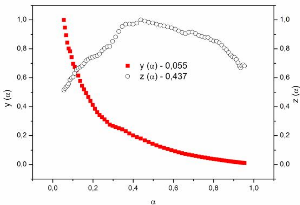
Figura 101: Funções y(\alpha) e z(\alpha) normalizadas para a obtenção de modelos cinéticos da curva TG ( 10^\circ\text{C/min} ) para a desidratação do \text{Fe}(2\text{-MeO-BP})_2 \cdot 0,5\text{H}_2\text{O} para a massa de 5mg.
