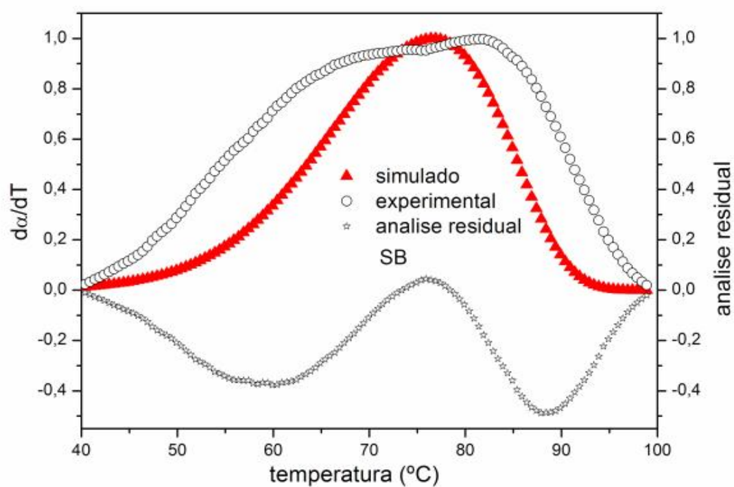
Figura 136: Curvas DTG simulada, experimental e analise residual para a desidratação do \text{Zn(2-MeO-BP)}_2 \text{H}_2\text{O} para massa de 1mg
