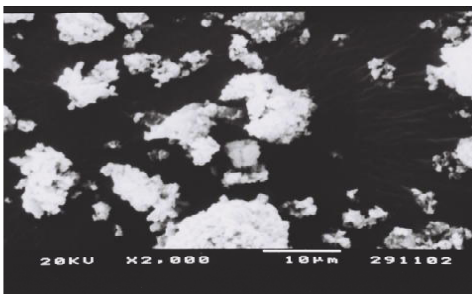
Figura 15: Microscopia eletrônica de varredura (2000X) do \text{Mn(2-MeO-BP)}_2 anidro.
