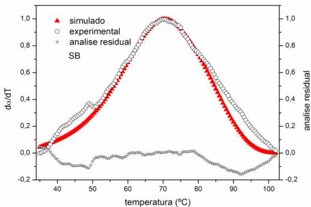
Figura 134: Curvas DTG simulada, experimental e analise residual para a desidratação do \text{Cu(2-MeO-BP)}_2 \cdot \text{H}_2\text{O} para massa de 1mg
