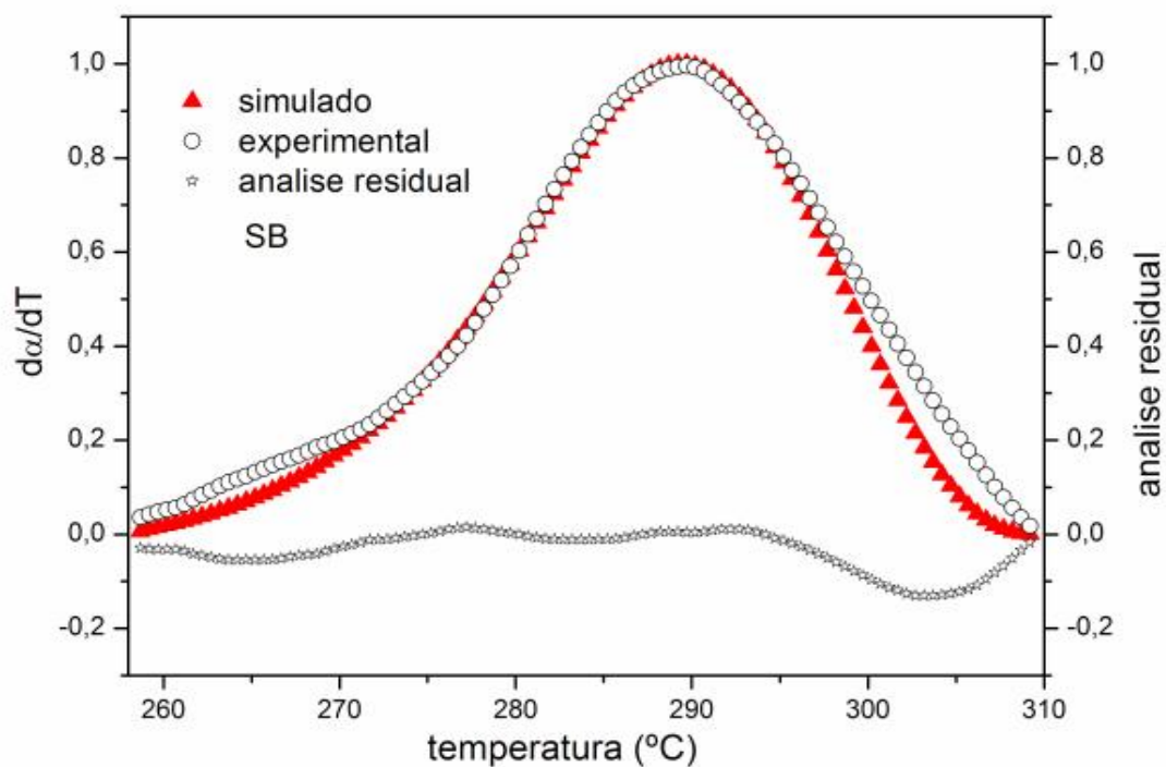
Figura 148: Curvas DTG simulada, experimental e analise residual para a decomposição do \text{Ni(2-MeO-BP)}_2 \cdot 2\text{H}_2\text{O} para massa de 1mg.
