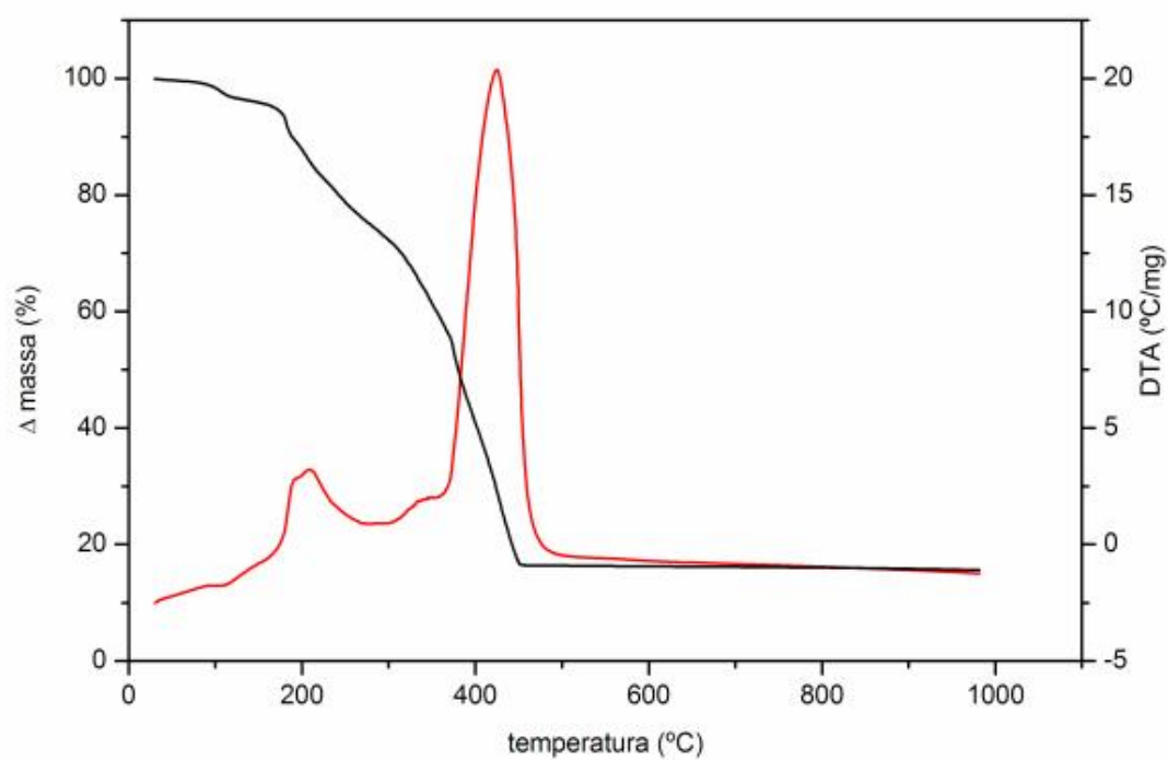
Figura 57: Curvas TG-DTA do \text{Fe(2-MeO-BP)}_2 \cdot \text{H}_2\text{O} em atmosfera de ar sintético, razão de aquecimento de 20^\circ\text{C}/\text{min} em cadinho de \alpha\text{-Al}_2\text{O}_3 e massa de 7,092 mg.
