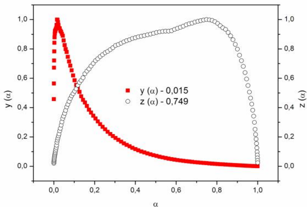
Figura 108: Funções y(\alpha) e z(\alpha) normalizadas para a obtenção de modelos cinéticos da curva TG ( 10^\circ\text{C/min} ) para a desidratação do \text{Zn}(2\text{-MeO-BP})_2 \cdot \text{H}_2\text{O} para a massa de 1mg.
