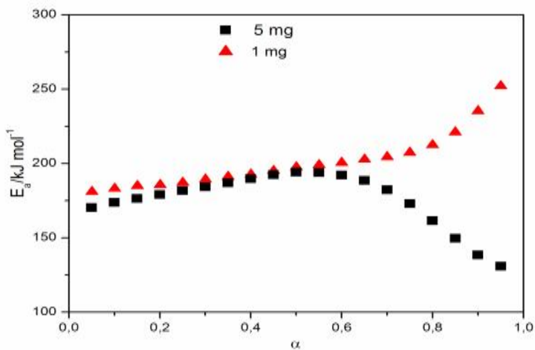
Figura 67: Variação da energia de ativação ( E_a/\text{kJ mol}^{-1} ) vs grau de conversão ( \alpha ) da decomposição do \text{Co(2-MeO-BP)}_2 para as massa de 1 e 5mg.
