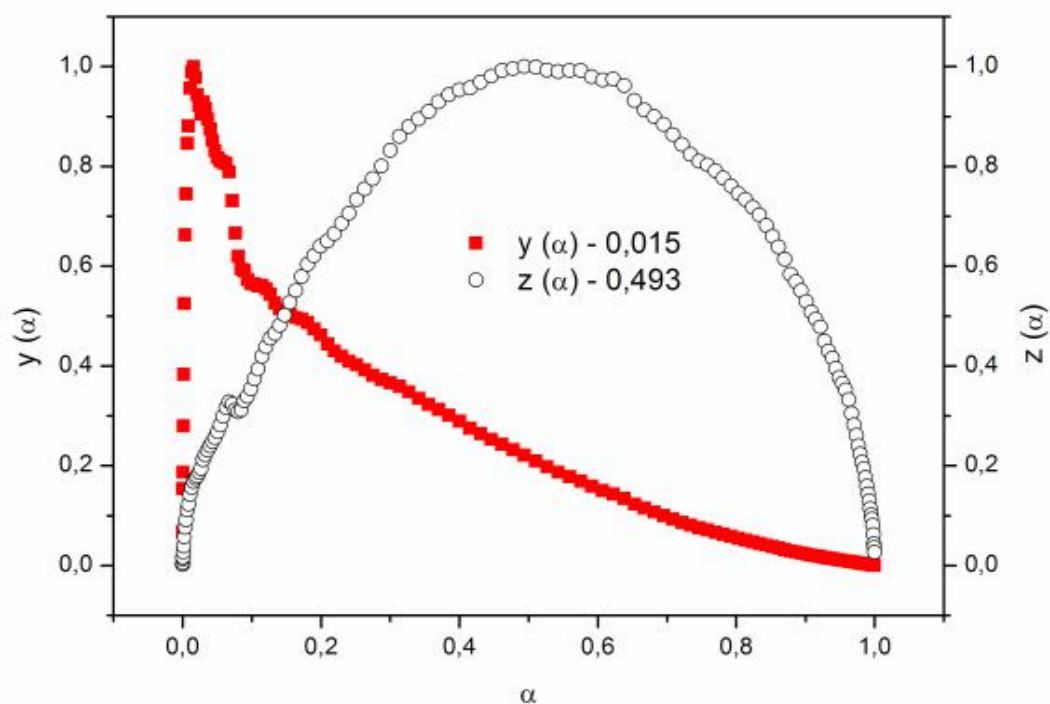
Figura 106: Funções y(\alpha) e z(\alpha) normalizadas para a obtenção de modelos cinéticos da curva TG ( 10^\circ\text{C/min} ) para a desidratação do \text{Cu}(2\text{-MeO-BP})_2 \cdot \text{H}_2\text{O} para a massa de 1 mg.
