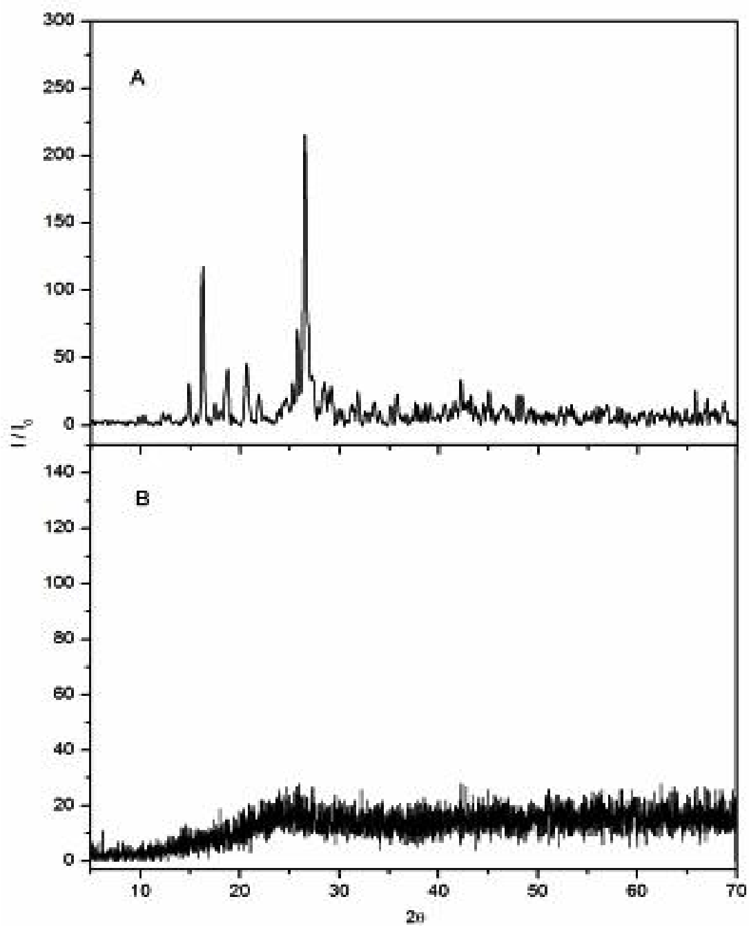
Figura 22: Difratograma de raios X do \text{Co}(2\text{-MeO-BP})_2 : (A) complexo hidratado e (B) complexo anidro.
