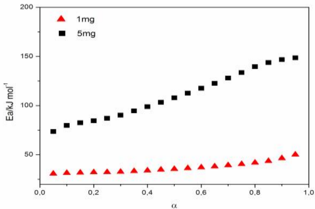
Figura 60: Variação da energia de ativação ( E_a/\text{kJ mol}^{-1} ) vs grau de conversão ( \alpha ) da desidratação do \text{Fe(2-MeO-BP)}_2 \cdot 0,65\text{H}_2\text{O} para as massa de 1 e 5mg.
