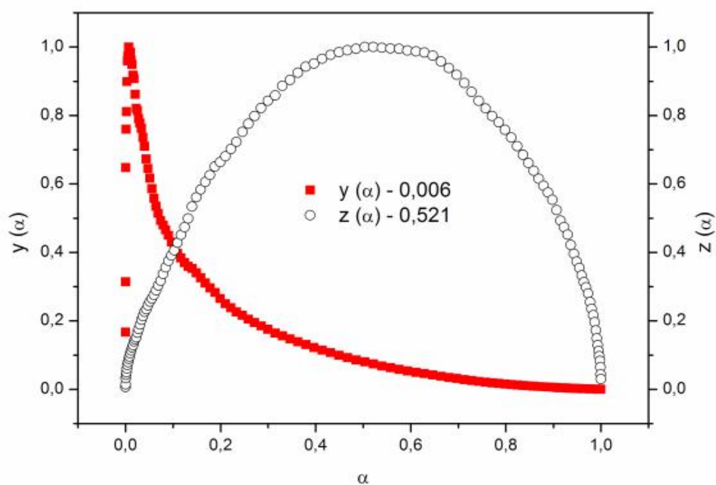
Figura 104: Funções y(\alpha) e z(\alpha) normalizadas para a obtenção de modelos cinéticos da curva TG ( 10^\circ\text{C/min} ) para a desidratação do \text{Ni(2-MeO-BP)}_2 \cdot 2\text{H}_2\text{O} para a massa de 1mg.
