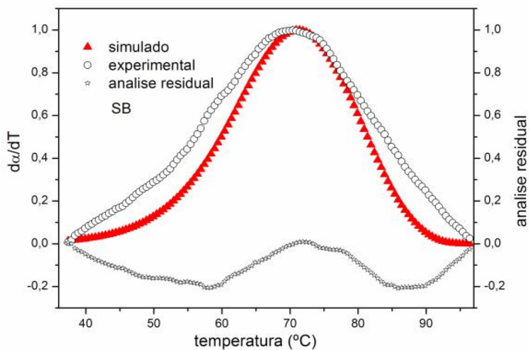
Figura 132: Curvas DTG simulada, experimental e analise residual para a desidratação do \text{Ni(2-MeO-BP)}_2 \cdot 2\text{H}_2\text{O} para massa de 1mg
