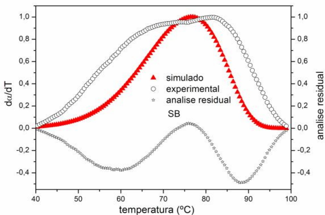
Figura 152: Curvas DTG simulada, experimental e analise residual para a decomposição do \text{Zn(2-MeO-BP)}_2 \cdot \text{H}_2\text{O} para massa de 1mg.
