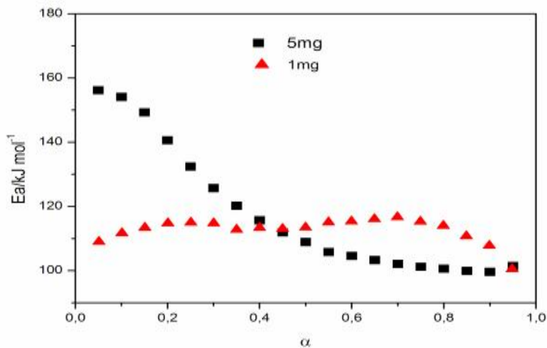
Figura 72: Variação da energia de ativação ( E_a/\text{kJ mol}^{-1} ) vs grau de conversão ( \alpha ) da desidratação do \text{Ni(2-MeO-BP)}_2 \cdot 1,65\text{H}_2\text{O} para as massa de 1 e 5mg.
