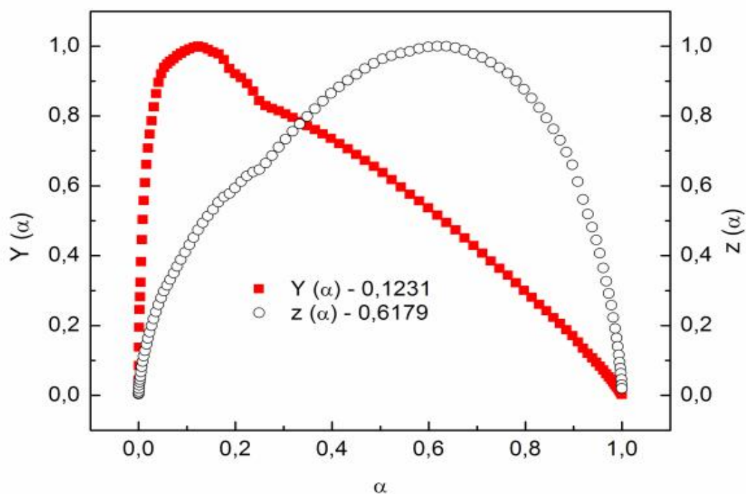
Figura 116: Funções y(\alpha) e z(\alpha) normalizadas para a obtenção de modelos cinéticos da curva TG ( 10^\circ\text{C/min} ) para a decomposição do \text{Fe}(2\text{-MeO-BP})_2 para a massa de 1mg.
