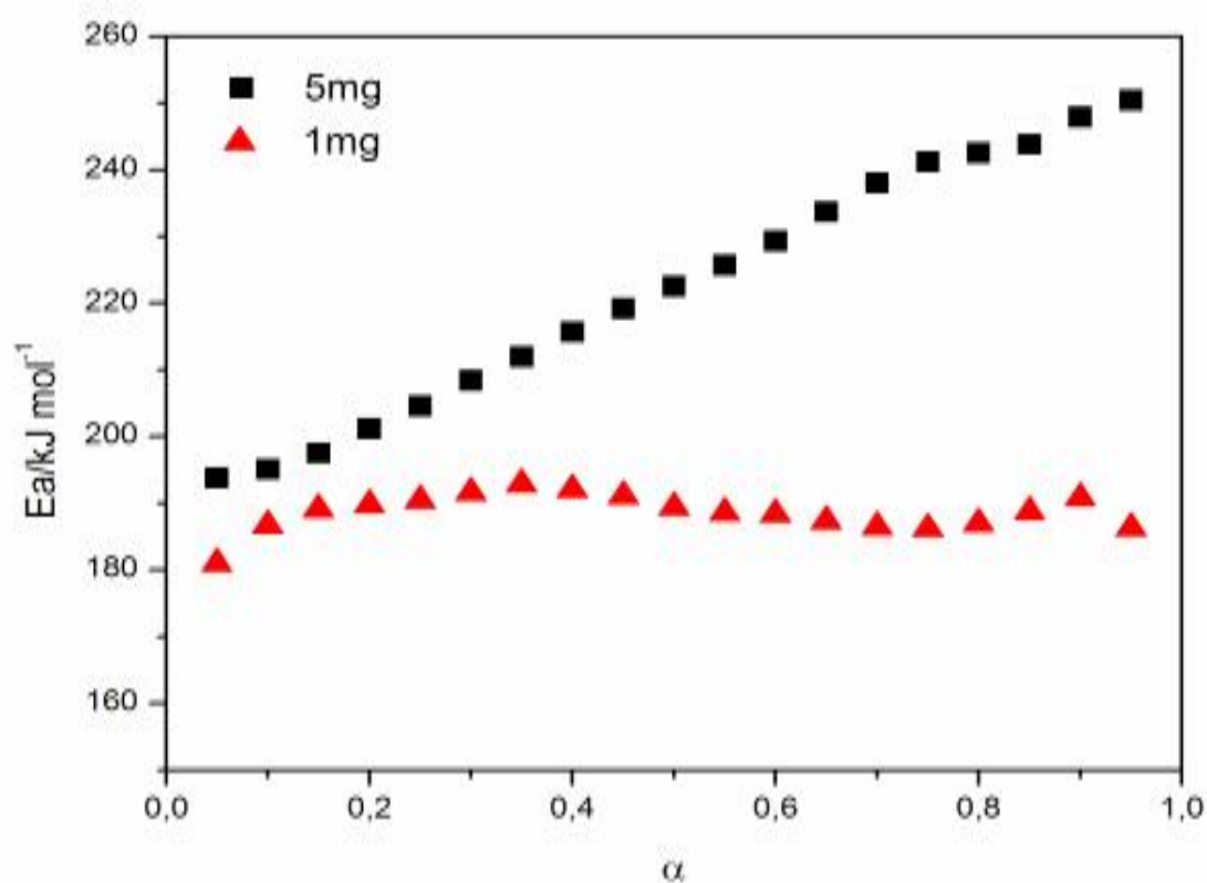
Figura 55: Variação da energia de ativação ( E_a/\text{kJ mol}^{-1} ) vs grau de conversão ( \alpha ) da decomposição do \text{Mn(2-MeO-BP)}_2 para as massa de 1 e 5mg.
