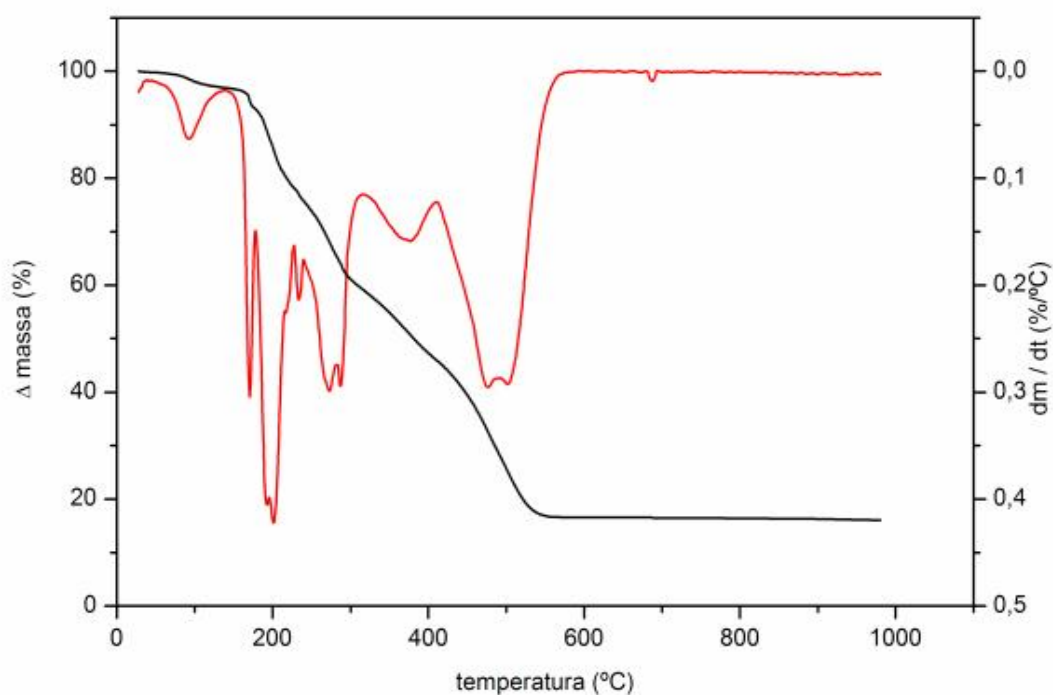
Figura 74: Curvas TG/DTG do \text{Cu(2-MeO-BP)}_2 \cdot \text{H}_2\text{O} em atmosfera de ar sintético, razão de aquecimento de 20^\circ\text{C}/\text{min} em cadinho de \alpha\text{-Al}_2\text{O}_3 e massa de 7,060 mg.
