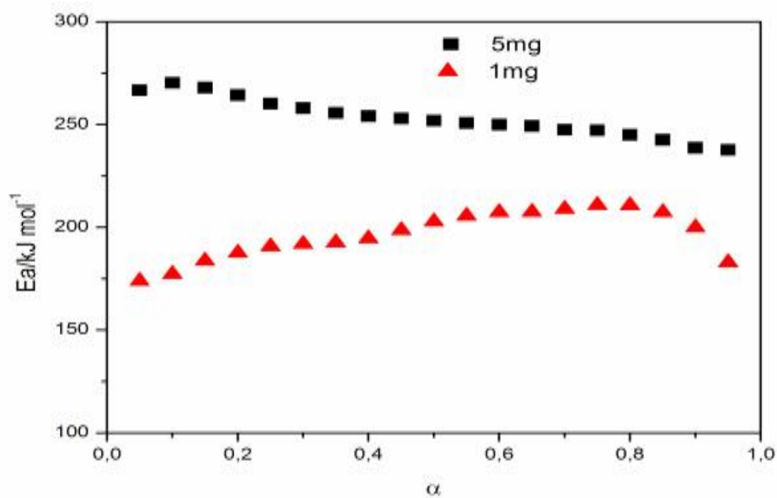
Figura 61: Variação da energia de ativação ( E_a/\text{kJ mol}^{-1} ) vs grau de conversão ( \alpha ) da decomposição do \text{Fe(2-MeO-BP)}_2 para as massa de 1 e 5mg.
