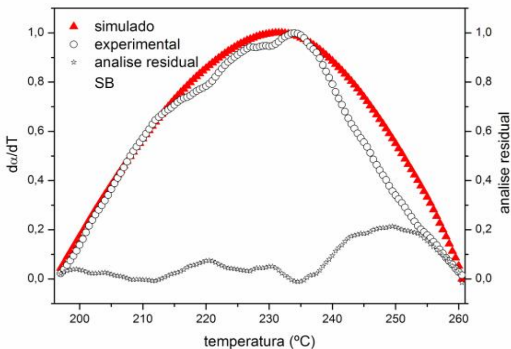
Figura 143: Curvas DTG simulada, experimental e analise residual para a decomposição do \text{Mn}(2\text{-MeO-BP})_2 \cdot \text{H}_2\text{O} para massa de 5mg.
