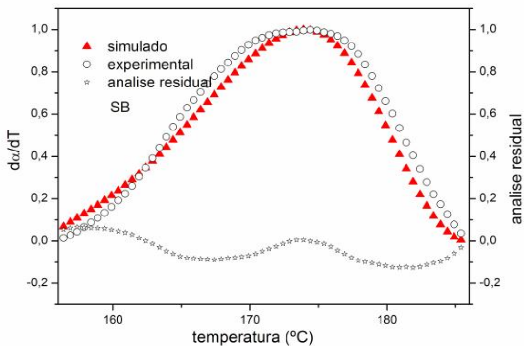
Figura 150: Curvas DTG simulada, experimental e análise residual para a decomposição do \text{Cu}(2\text{-MeO-BP})_2 \text{H}_2\text{O} para massa de 1mg.
