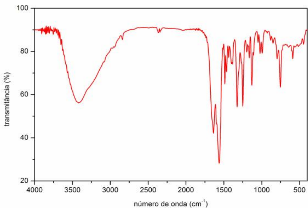
Figura 37: Espectro de absorção na região do infravermelho (FTIR) do \text{Ni}(\text{2-MeO-BP})_2 \cdot 2\text{H}_2\text{O} .
