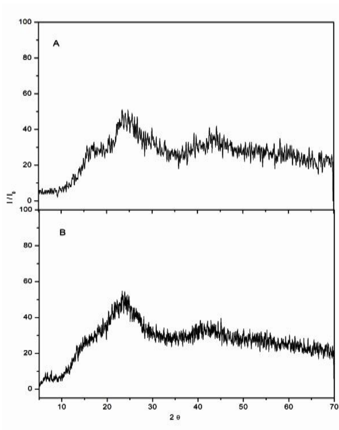
Figura 31: Difratoograma de raios X do \text{Zn}(\text{2-MeO-BP})_2 : (A) complexo hidratado e (B) complexo anidro.
