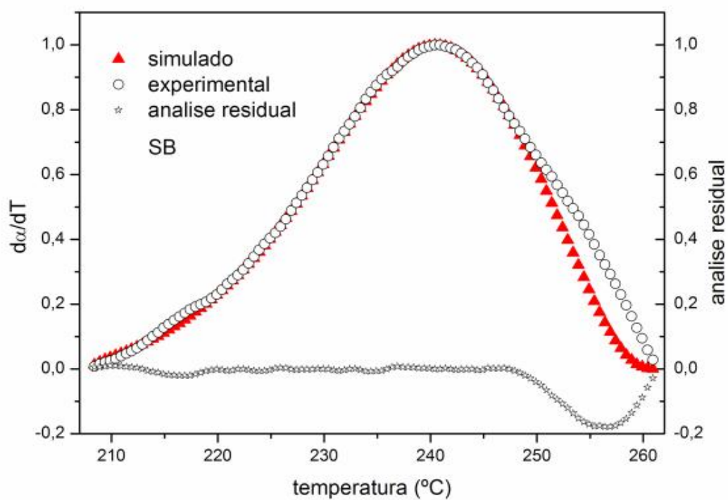
Figura 147: Curvas DTG simulada, experimental e analise residual para a decomposição do \text{Co}(2\text{-MeO-BP})_2 \text{H}_2\text{O} para massa de 5mg.
