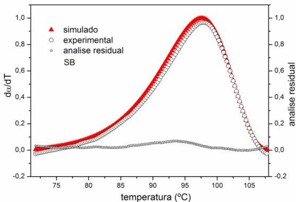
Figura 126: Curvas DTG simulada, experimental e analise residual para a desidratação do \text{Mn}(2\text{-MeO-BP})_2 \text{H}_2\text{O} para massa de 1mg.
