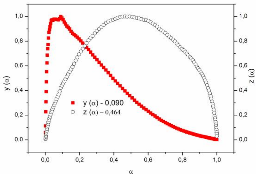
Figura 118: Funções y(\alpha) e z(\alpha) normalizadas para a obtenção de modelos cinéticos da curva TG (10°C/min) para a decomposição do \text{Co(2-MeO-BP)}_2 para a massa de 1mg.
