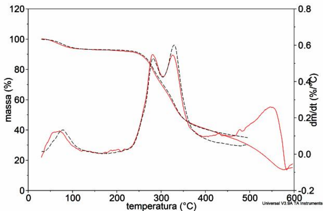
Figura 71: Curvas TG/DTG do \text{Ni(2-MeO-BP)}_2 \cdot 1,65\text{H}_2\text{O} em atmosfera de nitrogênio, razão de aquecimento de 10^\circ\text{C/min} , massa da amostra em torno de 1mg (vermelho) e 5mg (preto) em cadinho de \alpha\text{-Al}_2\text{O}_3 .
