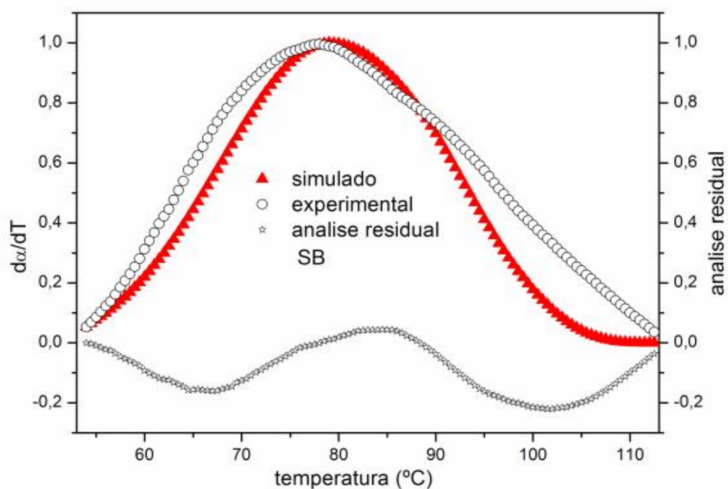
Figura 133: Curvas DTG simulada, experimental e analise residual para a desidratação do \text{Ni(2-MeO-BP)}_2 \cdot 2\text{H}_2\text{O} para massa de 5mg
