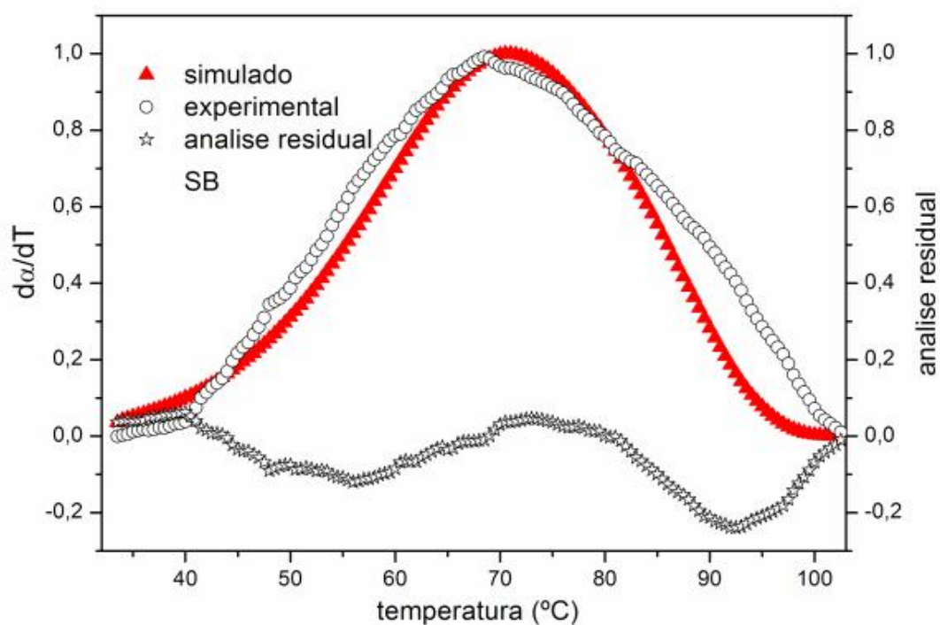
Figura 128: Curvas DTG simulada, experimental e analise residual para a desidratação do \text{Fe(2-MeO-BP)}_2 \cdot \text{H}_2\text{O} para massa de 1mg.
