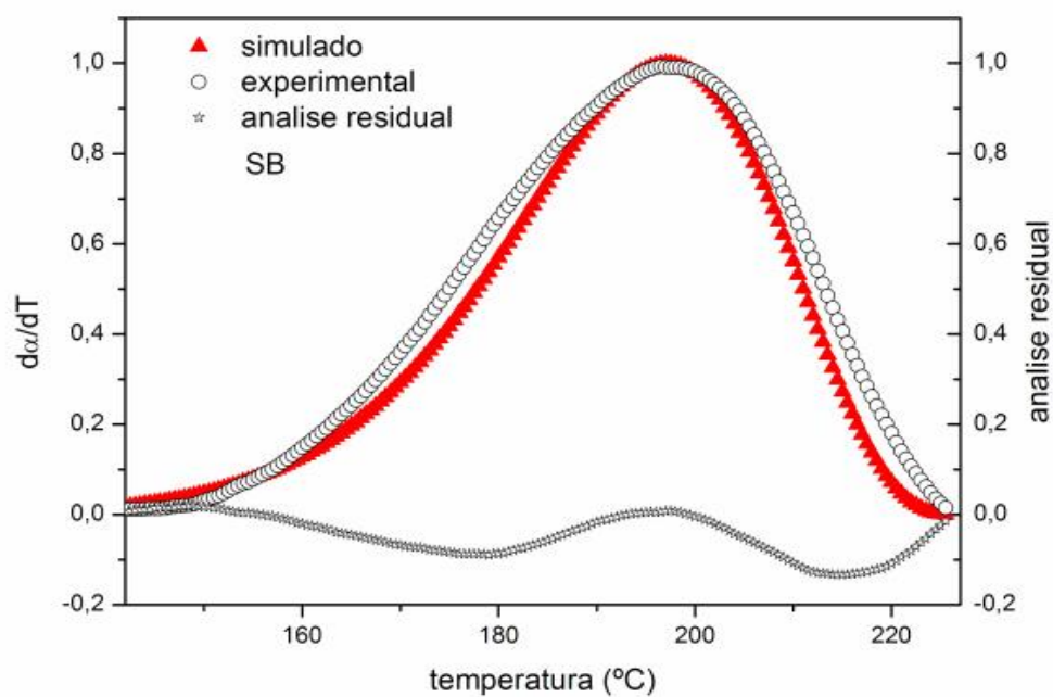
Figura 138: Curvas DTG simulada, experimental e analise residual para a decomposição do 2-MeO-BP'H + para massa de 1mg.
