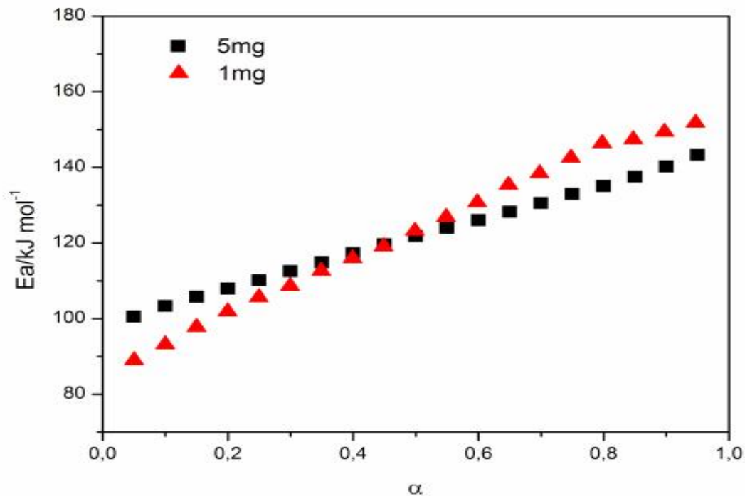
Figura 66: Variação da energia de ativação ( E_a/\text{kJ mol}^{-1} ) vs grau de conversão ( \alpha ) da desidratação do \text{Co(2-MeO-BP)}_2 \cdot 2\text{H}_2\text{O} para as massa de 1 e 5mg.
