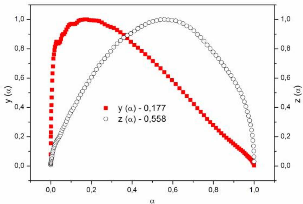
Figura 119: Funções y(\alpha) e z(\alpha) normalizadas para a obtenção de modelos cinéticos da curva TG (10°C/min) para a decomposição do \text{Co(2-MeO-BP)}_2 para a massa de 5mg.
