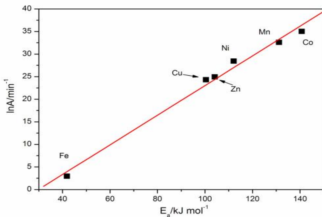
Figura 91: Dependência linear do fator pré-exponencial ( \ln A/\text{min}^{-1} ) vs energia de ativação ( E_a/\text{kJ mol}^{-1} ) para a desidratação dos compostos em alto grau de conversão ( 0,05 > \alpha < 1 ) para a massa de 1mg.
