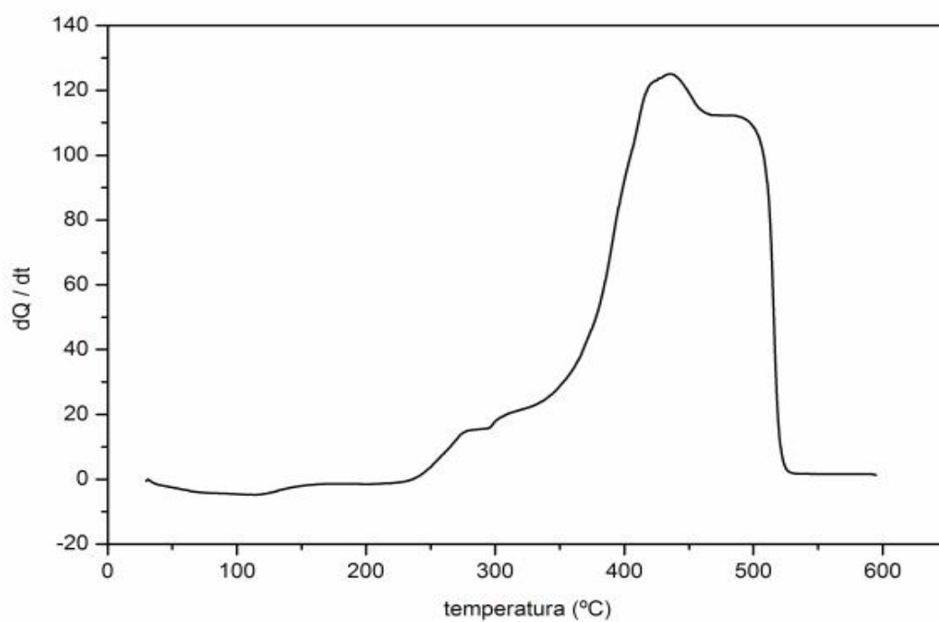
Figura 70: Curva DSC do \text{Ni}(2\text{-MeO-BP}) 2\text{H}_2\text{O} em atmosfera de ar sintético, razão de aquecimento de 20^\circ\text{C}/\text{min} em cadinho de alumínio com tampa perfurada e massa de 3,70 mg.
