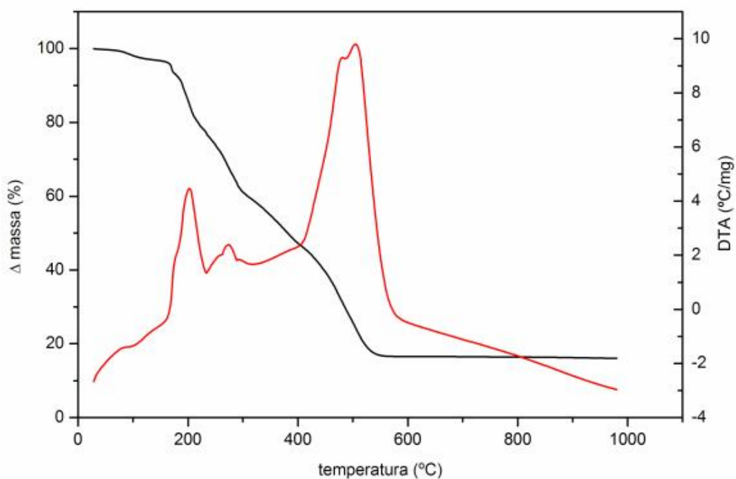
Figura 75: Curvas TG-DTA do \text{Cu(2-MeO-BP)}_2 \cdot \text{H}_2\text{O} em atmosfera de ar sintético, razão de aquecimento de 20^\circ\text{C}/\text{min} em cadinho de \alpha\text{-Al}_2\text{O}_3 e massa de 7,060 mg.
