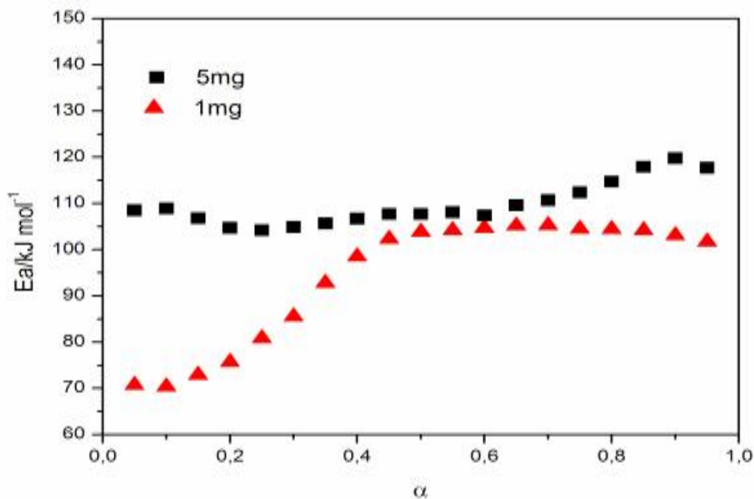
Figura 84: Variação da energia de ativação ( E_a/\text{kJ mol}^{-1} ) vs grau de conversão ( \alpha ) da desidratação do \text{Zn(2-MeO-BP)}_2 \cdot 1,5\text{H}_2\text{O} para as massa de 1 e 5mg.
