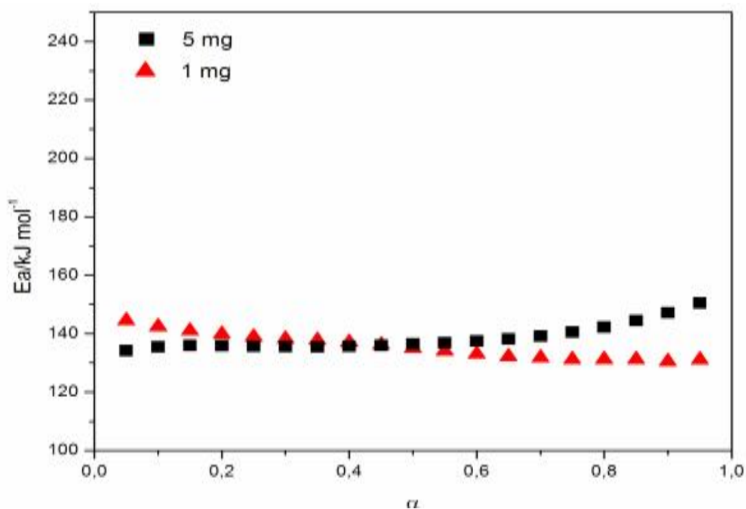
Figura 49: Variação da energia de ativação ( E_a/\text{kJ mol}^{-1} ) vs grau de conversão ( \alpha ) da decomposição do 2-MeO-BPNa + para as massa de 1 e 5mg.
