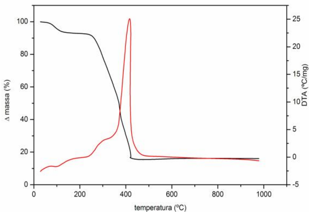
Figura 69: Curvas TG-DTA do \text{Ni(2-MeO-BP)}_2 \cdot 2\text{H}_2\text{O} em atmosfera de ar sintético, razão de aquecimento de 20^{\circ}\text{C/min} em cadinho de \alpha\text{-Al}_2\text{O}_3 e massa de 6,926 mg.
