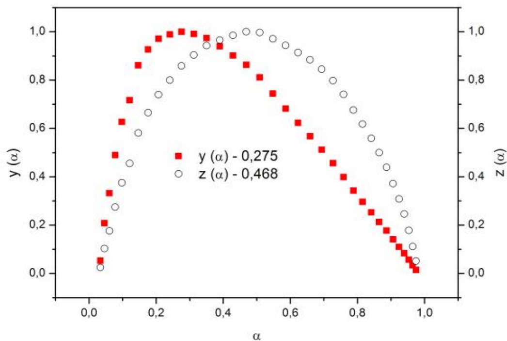
Figura 125: Funções y(\alpha) e z(\alpha) normalizadas para a obtenção de modelos cinéticos da curva TG ( 10^\circ\text{C/min} ) para a decomposição do \text{Zn}(2\text{-MeO-BP})_2 para a massa de 5mg.
