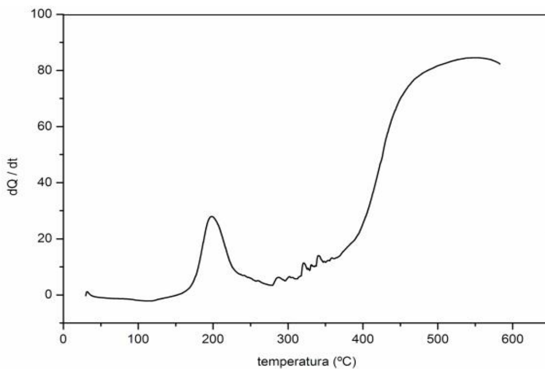
Figura 58: Curva DSC do \text{Fe(2-MeO-BP) H}_2\text{O} em atmosfera de ar sintético, razão de aquecimento de 20^{\circ}\text{C}/\text{min} em cadinho de alumínio com tampa perfurada e massa de 3,810 mg.
