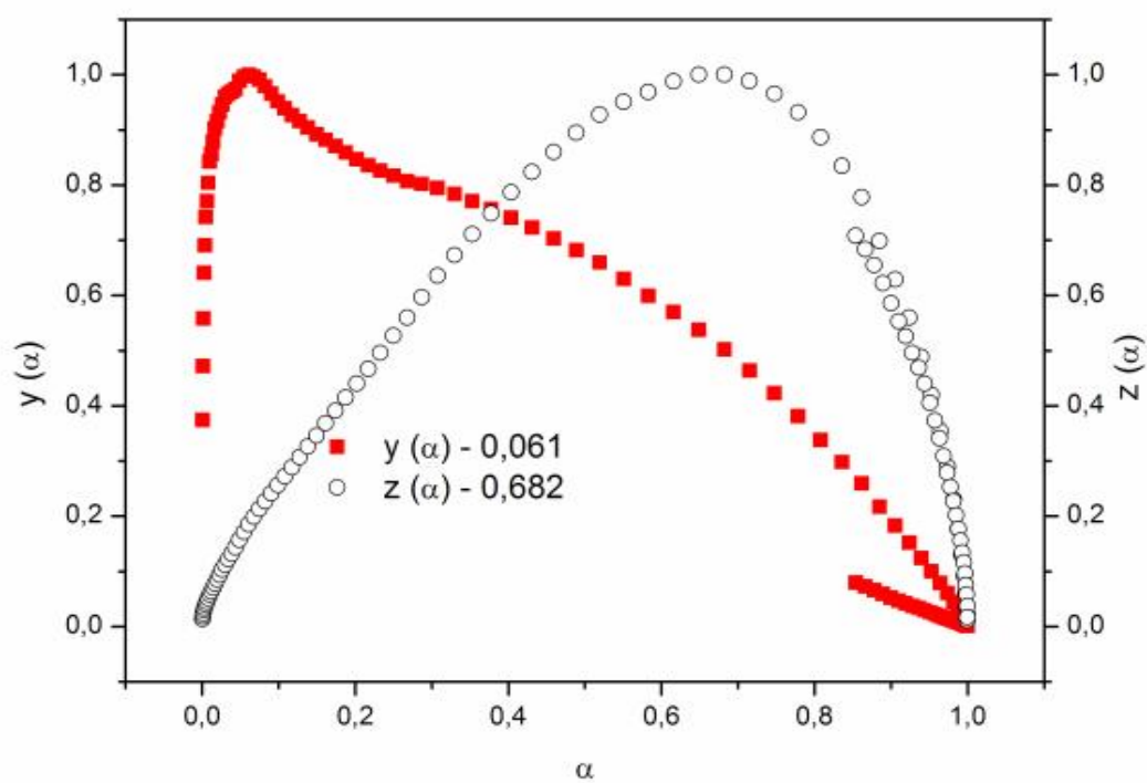
Figura 103: Funções y(\alpha) e z(\alpha) normalizadas para a obtenção de modelos cinéticos da curva TG ( 10^\circ\text{C/min} ) para a desidratação do \text{Co}(2\text{-MeO-BP})_2 \cdot 2\text{H}_2\text{O} para a massa de 5mg.
