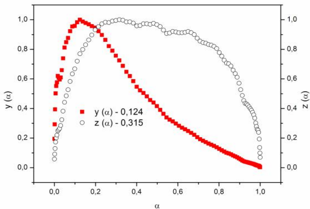
Figura 124: Funções y(\alpha) e z(\alpha) normalizadas para a obtenção de modelos cinéticos da curva TG ( 10^\circ\text{C/min} ) para a decomposição do \text{Zn}(2\text{-MeO-BP})_2 para a massa de 1mg.
