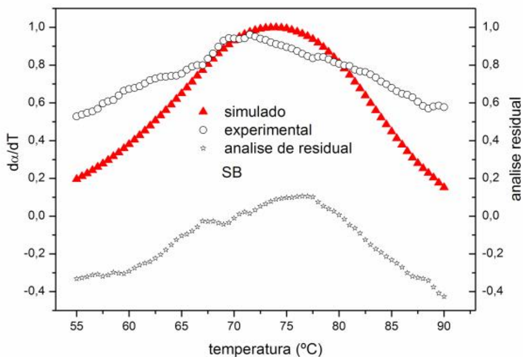
Figura 129: Curvas DTG simulada, experimental e analise residual para a desidratação do \text{Fe(2-MeO-BP)}_2 \cdot \text{H}_2\text{O} para massa de 5mg.
