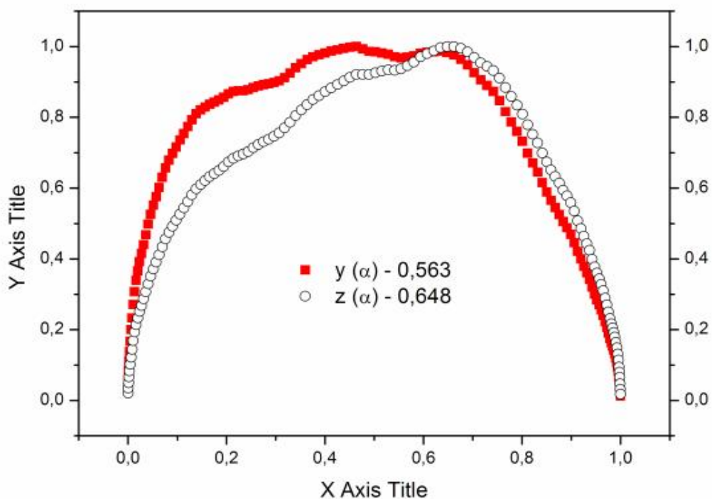
Figura 115: Funções y(\alpha) e z(\alpha) normalizadas para a obtenção de modelos cinéticos da curva TG (10°C/min) para a decomposição do \text{Mn}(2\text{-MeO-BP})_2 para a massa de 5mg.
