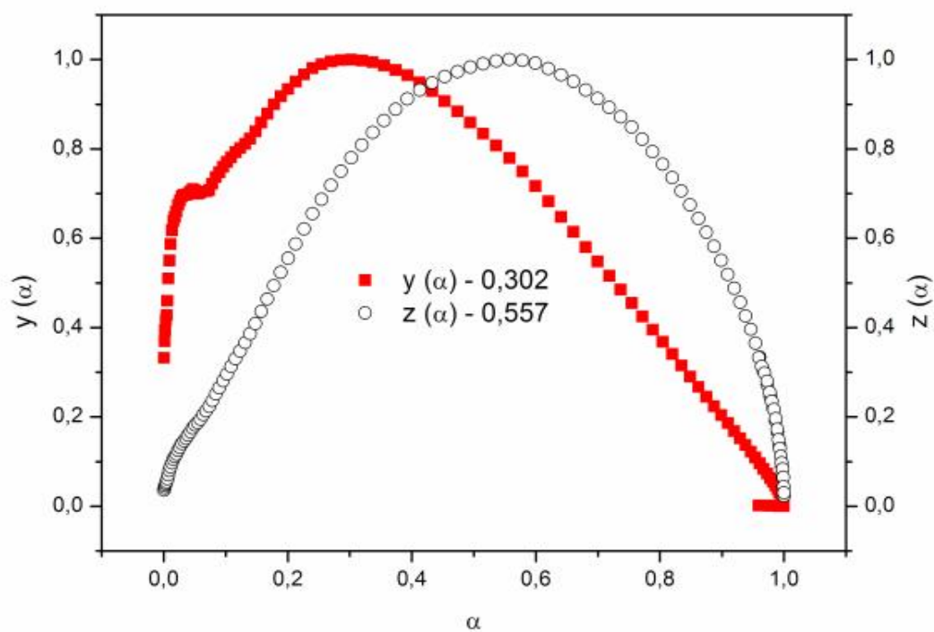
Figura 120: Funções y(\alpha) e z(\alpha) normalizadas para a obtenção de modelos cinéticos da curva TG (10°C/min) para a decomposição do \text{Ni(2-MeO-BP)}_2 para a massa de 1mg.
