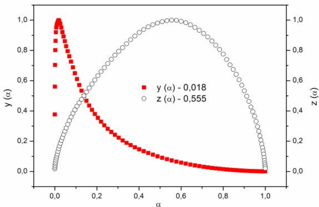
Figura 117: Funções y(\alpha) e z(\alpha) normalizadas para a obtenção de modelos cinéticos da curva TG ( 10^\circ\text{C/min} ) para a decomposição do \text{Fe}(2\text{-MeO-BP})_2 para a massa de 5mg.
