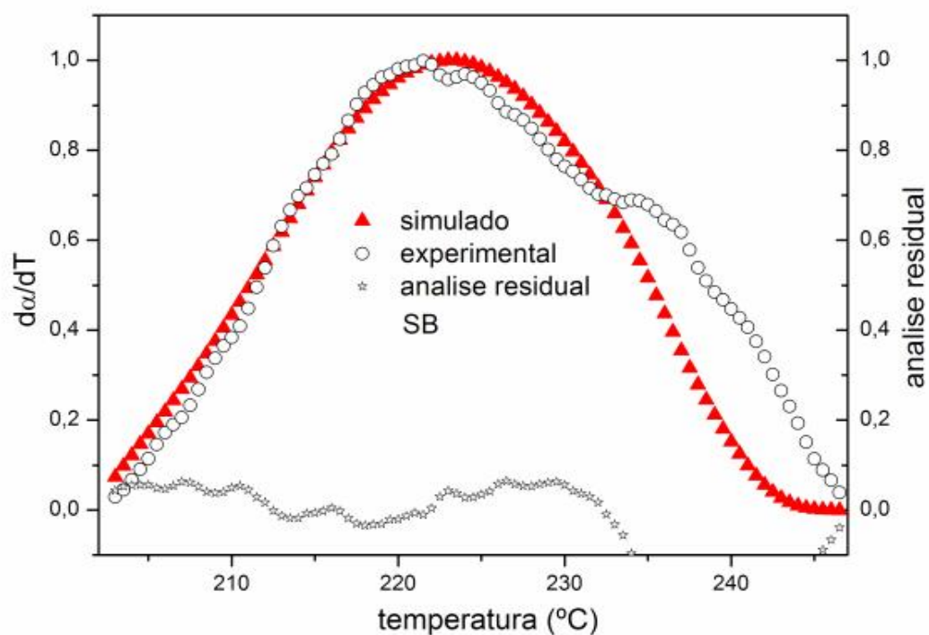
Figura 142: Curvas DTG simulada, experimental e analise residual para a decomposição do \text{Mn}(2\text{-MeO-BP})_2 \cdot \text{H}_2\text{O} para massa de 1mg.
