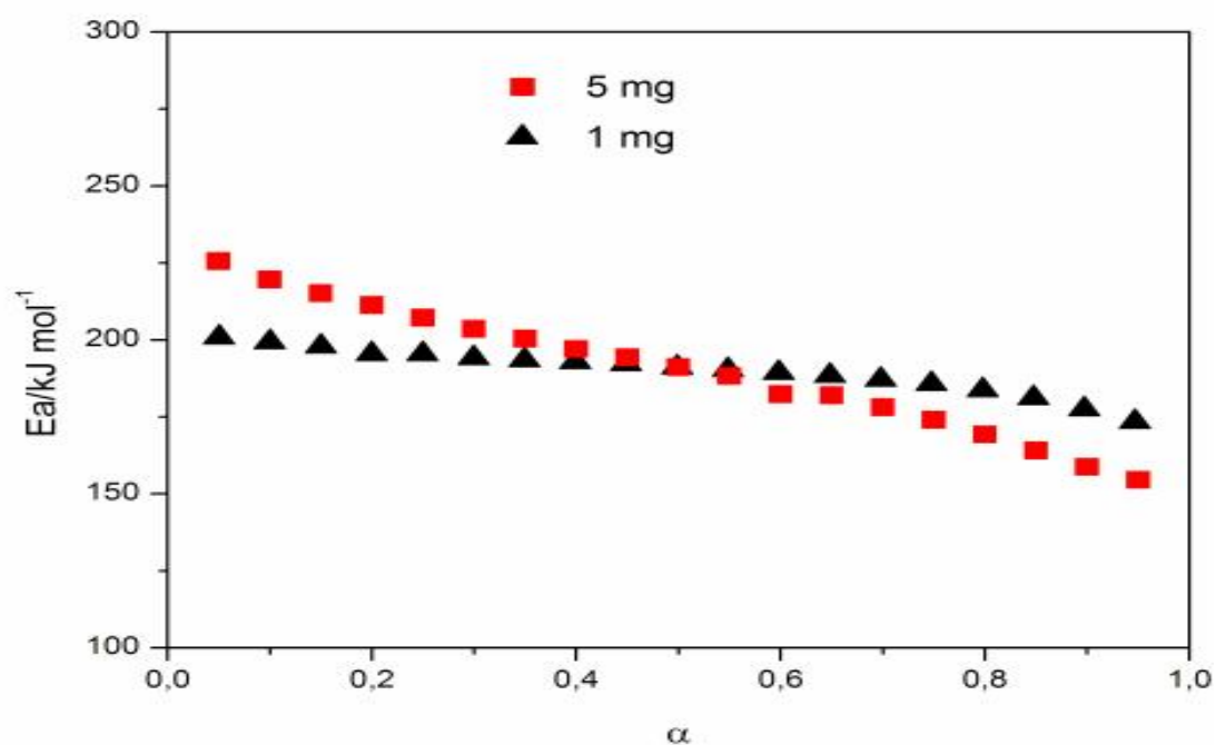
Figura 73: Variação da energia de ativação ( E_a/\text{kJ mol}^{-1} ) vs grau de conversão ( \alpha ) da decomposição do \text{Ni(2-MeO-BP)}_2 para as massa de 1 e 5mg.
