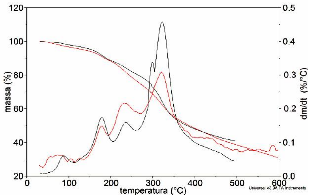
Figura 59: Curvas TG/DTG do \text{Fe(2-MeO-BP)}_2 \cdot 0,65\text{H}_2\text{O} em atmosfera de nitrogênio, razão de aquecimento de 5^\circ\text{C}/\text{min} , massa da amostra em torno de 1mg (vermelho) e 5mg (preto) em cadinho de \alpha\text{-Al}_2\text{O}_3 .
