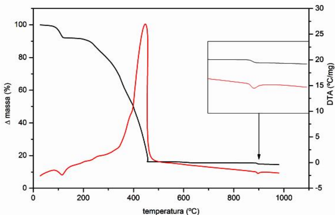
Figura 63: Curvas TG-DTA do \text{Co(2-MeO-BP)}_2 \cdot 2,5\text{H}_2\text{O} em atmosfera de ar sintético, razão de aquecimento de 20^{\circ}\text{C}/\text{min} em cadinho de \alpha\text{-Al}_2\text{O}_3 e massa de 7,115 mg.
