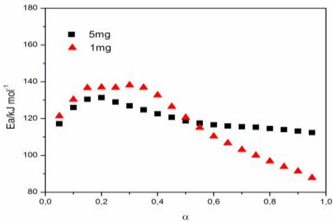
Figura 78: Variação da energia de ativação ( E_a/\text{kJ mol}^{-1} ) vs grau de conversão ( \alpha ) da desidratação do \text{Cu(2-MeO-BP)}_2 \cdot 0,70\text{H}_2\text{O} para as massa de 1 e 5mg.
