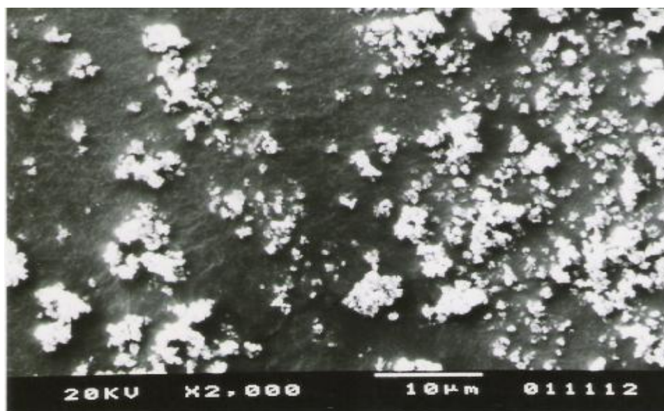
Figura 23: Microscopia eletrônica de varredura (2000X) do \text{Ni}(\text{2-MeO-BP})_2 \cdot 2\text{H}_2\text{O} hidratado.
