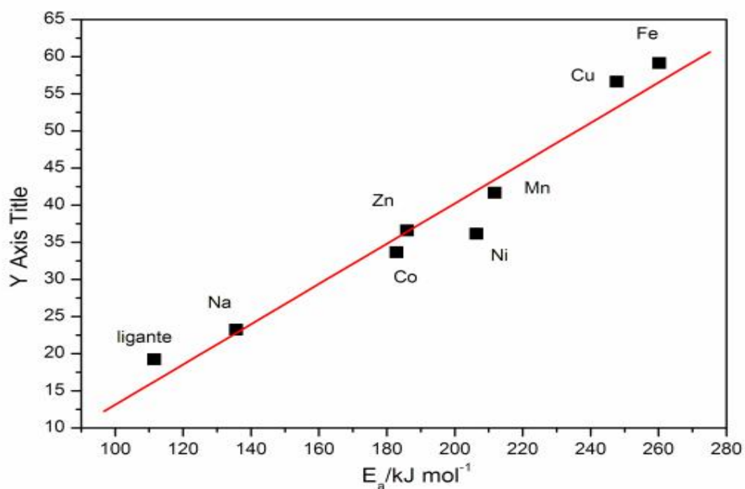
Figura 96: Dependência linear do fator pré-exponencial ( \ln A / \text{min}^{-1} ) vs energia de ativação ( E_a / \text{kJ mol}^{-1} ) para a decomposição dos compostos em baixo grau de conversão ( 0,05 > \alpha < 0,5 ) para a massa de 5mg.
