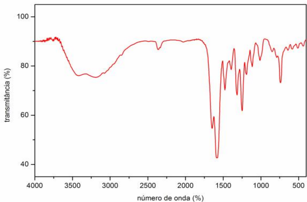
Figura 36: Espectro de absorção na região do infravermelho (FTIR) do \text{Co}(\text{2-MeO-BP})_2 \cdot 2,5\text{H}_2\text{O} .
