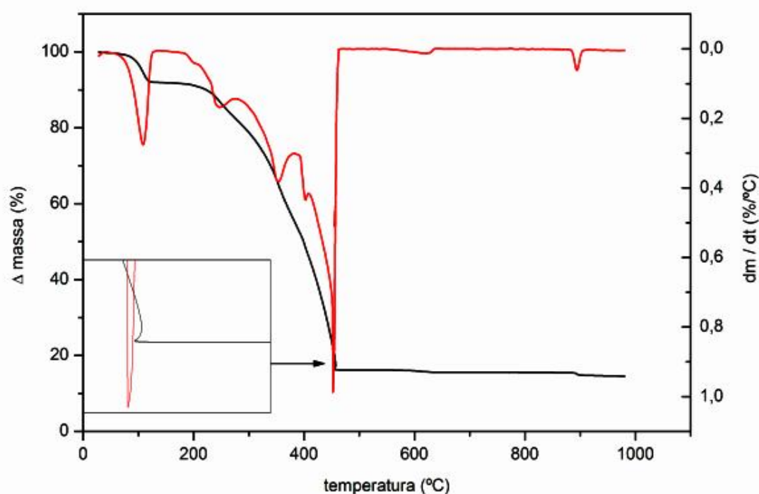
Figura 62: Curvas TG/DTG do \text{Co(2-MeO-BP)}_2 \cdot 2,5\text{H}_2\text{O} em atmosfera de ar sintético, razão de aquecimento de 20^{\circ}\text{C}/\text{min} em cadinho de \alpha\text{-Al}_2\text{O}_3 e massa de 7,115 mg.
