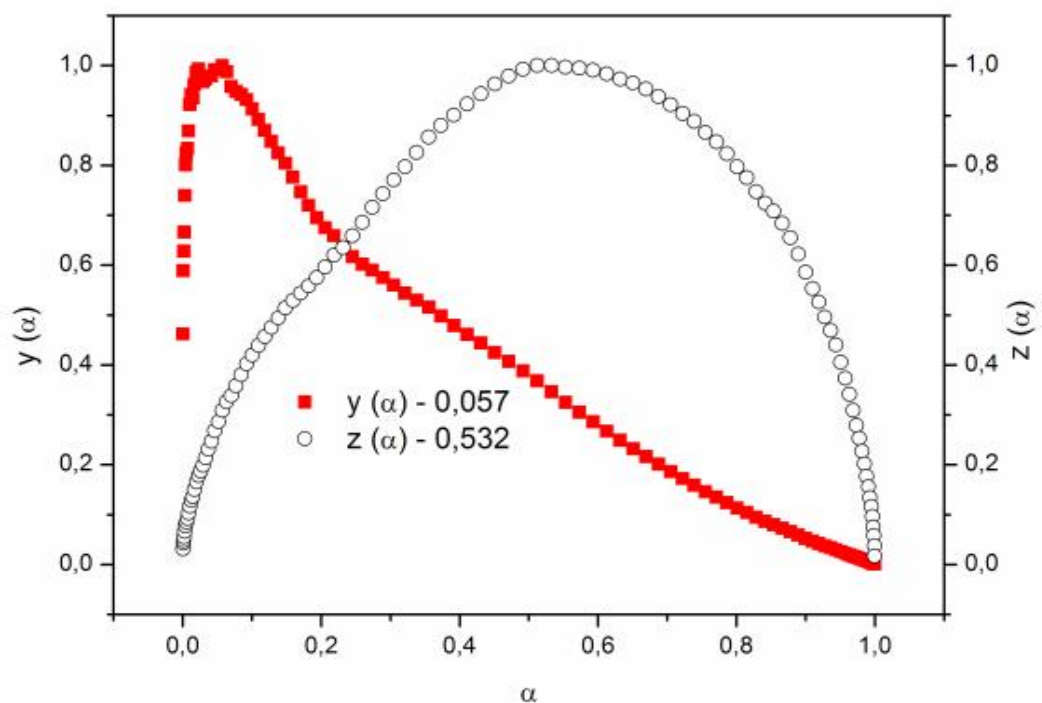
Figura 109: Funções y(\alpha) e z(\alpha) normalizadas para a obtenção de modelos cinéticos da curva TG ( 10^\circ\text{C/min} ) para a desidratação do \text{Zn}(2\text{-MeO-BP})_2 \cdot \text{H}_2\text{O} para a massa de 5mg.
