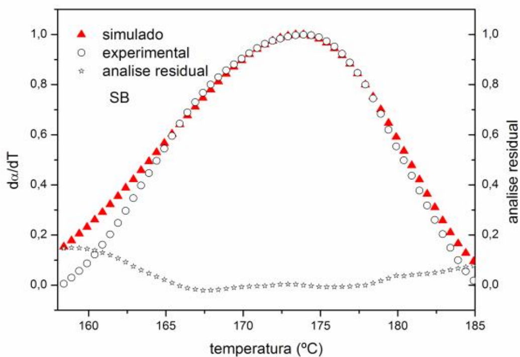
Figura 151: Curvas DTG simulada, experimental e análise residual para a decomposição do \text{Cu}(2\text{-MeO-BP})_2 \text{H}_2\text{O} para massa de 5mg.
