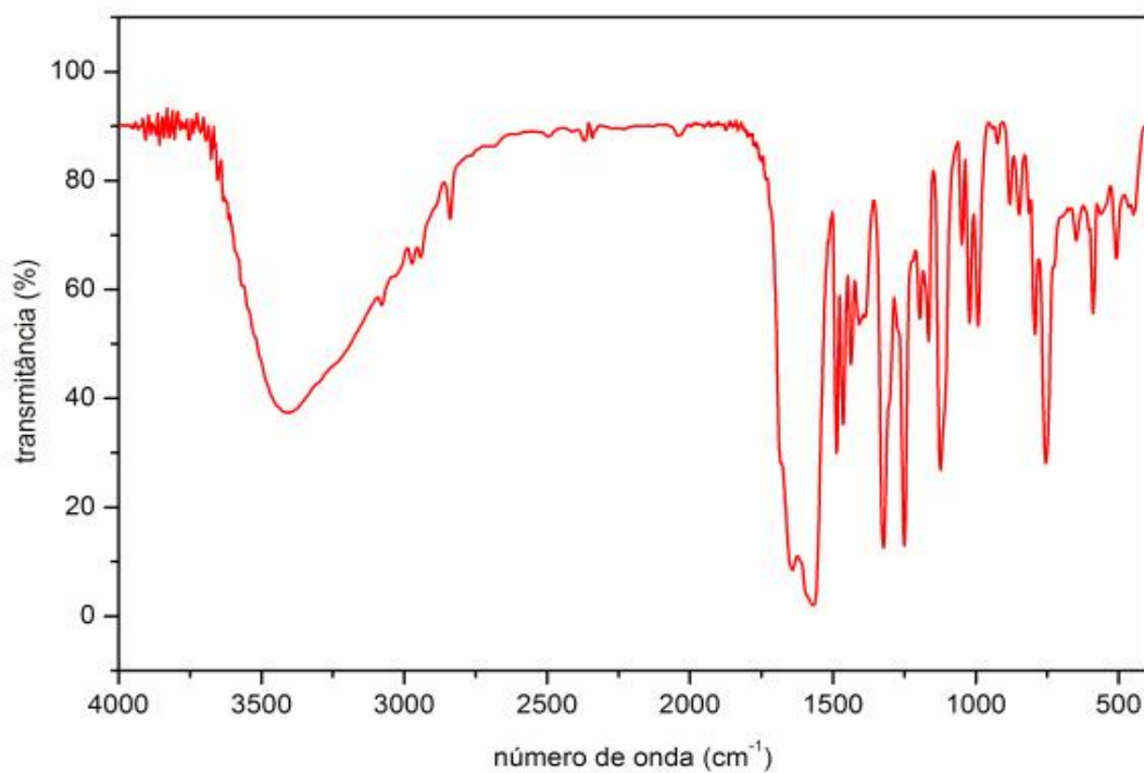
Figura 34: Espectro de absorção na região do infravermelho (FTIR) do Mn(2-MeO-BP) 2 1,5H 2 O.
