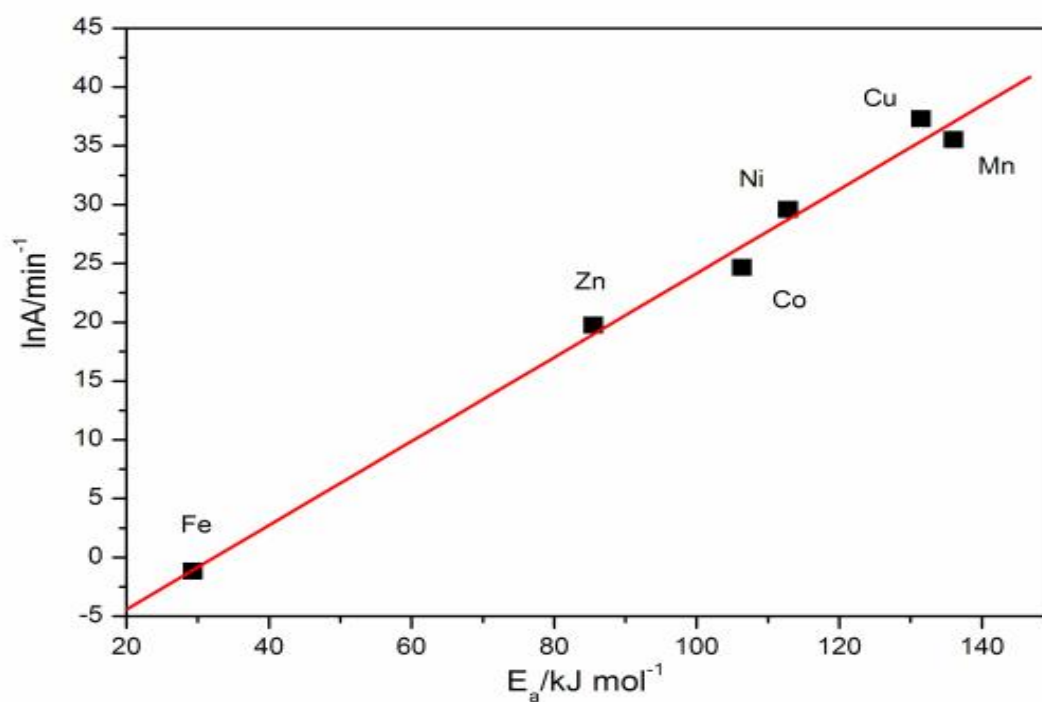
Figura 90: Dependência linear do fator pré-exponencial ( \ln A/\text{min}^{-1} ) vs energia de ativação ( E_a/\text{kJ mol}^{-1} ) para a desidratação dos compostos em baixo grau de conversão ( 0,05 > \alpha < 0,5 ) para a massa de 1mg.
