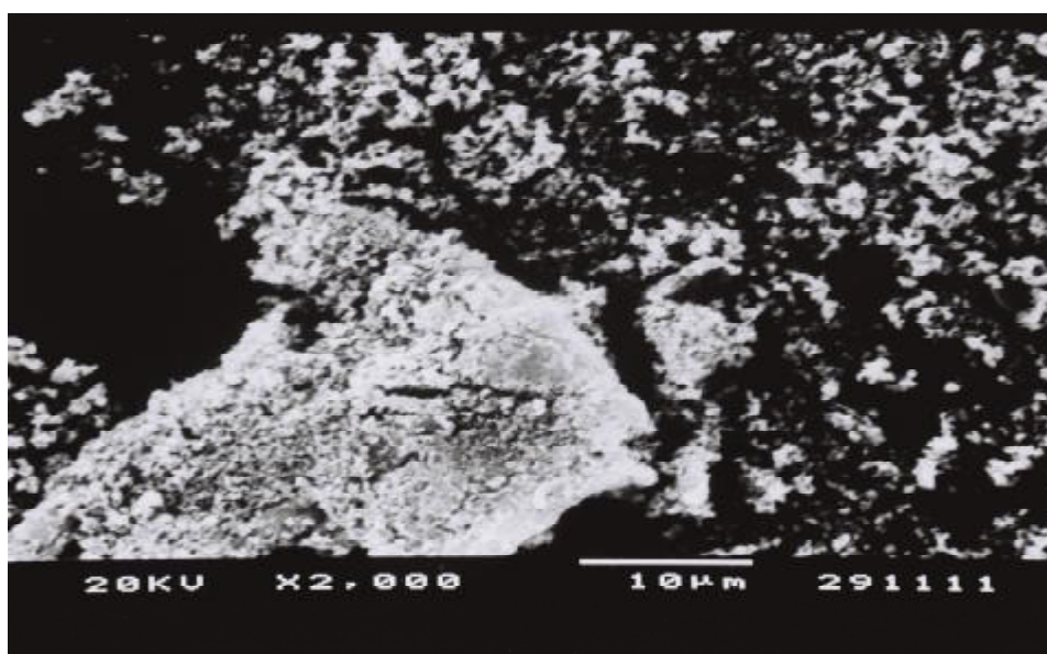
Figura 24: Microscopia eletrônica de varredura (2000X) do \text{Ni}(\text{2-MeO-BP})_2 anidro.
