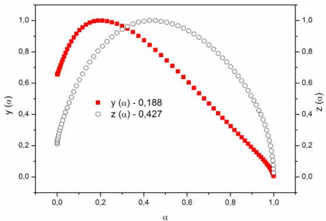
Figura 121: Funções y(\alpha) e z(\alpha) normalizadas para a obtenção de modelos cinéticos da curva TG (10°C/min) para a decomposição do \text{Ni(2-MeO-BP)}_2 para a massa de 5mg.
