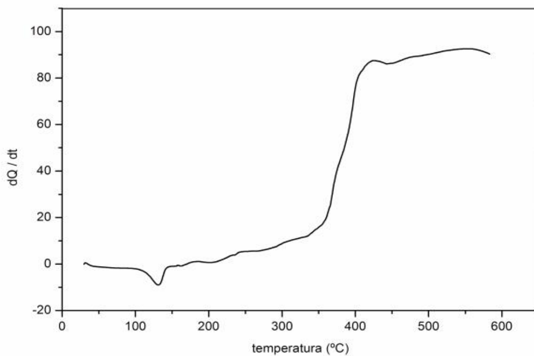
Figura 52: Curva DSC do Mn(2-MeO-BP) 1,5H_2O em atmosfera de ar sintético, razão de aquecimento de 20^{\circ}C/min em cadinho de alumínio com tampa perfurada e massa de 3,581 mg.
