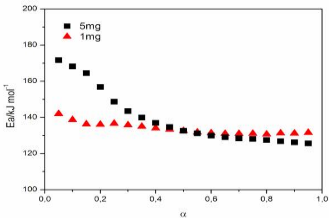
Figura 54: Variação da energia de ativação ( E_a/\text{kJ mol}^{-1} ) vs grau de conversão ( \alpha ) da desidratação do \text{Mn(2-MeO-BP)}_2 \cdot 1,5\text{H}_2\text{O} para as massa de 1 e 5mg.
