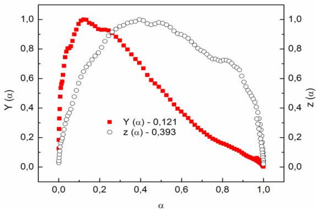
Figura 114: Funções y(\alpha) e z(\alpha) normalizadas para a obtenção de modelos cinéticos da curva TG (10°C/min) para a decomposição do \text{Mn}(2\text{-MeO-BP})_2 para a massa de 1mg
