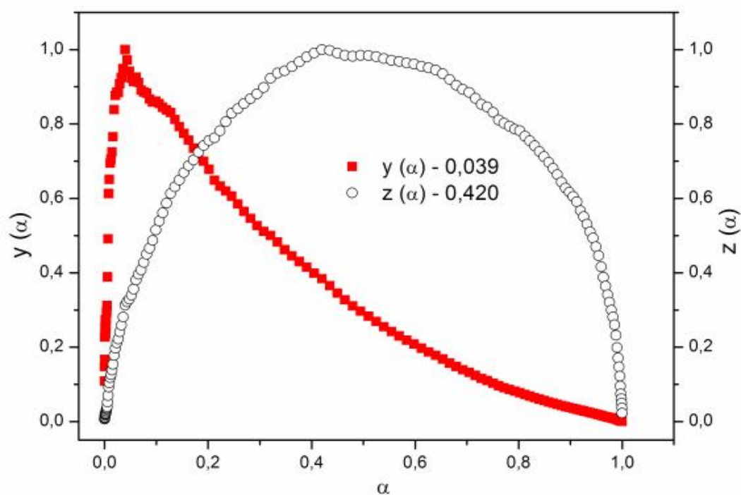
Figura 100: Funções y(\alpha) e z(\alpha) normalizadas para a obtenção de modelos cinéticos da curva TG ( 10^\circ\text{C/min} ) para a desidratação do \text{Fe}(2\text{-MeO-BP})_2 \cdot 0,5\text{H}_2\text{O} para a massa de 1mg.
