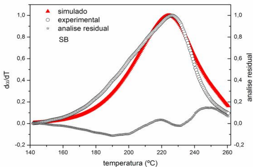
Figura 139: Curvas DTG simulada, experimental e analise residual para a decomposição do 2-MeO-BP'H + para massa de 5mg
