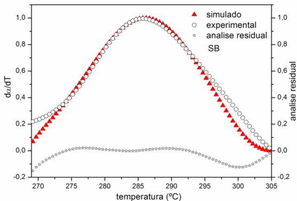
Figura 149: Curvas DTG simulada, experimental e analise residual para a decomposição do \text{Ni(2-MeO-BP)}_2 \cdot 2\text{H}_2\text{O} para massa de 5mg.
