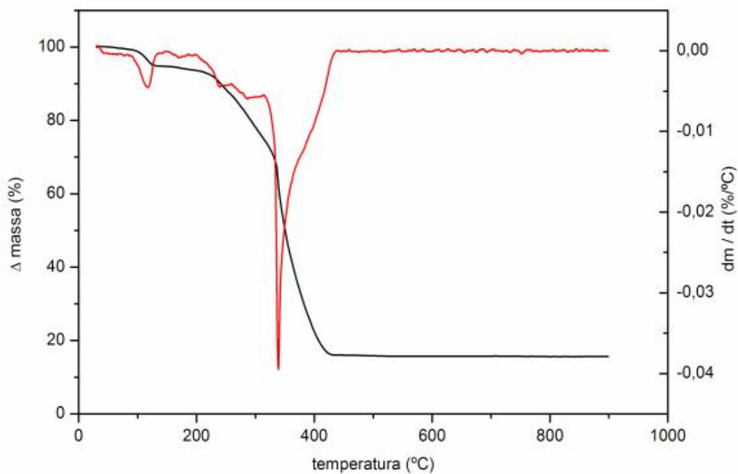
Figura 50: Curvas TG/DTG do \text{Mn}(2\text{-MeO-BP})_2 \cdot 1,5\text{H}_2\text{O} em atmosfera de ar sintético, razão de aquecimento de 20^{\circ}\text{C}/\text{min} em cadinho de \alpha\text{-Al}_2\text{O}_3 e massa de 7,410mg.
