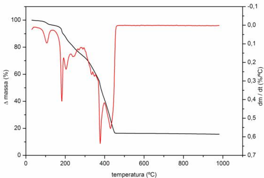
Figura 56: Curvas TG/DTG do \text{Fe(2-MeO-BP)}_2 \cdot \text{H}_2\text{O} em atmosfera de ar sintético, razão de aquecimento de 20^\circ\text{C}/\text{min} em cadinho de \alpha\text{-Al}_2\text{O}_3 e massa de 7,092 mg.
