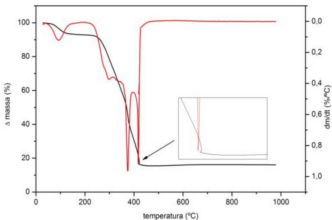
Figura 68: Curvas TG/DTG do \text{Ni(2-MeO-BP)}_2 \cdot 2\text{H}_2\text{O} em atmosfera de ar sintético, razão de aquecimento de 20^{\circ}\text{C/min} em cadinho de \alpha\text{-Al}_2\text{O}_3 e massa de 6,926 mg.
