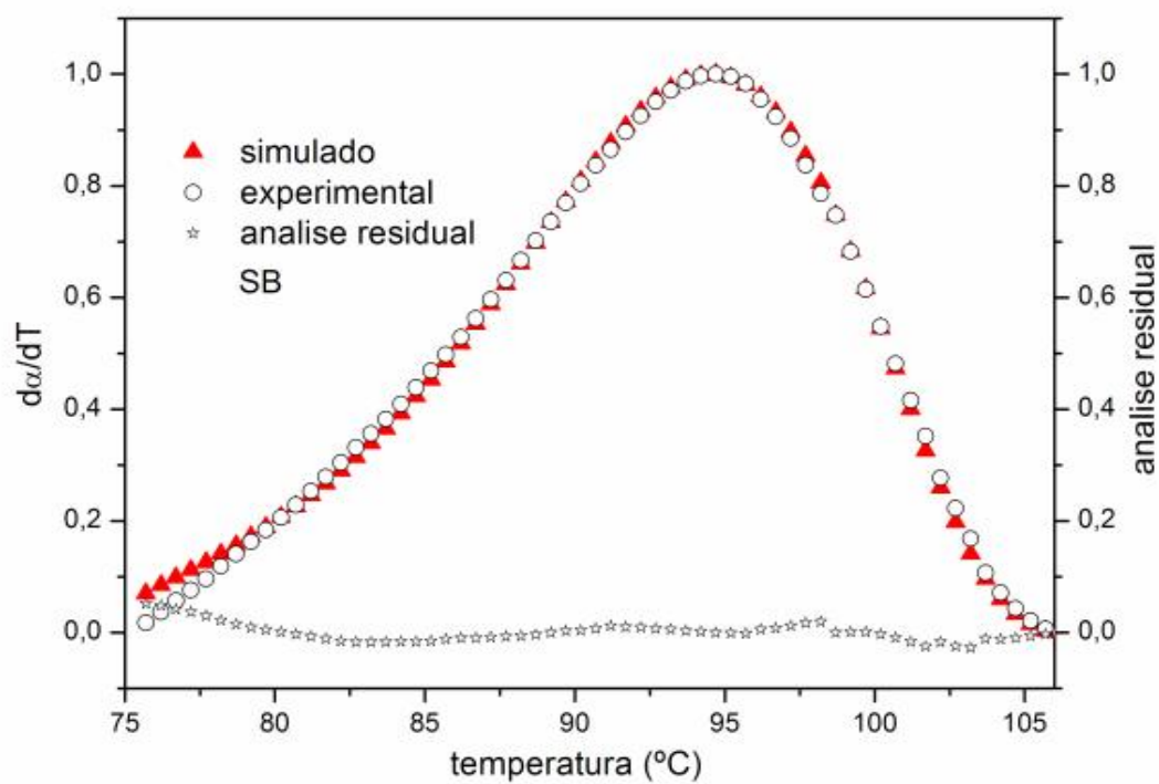
Figura 137: Curvas DTG simulada, experimental e analise residual para a desidratação do \text{Zn(2-MeO-BP)}_2 \text{H}_2\text{O} para massa de 5mg.
