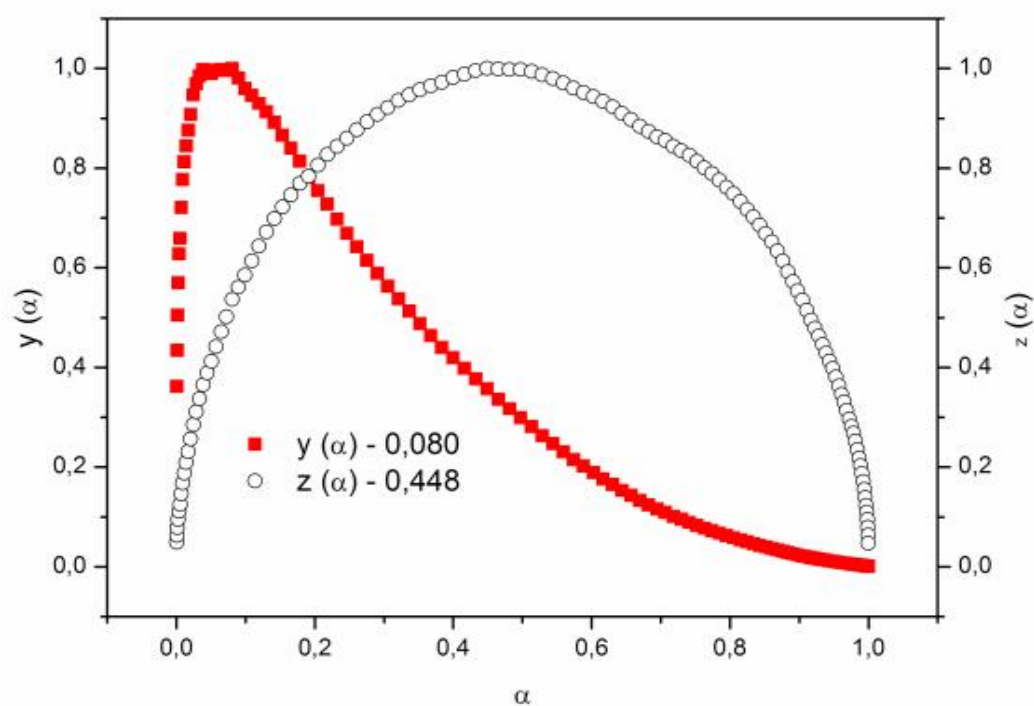
Figura 105: Funções y(\alpha) e z(\alpha) normalizadas para a obtenção de modelos cinéticos da curva TG ( 10^\circ\text{C/min} ) para a desidratação do \text{Ni(2-MeO-BP)}_2 \cdot 2\text{H}_2\text{O} para a massa de 5mg.
