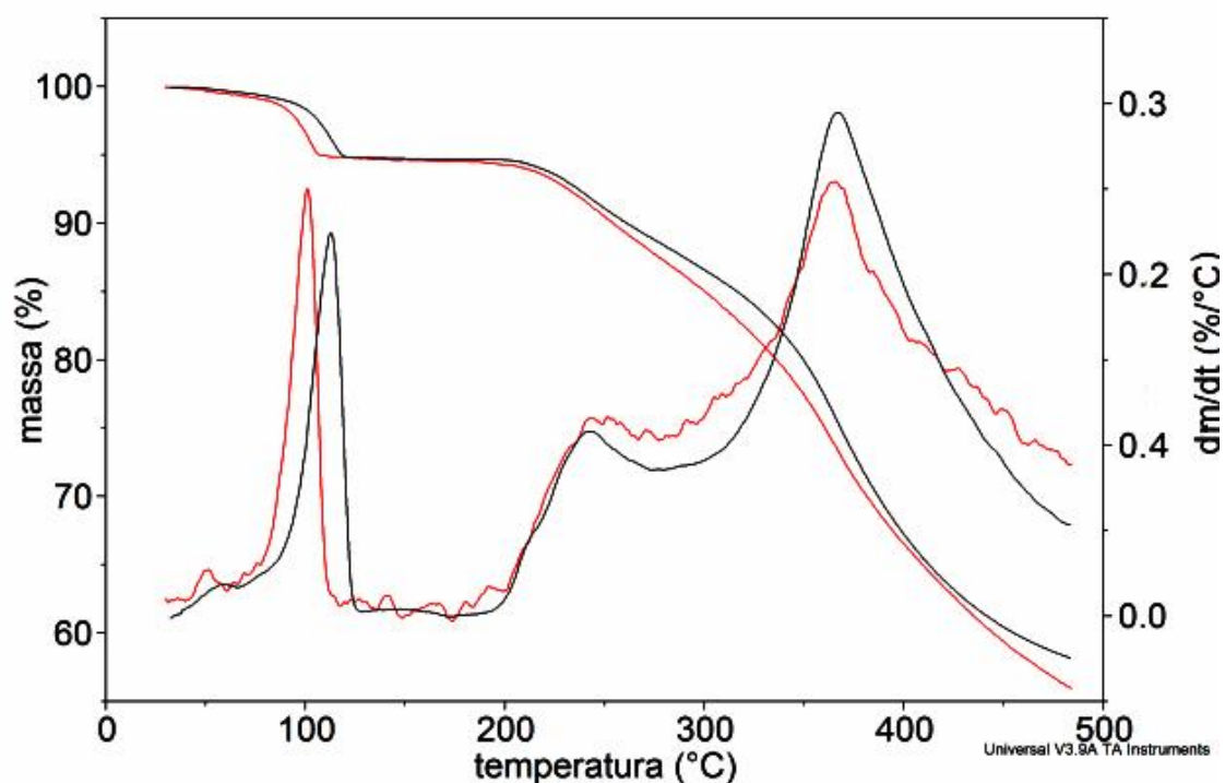
Figura 53: Curvas TG/DTG do \text{Mn(2-MeO-BP)}_2 \cdot 1,5\text{H}_2\text{O} em atmosfera de nitrogênio, razão de aquecimento de 10^\circ\text{C min}^{-1} , massa da amostra em torno de 1mg (vermelho) e 5mg (preto) em cadinho de \alpha\text{-Al}_2\text{O}_3 .
