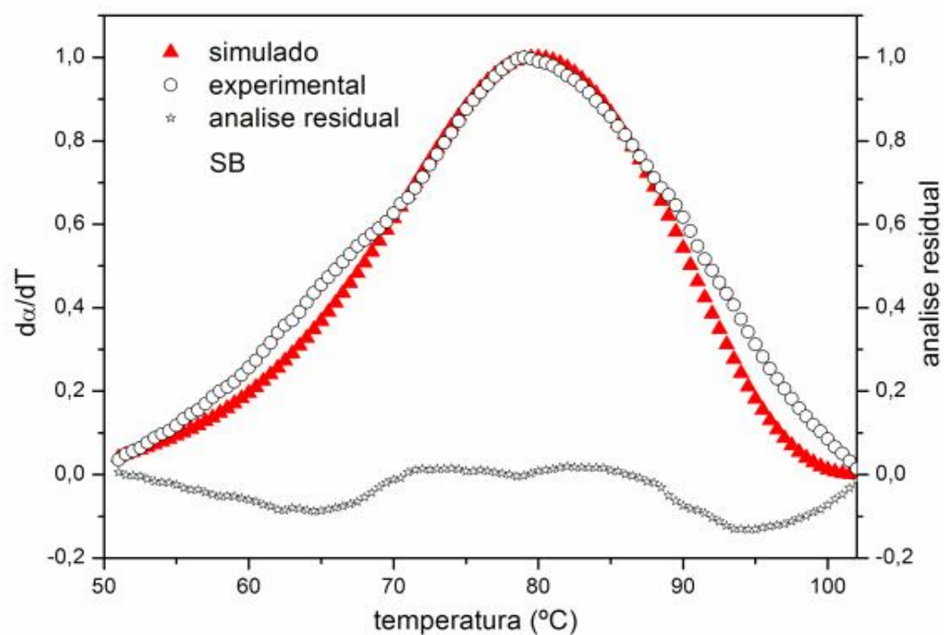
Figura 135: Curvas DTG simulada, experimental e analise residual para a desidratação do \text{Cu(2-MeO-BP)}_2 \cdot \text{H}_2\text{O} para massa de 5mg
