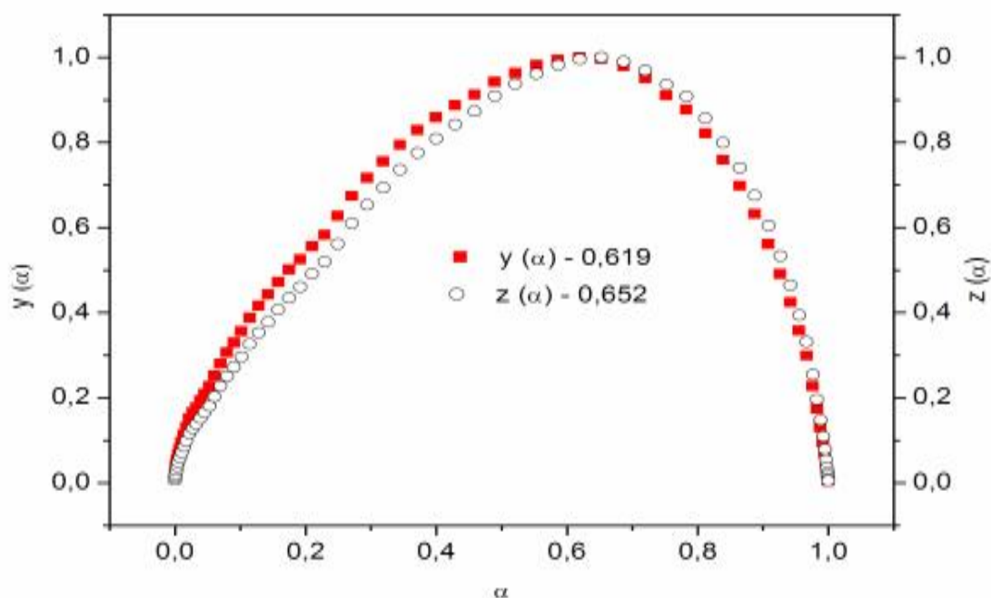
Figura 102: Funções y(\alpha) e z(\alpha) normalizadas para a obtenção de modelos cinéticos da curva TG ( 10^\circ\text{C/min} ) para a desidratação do \text{Co}(2\text{-MeO-BP})_2 \cdot 2\text{H}_2\text{O} para a massa de 1mg.
