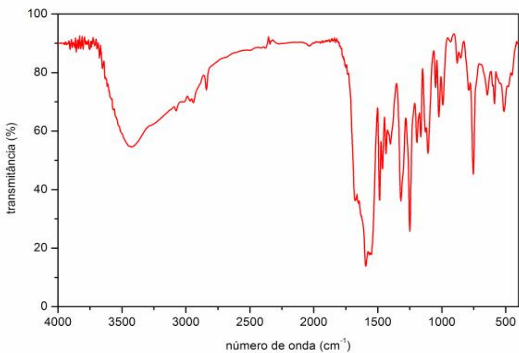
Figura 35: Espectro de absorção na região do infravermelho (FTIR) do Fe(2-MeO-BP) 2 H 2 O.
