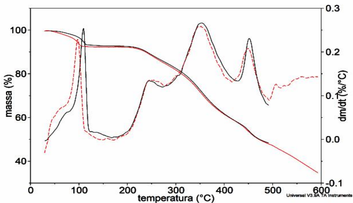
Figura 65: Curvas TG/DTG do \text{Co(2-MeO-BP)}_2 \cdot 2\text{H}_2\text{O} em atmosfera de nitrogênio, razão de aquecimento de 10^\circ\text{C/min} , massa da amostra em torno de 1mg (vermelho) e 5mg (preto) em cadinho de \alpha\text{-Al}_2\text{O}_3 .
