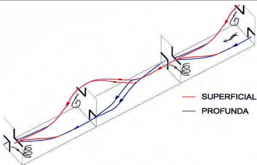
Figura 2 – Desenho esquemático da estrutura padrão das escadas para peixes das usinas do Complexo Canoas, evidenciando a hidrodinâmica (fluxo de água) (MARTINS, 2000).
