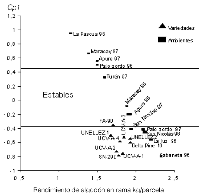
Figura 3. Doble representación Biplot de 9 variedades de algodón en 12 ambientes, según modelo AMMI.
