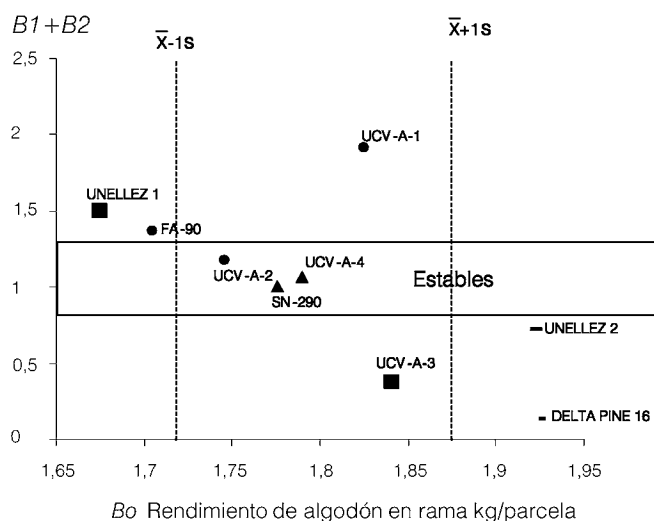
Figura 2. Coeficiente de regresión ( B_1 + B_2 ) y rendimiento de algodón en rama ( B_0 ) de 9 variedades en 12 ambientes, según el método de Cruz et al. (1989).
